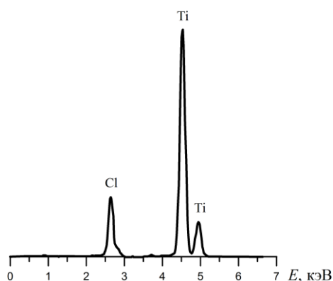
Рис. 4. Рентгенофлуоресцентный спектр
