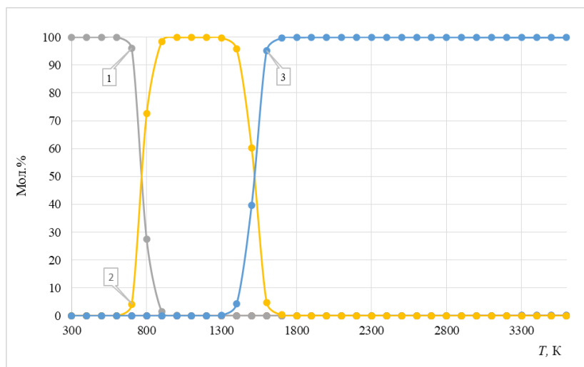
Рис. 1. Распределение цезия по равновесным фазам при нагревании радиоактивного графита в воздухе: 1 — CsCl (к.); 2 — CsCl; 3 — Cs+
