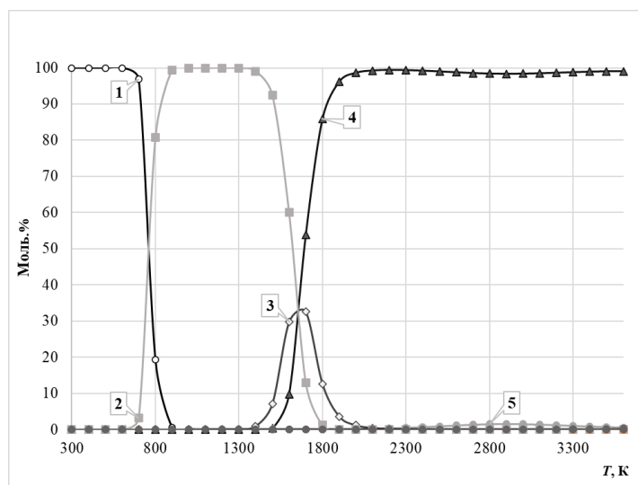
Рис. 1. Распределение никеля по равновесным фазам при нагревании радиоактивного графита в воздухе: 1 – NiCl 2(к.) ; 2 – NiCl 2 ; 3 – NiCl; 4 – Ni; 5 – NiO
