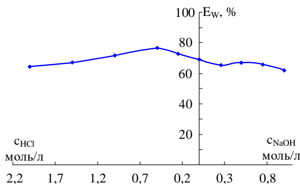
Рис. 1. Зависимость степени извлечения 1 \cdot 10^{-5} M WO_4^{2-} от кислотности в системе АП-ССК- H_2O ( C_{АП} = 0,60 M, C_{ССК} = 0,30 M; C_{HCl} = 1,0 M; C_{NaOH} = 1,0 M)
