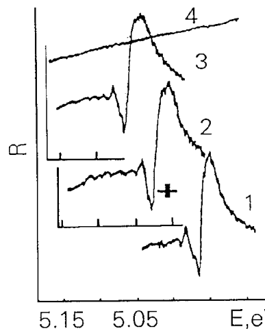
Рис. 4. Спектр зеркального отражения кристаллов LiH (1), \text{LiH}_x\text{D}_{1-x} (2), LiD (3) при 4.2 K, распределение интенсивности света от лампы через установку без кристалла (4)
