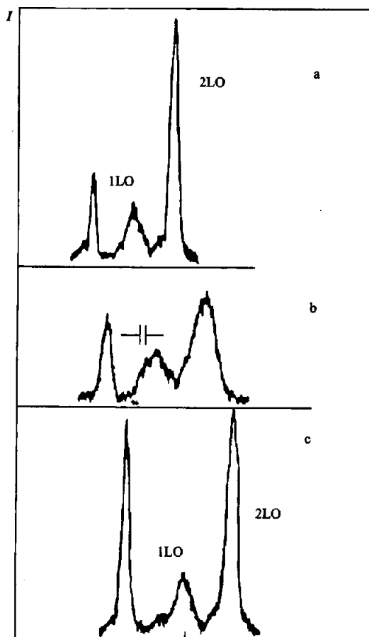
Рис. 5. Спектр люминесценции свободных экситонов в кристаллах, сколотых в сверхтекучем гелии: а – LiH; б – LiHxD1-x; в – LiD при 2 К. Указано разрешение спектрального прибора
