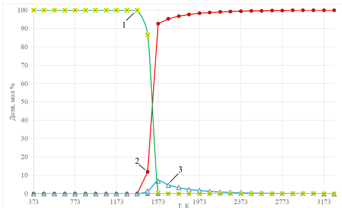
Рис. 1. Распределение марганца по фазам. 1 – \text{MnC}_{2(\text{конд.})} , 2 – \text{Mn}_{(\text{г})} , 3 – \text{MnH}_{(\text{г})}
