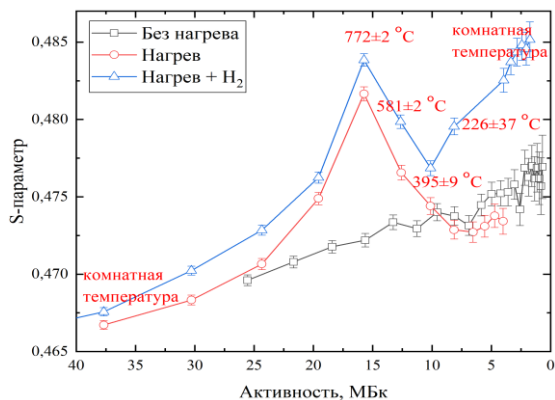
Рисунок 1. Зависимость S- параметра от активности источника 64 Cu для образцов Ti
