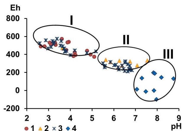
Рисунок 4 – Зависимость Eh-pH для вод, развитых в районах месторождений:
