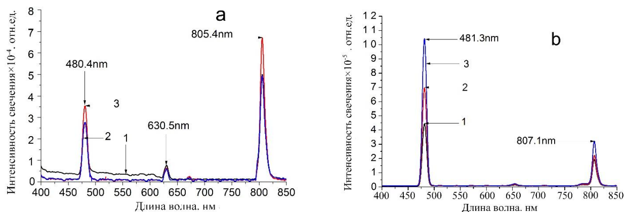
Рисунок 3.2. Спектры люминесценции \text{ZnS-Tm}^{3+} при 303K, после 30 минутного прогрева в вакууме 10^{-6} торр при 573K:
