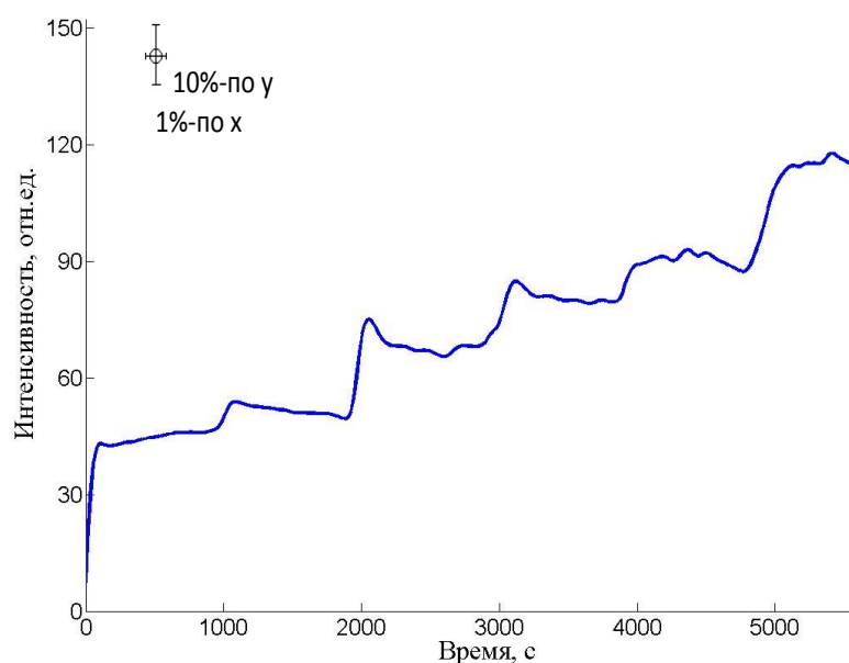
Рисунок 6.6 Приращения интенсивности ГХЛ Н люминофора AlN-Eu 3+ при ступенчатом увеличении плотности потока (концентрации) атомов водорода. Температура 295 К, Давление в трубке 3.0 \cdot 10^{-2} торр, Образец предварительно
