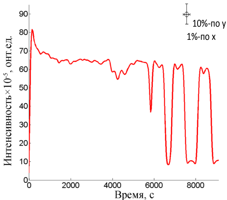
Рисунок 6.4 Интенсивность ГХЛ Н AlN-Eu 3+ при «выключении» и «включении» атомов водорода – «темновые» паузы различной длительности. T=306 К, P H+H 2 =3.0·10 -2 торр.
