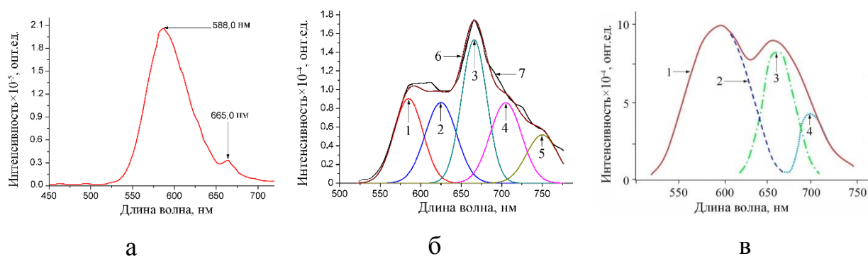
Рисунок 4.1. Спектры свечения микрокристаллического люминофора ZnS-Mn^{2+} (2,5 вес%), 295 К, плотность потока атомов Н в эффузионном пучке 10^{14-16} \text{ см}^{-2} \text{ с}^{-1} ; P_{H+H_2} = 3 \cdot 10^{-2} торр;
