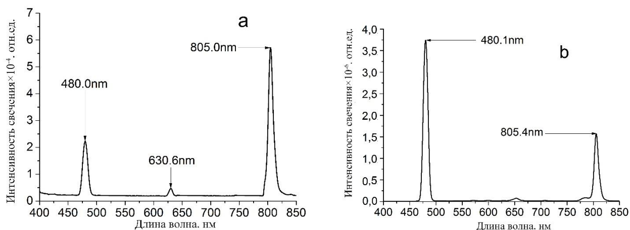
Рисунок 3.4. Спектры люминесценции \text{ZnS-Tm}^{3+} при 303K, после 30 минутного прогрева в \text{H+H}_2 при 573K:
