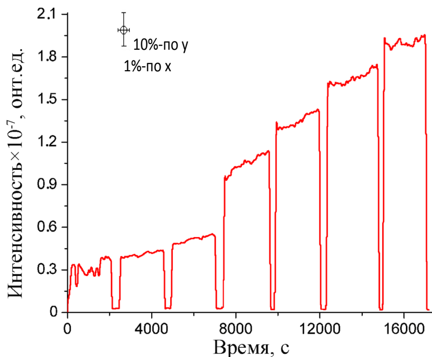
Рисунок. 4.5 Интенсивность ГХЛ Н люминофора \text{ZnS-Mn}^{2+} при «включении» и «выключении» (вспышка-тушение ГХЛ Н ) пучка атомов водорода различной плотности. T = 306\text{K} , P_{\text{H+H}_2} = 3.0 \cdot 10^{-2} торр.
