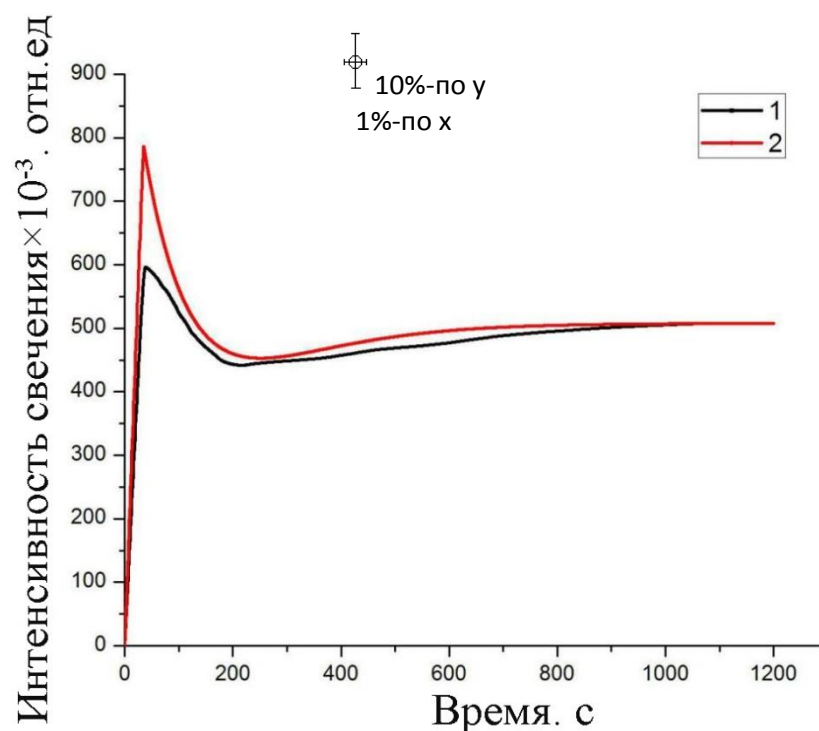
Рисунок 3.7. Вспышка гетерогенной хемилюминесценции при напуске атомов Н
