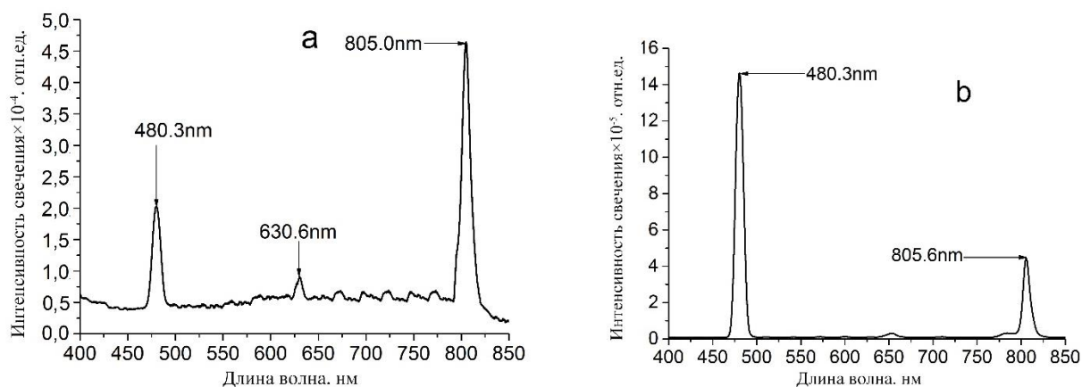
Рисунок 3.3. Спектры люминесценции \text{ZnS-Tm}^{3+} при 303K, после 30 минутного прогрева в \text{H}_2 при 573K:
