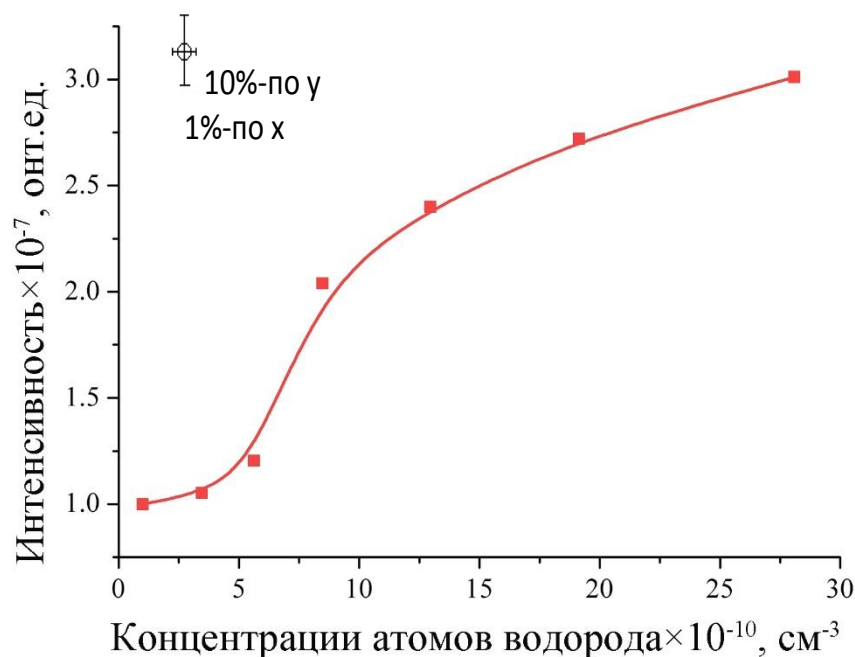
Рисунок 4.7. Стационарная интенсивность ГХЛ н ZnS–Mn 2+ при различных концентрациях атомов водорода. ( 306 K).
