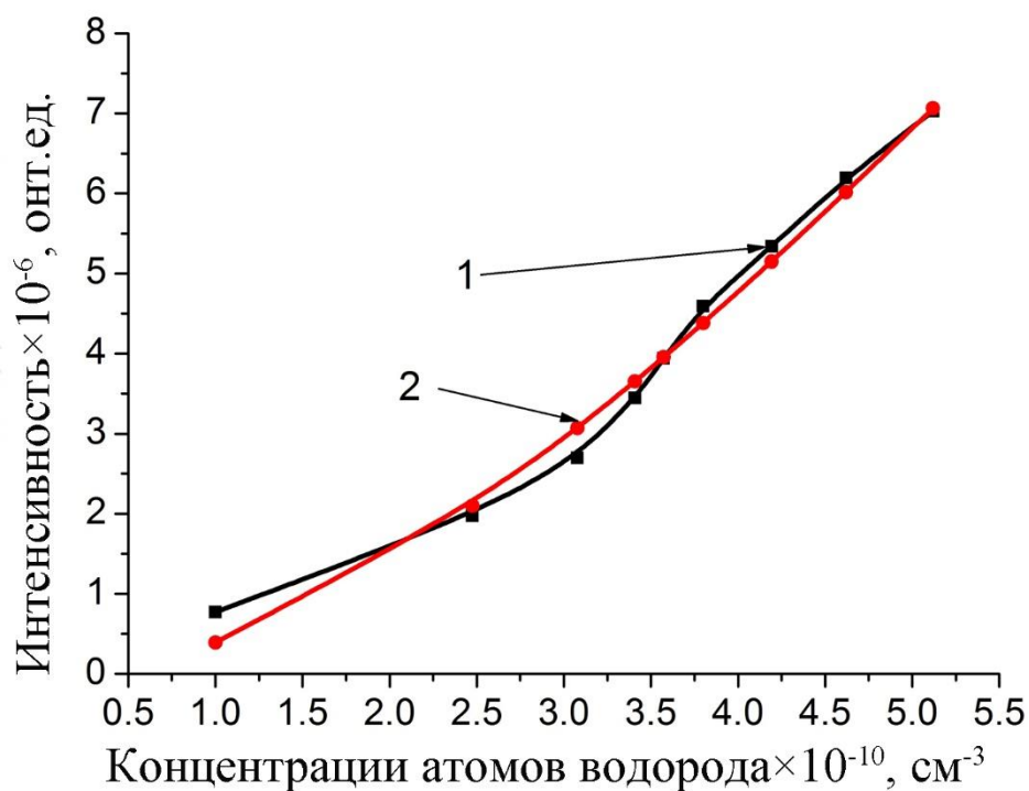
Рисунок 4.6. Зависимость интенсивности ГХЛ II ZnS–Mn 2+ от концентрации атомов водорода, T=295K
