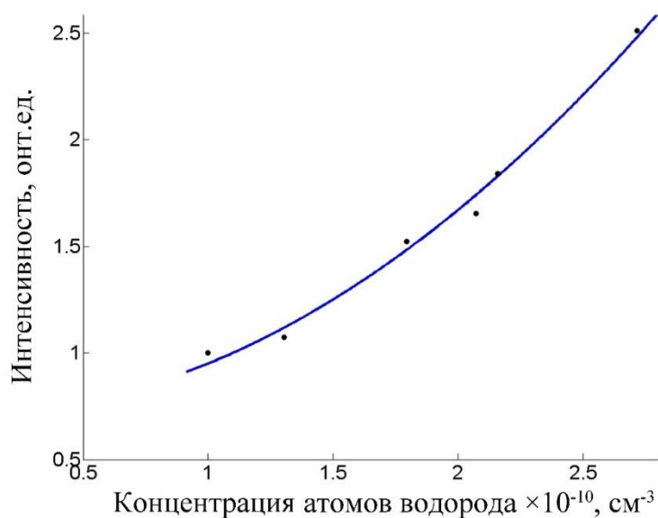
Рисунок 6.7 Зависимость интенсивности ГХЛ H AlN-Eu 3+ от концентрации атомов водорода.
