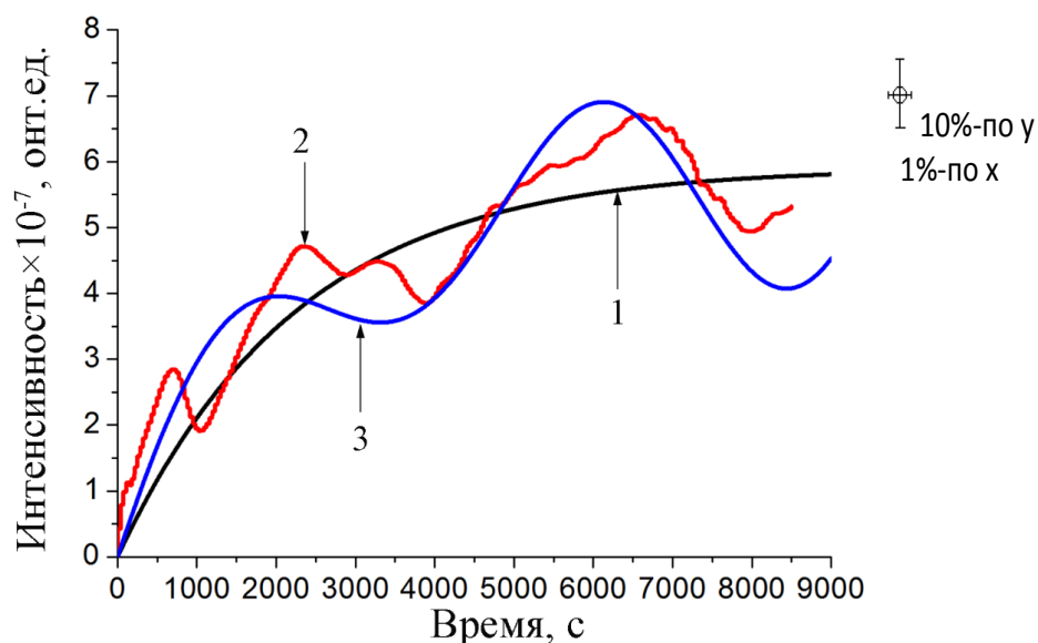
Рисунок 4.3. Разгорание люминесценции \text{ZnS-Mn}^{2+} возбуждаемой атомарным водородом (люминофор \text{ZnS-Mn}^{2+} предварительно прогрет в вакууме 3.0 \cdot 10^{-6} торр). 1- аппроксимация кинетической кривой люминесценции рассчитана по формуле (4.6), 2- эксперимент, 3- аппроксимация кинетической кривой с учетом энергообмена в адсорбционном слое (4.6a). T=295 K.
