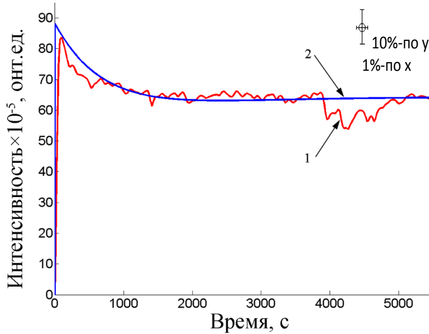
Рисунок 6.3. Кинетическая кривая ГХЛ фосфора \text{AlN-Eu}^{3+} в атомарном водороде. (при концентрациях атомов водорода \sim 10^{10} \text{ см}^{-3} ), T = 295 \text{ K} ; 1-эксперимент; 2- аппроксимирующая зависимость (6.1);
