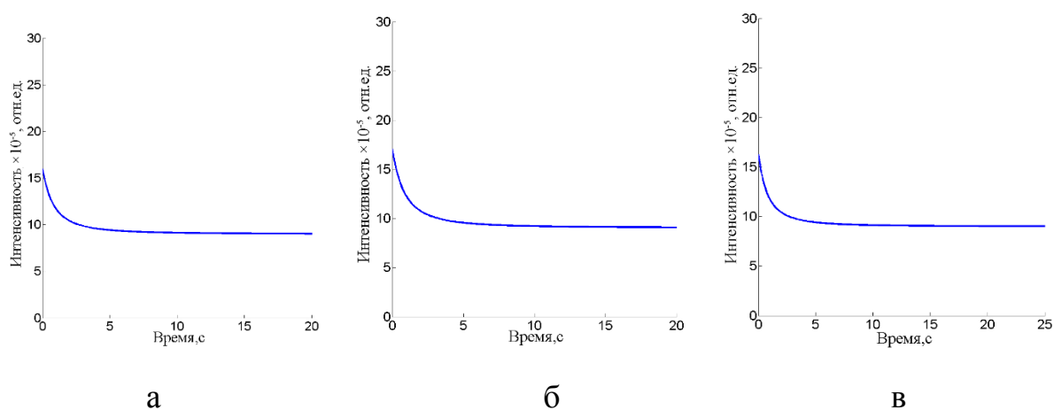
Рисунок 6.5. Начальные участки затухания люминесценции AlN-Eu 3+ при «выключениях» атомов водорода. Длительность предыдущей «темновой» паузы: а- 5, б-10, в-15 мин. Температура образца 306К, давление в разрядной трубке 3.0·10 -2
