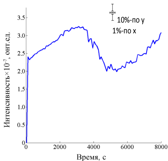
Рисунок 4.4. Зависимость от времени интенсивности свечения ГХЛ фосфора \text{ZnS-Mn}^{2+} возбуждаемой атомами водорода.
