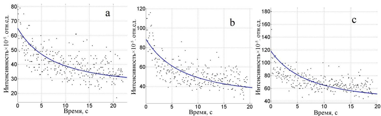
Рисунок 3.9. Начальные участки затухания люминесценции \text{ZnS-Tm}^{3+} после «выключения» атомов водорода после длительных (а-3, b-3,5, c-4 часа) начальных заполнениях поверхности атомами водорода. Температура образца 306K, давление в разрядной трубке 3 \cdot 10^{-2} торр
