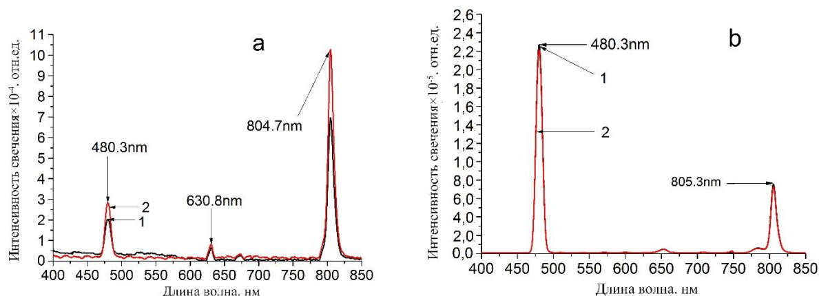
Рисунок 3.5. Спектры люминесценции \text{ZnS-Tm}^{3+} при 303K, после 30 минутного прогрева в вакууме 10^{-6} торр при 573K:
