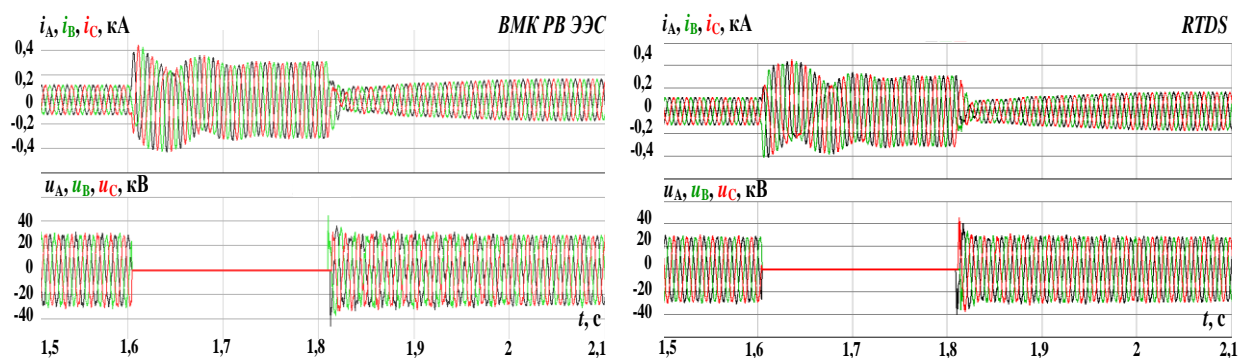
Рисунок 3.27 – Осциллограммы фазных токов и напряжений в узле подключения ВЭУ к ЭЭС при трехфазном КЗ
