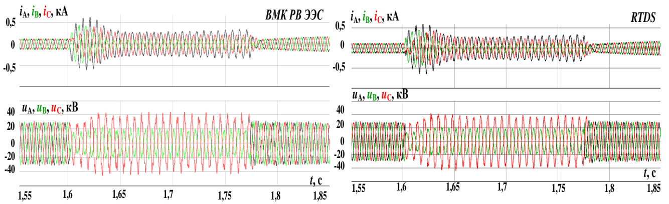
Рисунок 3.39 – Осциллограммы фазных токов и напряжений в узле подключения ВЭУ к ЭЭС при междуфазном КЗ
