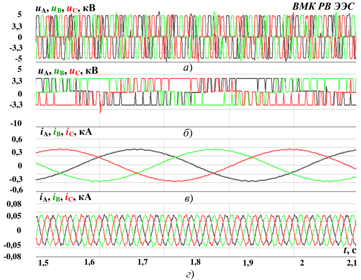
Рисунок 3.10 – Осциллограммы фазных токов и напряжений ВПТ ВЭУ ВМК РВ ЭЭС
