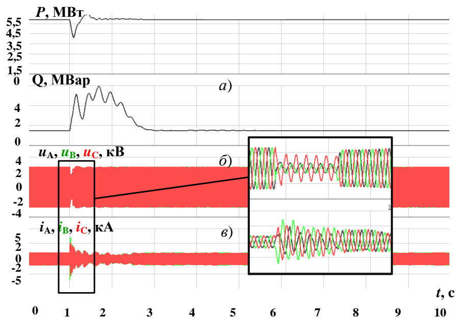
Рисунок Б.13 – Осциллограммы активной (а) и реактивной (б) мощности, фазных токов (г) и напряжений (в) на выходе ВПТ при междуфазном КЗ
