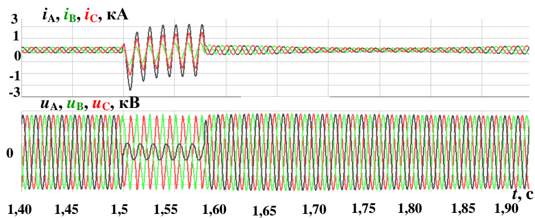
Рисунок 4.24 – Осциллограммы фазных токов и напряжений ЛЭП 110 кВ ПС 3 при однофазном КЗ
