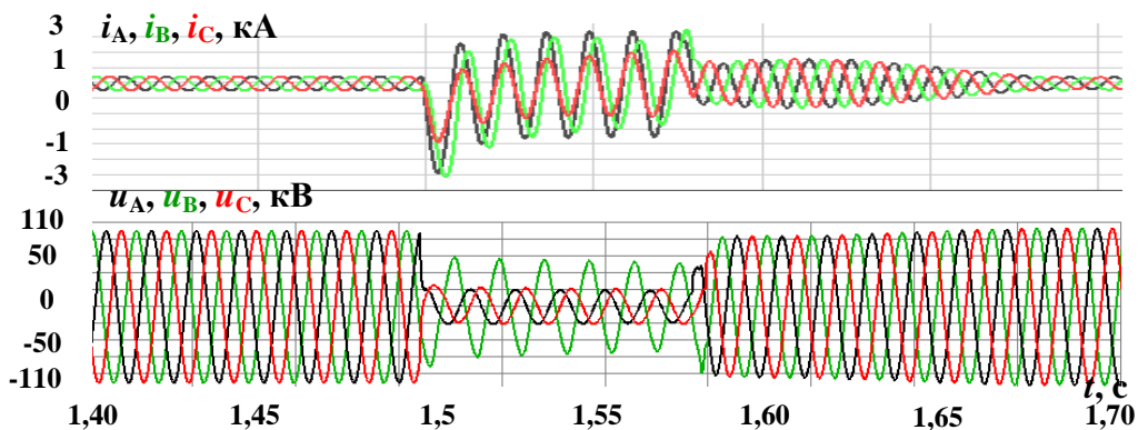
Рисунок 4.31— Осциллограммы фазных токов и напряжений ЛЭП 110 кВ ГРЭС при междуфазном КЗ
