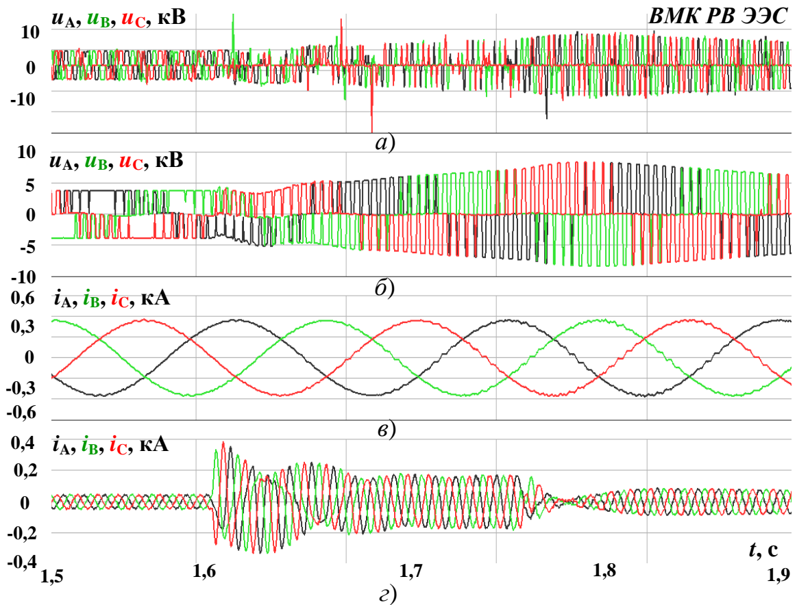
Рисунок 3.29 – Осциллограммы фазных токов и напряжений ВПТ ВЭУ ВМК РВ ЭЭС при трехфазном КЗ
