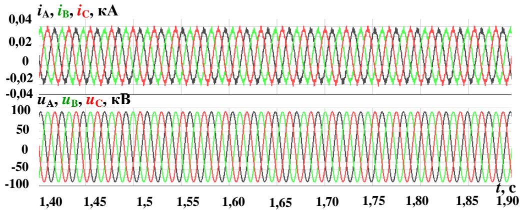
Рисунок 4.4 – Осциллограммы фазных токов и напряжений в узле присоединения ВЭУ при трехфазном КЗ
