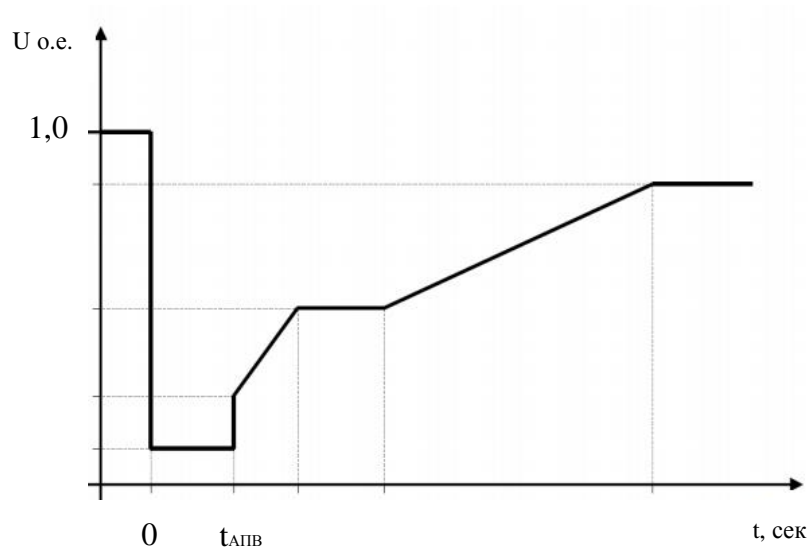
Рисунок 3.24 – Структура зависимости U=f(t) в узле подключения ВЭУ, соответствующей появлению в энергосистеме короткого замыкания и выходу из аварийного режима
