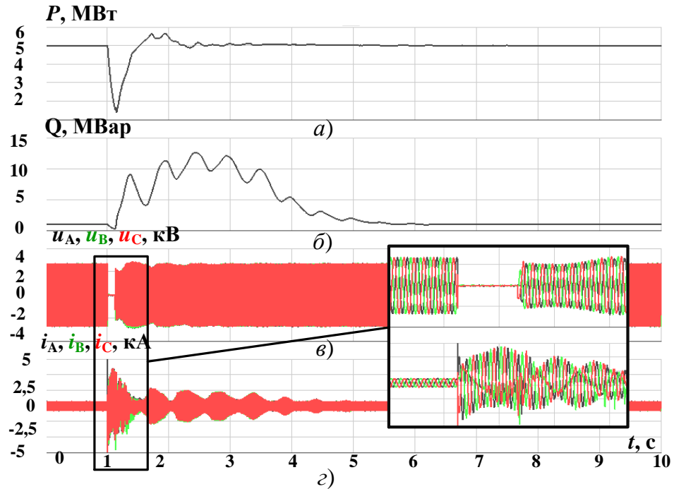
Рисунок 4.14 – Осциллограммы активной (а) и реактивной (б) мощности, фазных токов (г) и напряжений (в) на выходе ВПТ при трехфазном КЗ
