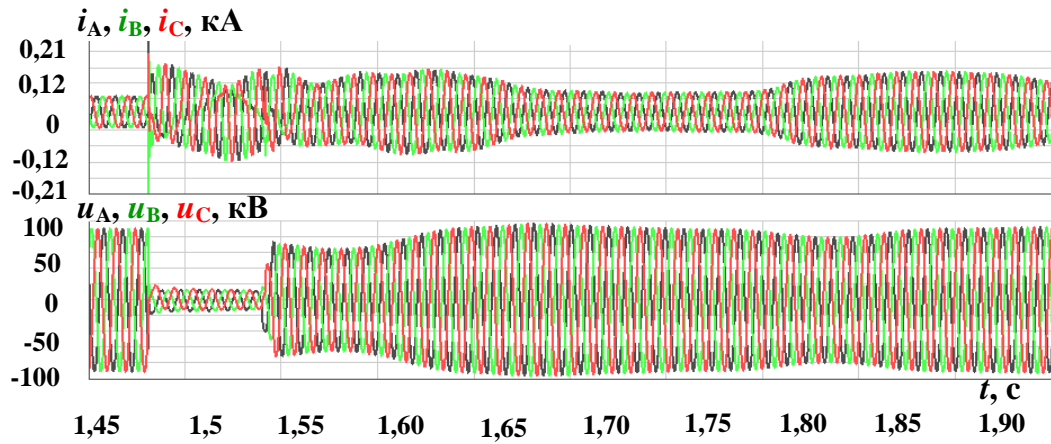
Рисунок Б.3 – Осциллограммы фазных токов и напряжений в узле присоединения ВЭУ при трехфазном КЗ
