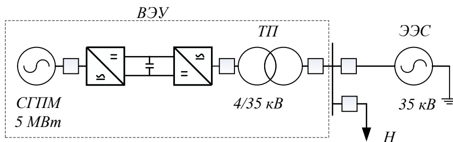
Рисунок 3.5 – Тестовая схема ЭЭС
