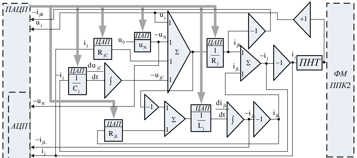
Рисунок 2.16 – Функциональная схема j -ой фазы ГСП ФВГ
