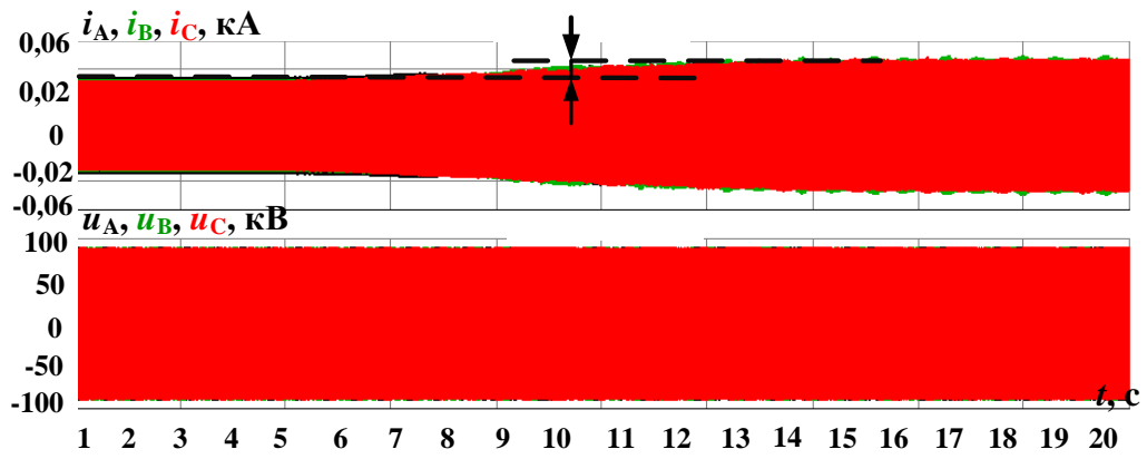
Рисунок 4.10 – Осциллограммы фазных токов и напряжений в узле присоединения ВЭУ
