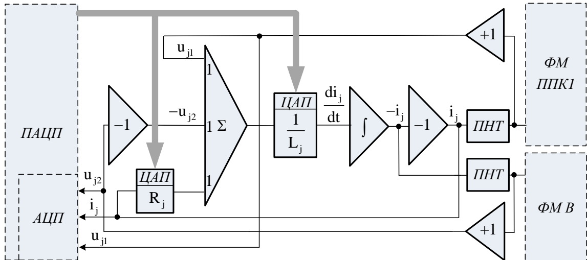
Рисунок 2.8 – Функциональная схема j -ой фазы ГСП Р
