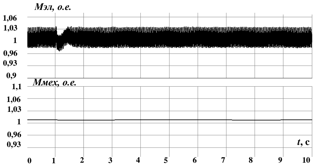
Рисунок 4.15 – Осциллограммы электромагнитного и механического моментов при трехфазном КЗ
