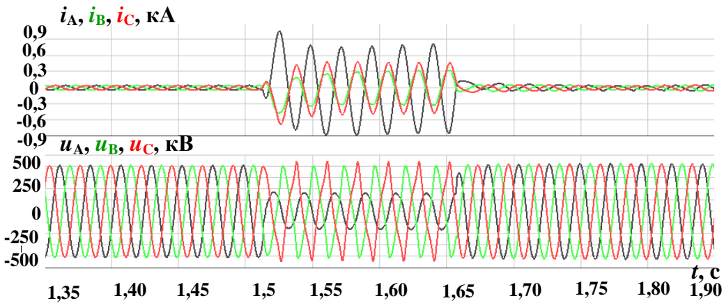
Рисунок 4.23– Осциллограммы фазных токов и напряжений ЛЭП 500 кВ ПС 1 при однофазном КЗ
