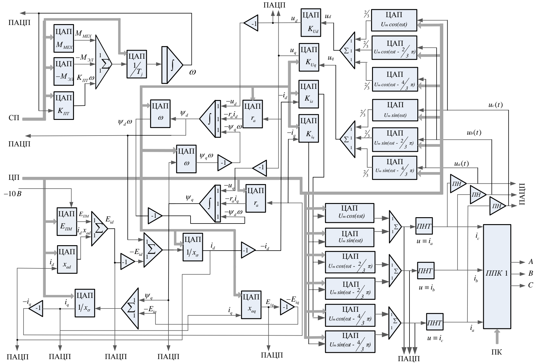
Рисунок 2.4 – Функциональная схема ГСП СГПМ
