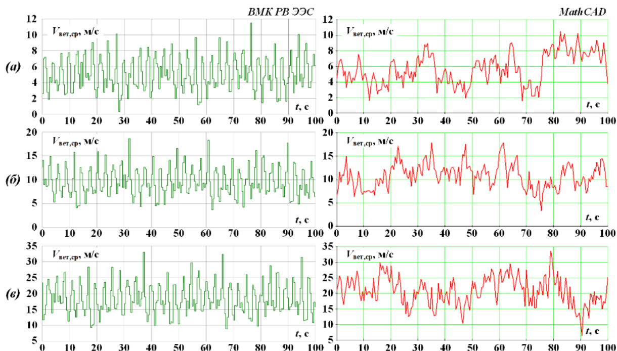
Рисунок 3.1 – Результаты моделирования ветра
