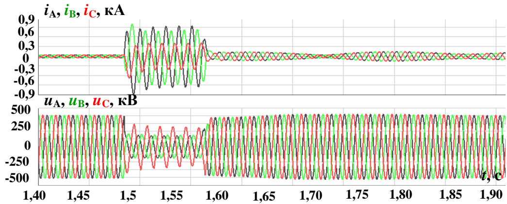
Рисунок 4.29 – Осциллограммы фазных токов и напряжений ЛЭП 500 кВ ПС 1 при междуфазном КЗ
