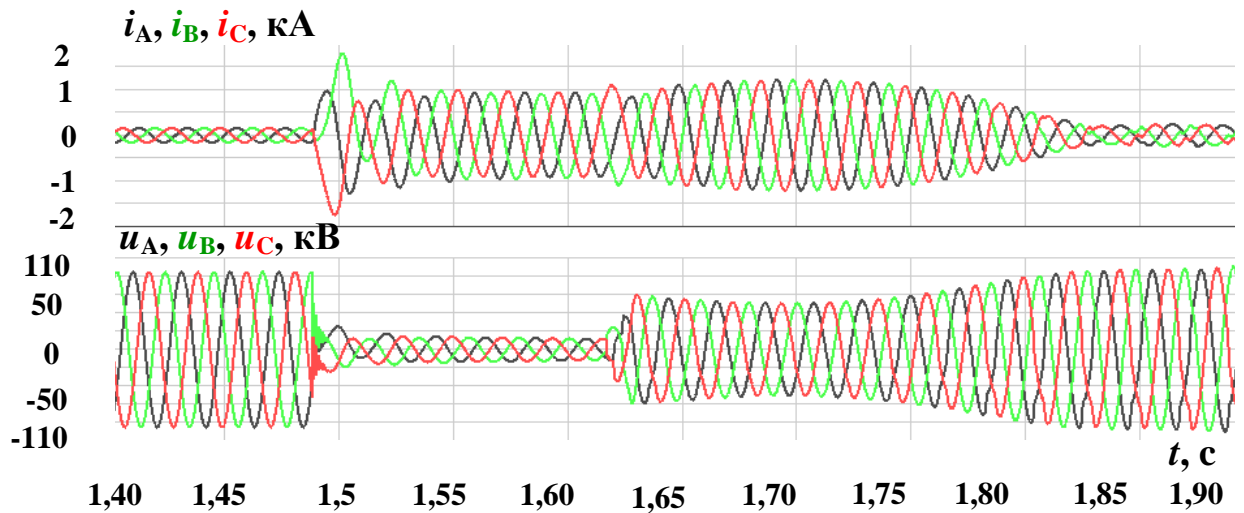
Рисунок 4.19 – Осциллограммы фазных токов и напряжений ЛЭП 110 кВ ПС 4 при трехфазном КЗ
