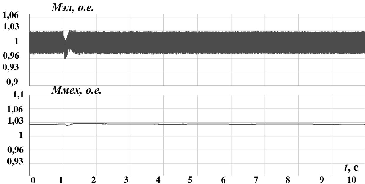
Рисунок 4.21– Осциллограммы электромагнитного и механического моментов при однофазном КЗ
