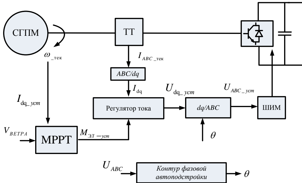
Рисунок 2.10 – Схема управления ФМ В
