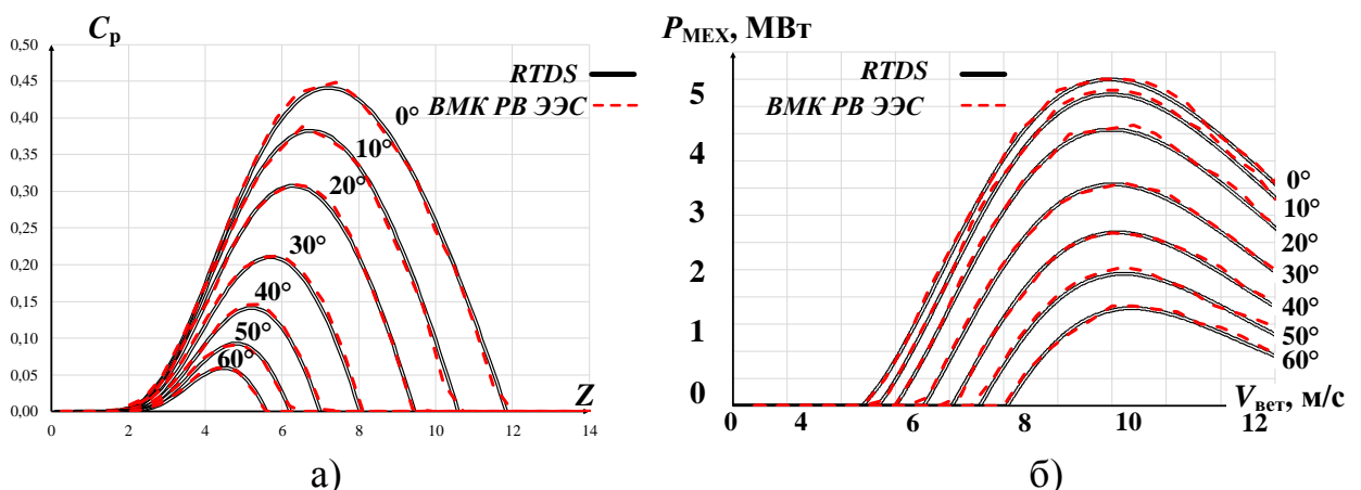
Рисунок 3.2 – Зависимость коэффициента мощности C_p от быстроходности Z при разных углах поворота лопасти (а), Зависимость мощности турбины P_{MEX} от скорости ветра V_0 при разных углах поворота лопасти (б)
