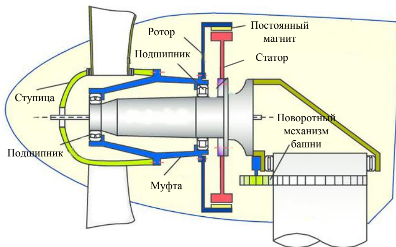
Рисунок 1.4 – Структура трансмиссии ВЭУ
