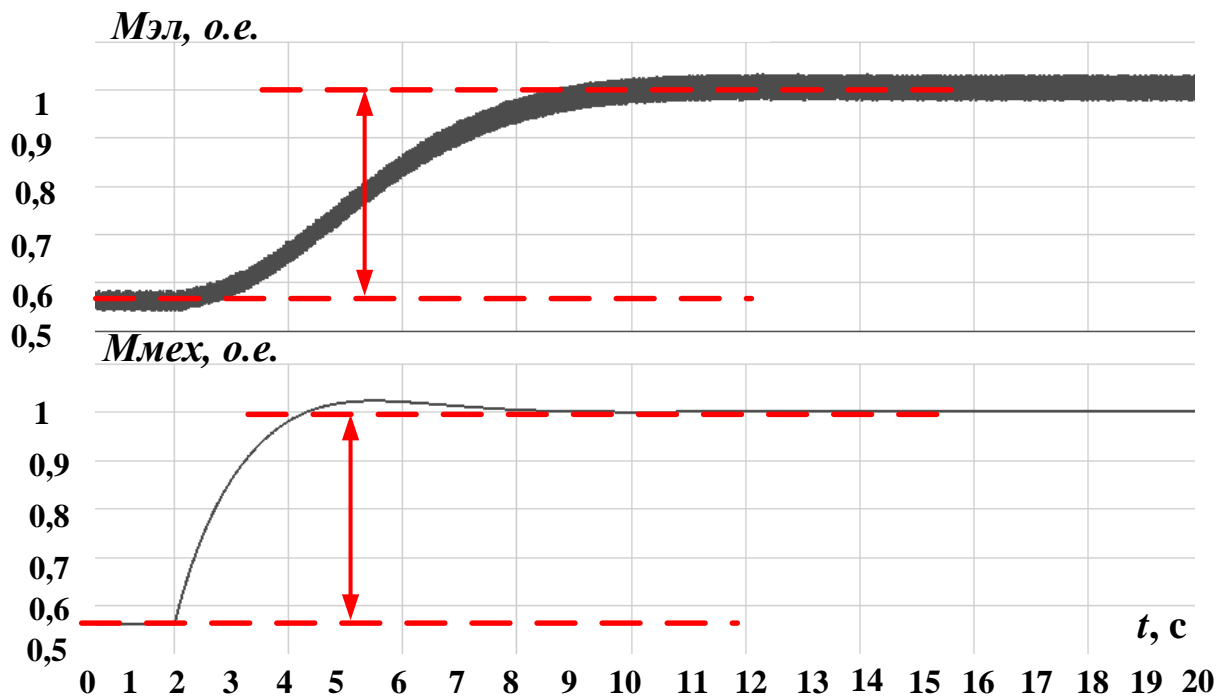
Рисунок 4.9 – Осциллограммы электромагнитного и механического моментов
