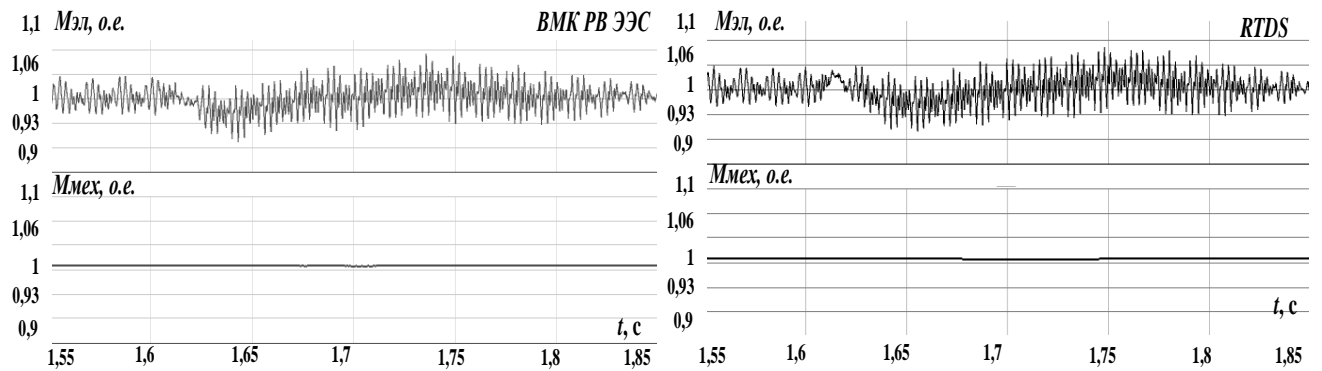
Рисунок 3.40 – Осциллограммы электромагнитного и механического моментов ВЭУ при междуфазном КЗ
