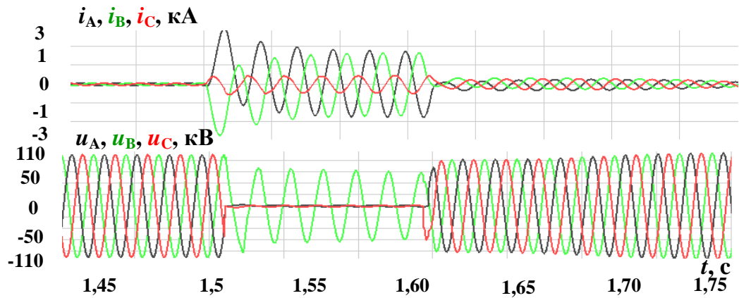
Рисунок Б.18 – Осциллограммы фазных токов и напряжений ЛЭП 110 кВ ГРЭС при междуфазном КЗ
