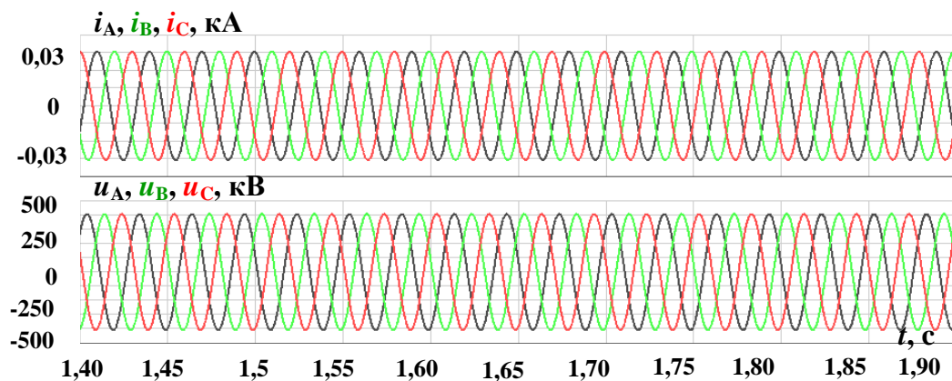
Рисунок 4.5 – Осциллограммы фазных токов и напряжений ЛЭП 500 кВ ПС 1
