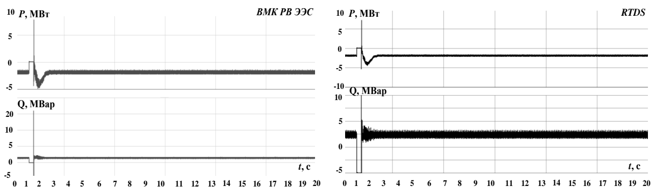
Рисунок 3.26 – Осциллограммы перетока активной и реактивной мощности в ЭЭС при трехфазном КЗ
