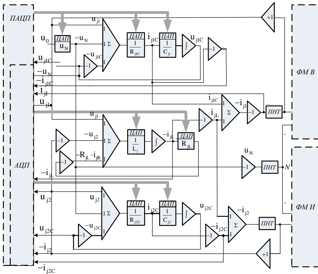
Рисунок 2.12 – Структурная схема j -го полюса ГСП ЦПТ
