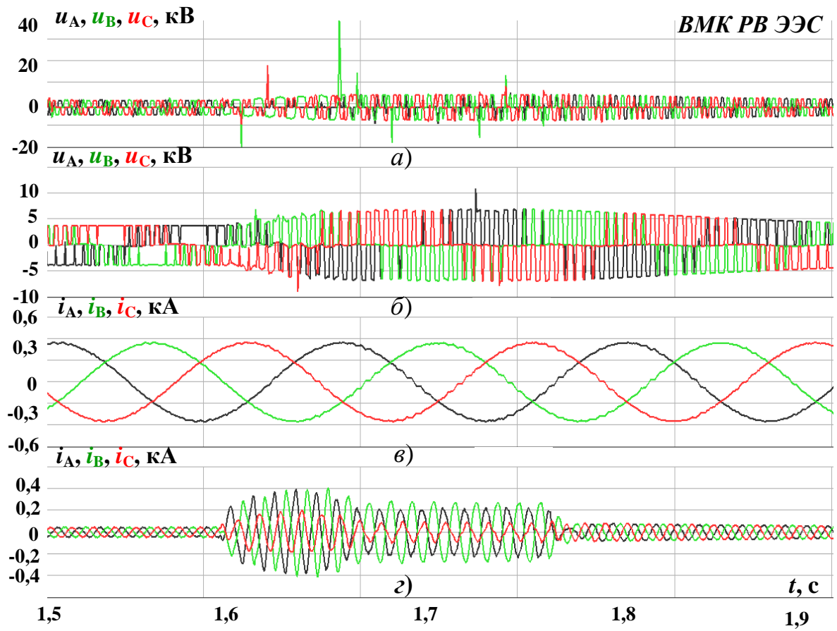
Рисунок 3.35 – Осциллограммы фазных токов и напряжений ВПТ ВЭУ ВМК РВ ЭЭС при однофазном КЗ
