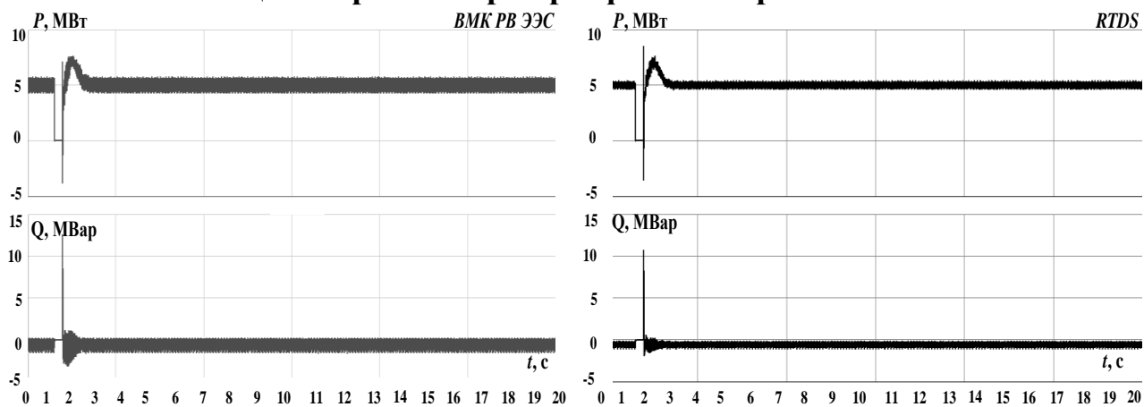
Рисунок 3.25 – Осциллограммы активной и реактивной мощности ВЭУ при трехфазном КЗ
