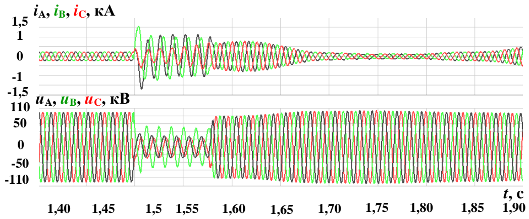
Рисунок Б.17 – Осциллограммы фазных токов и напряжений ЛЭП 110 кВ ПС 3 при междуфазном КЗ
