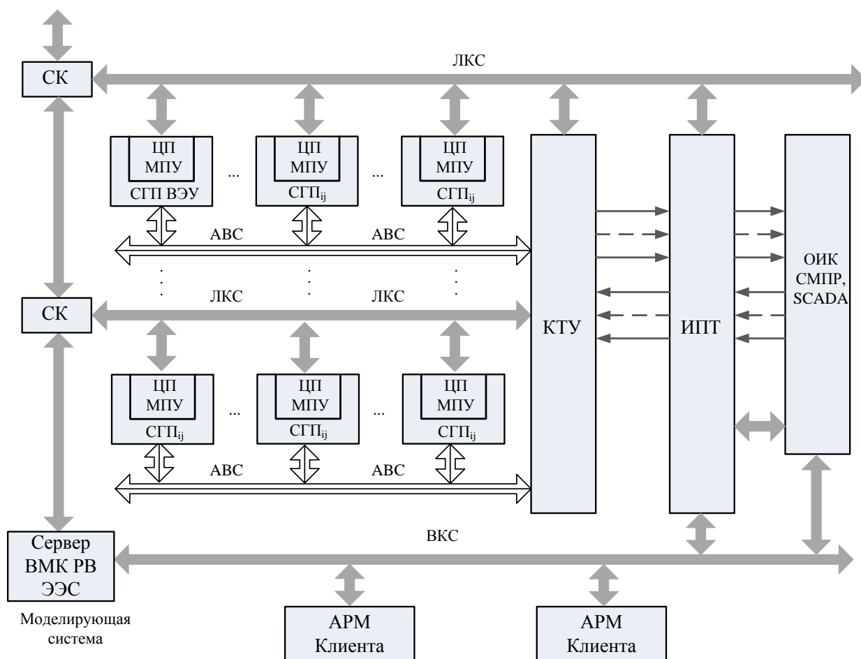
Рисунок 2.1 – Структурная схема ВМК РВ ЭЭС
