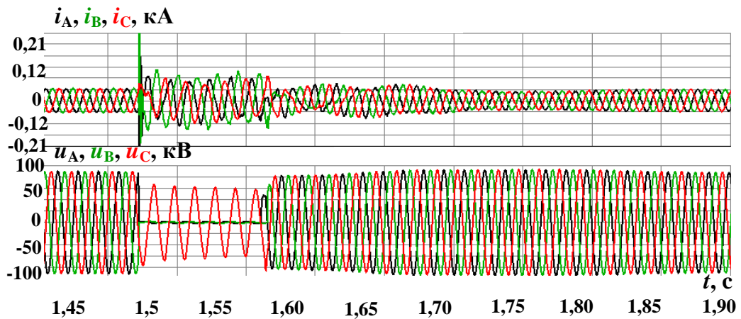
Рисунок 4.28 – Осциллограммы фазных токов и напряжений в узле присоединения ВЭУ при междуфазном КЗ
