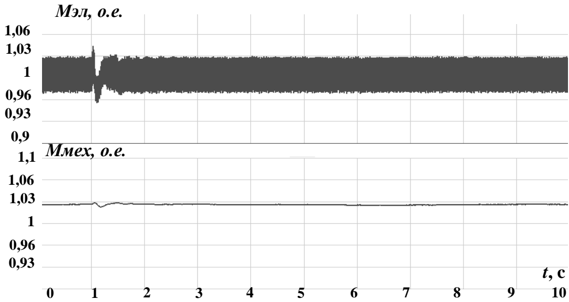
Рисунок 4.27 – Осциллограммы электромагнитного и механического моментов при междуфазном КЗ
