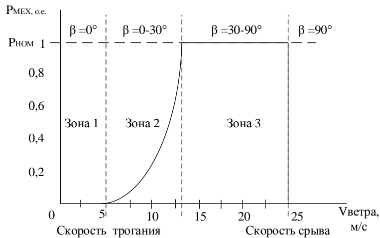
Рисунок 1.2 – Зависимость мощности P_{MEX} от \beta
