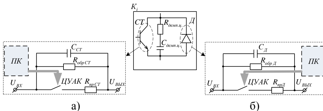
Рисунок 2.6 – ЦУ ФМ i -го ключа
