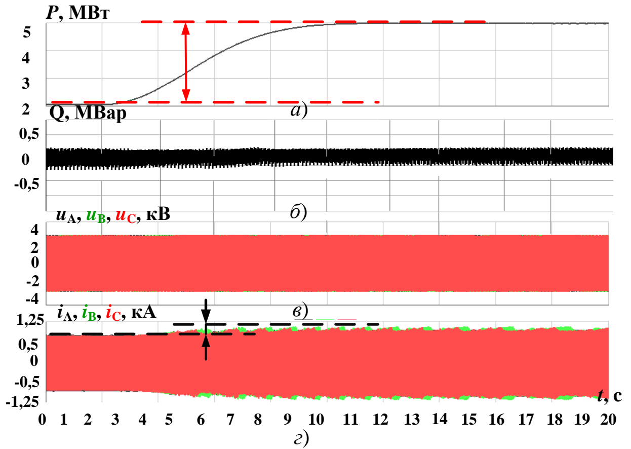
Рисунок 4.8 – Осциллограммы активной (а) и реактивной (б) мощности, фазных токов (г) и напряжений (в) на выходе ВПТ
