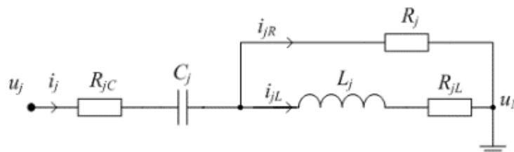
Рисунок 2.15 – Схема замещения j -ой фазы ФВГ
