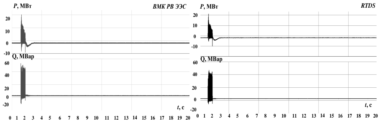
Рисунок 3.38 – Осциллограммы перетока активной и реактивной мощности в ЭЭС при междуфазном КЗ
