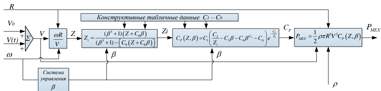
Рисунок 1.1 – Функциональная схема математической модели
