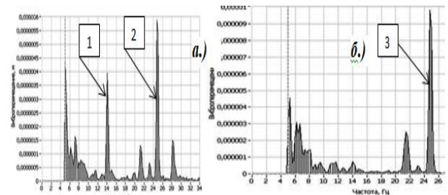
Рисунок 35 – Результаты эксперимента при определении резонансных частот \Omega_i^* на узлах станка при тестовом воздействии в виде спектрограмм СКЗ виброперемещений в направлении действия силы \Delta F_{рез\ y}
