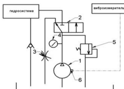
Рисунок 36 – Схема включения в гидропривод устройства для подсоединения диагностического оборудования
