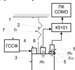
1 – основание, 2 – пружина, 3 – масса, 4 – генератор электромеханический, 5 – испытуемый образец, 6, 8 – акселерометры, 7 – электрический генератор сигналов специальной формы Рисунок 38 – Устройство для определения демпфирующих свойств материалов
