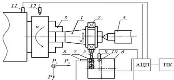
Рисунок 34 – Принципиальная схема устройства для определения динамической жесткости несущих узлов токарно-винторезного станка
