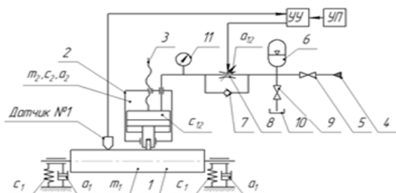
Рисунок 25 – Кинематическая схема виброгасителя вязкого трения
