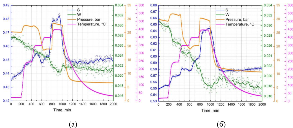
Рисунок 7 – Зависимости S(t) , W(t) , P(t) , T(t) , после отжига в вакууме и при нагреве в среде водорода а) Mg; б) композита \text{Mg-Cr}_2\text{O}_3
