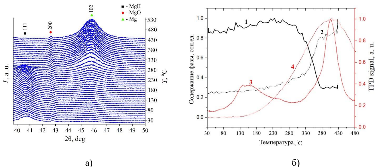
Рисунок 2 – Дифракционные картины in situ PCA а) композит \text{MgH}_2\text{--Cr}_2\text{O}_3 ; б) график фазового перехода с нормированными спектрами температурно-программированной десорбции; 1 - фаза \text{MgH}_2 ; 2 - фаза Mg; 3 - спектры температурно-программированной десорбции \text{H}_2 для композита \text{MgH}_2\text{--Cr}_2\text{O}_3 ; 4 - спектры температурно-программированной десорбции \text{H}_2 для \text{MgH}_2
