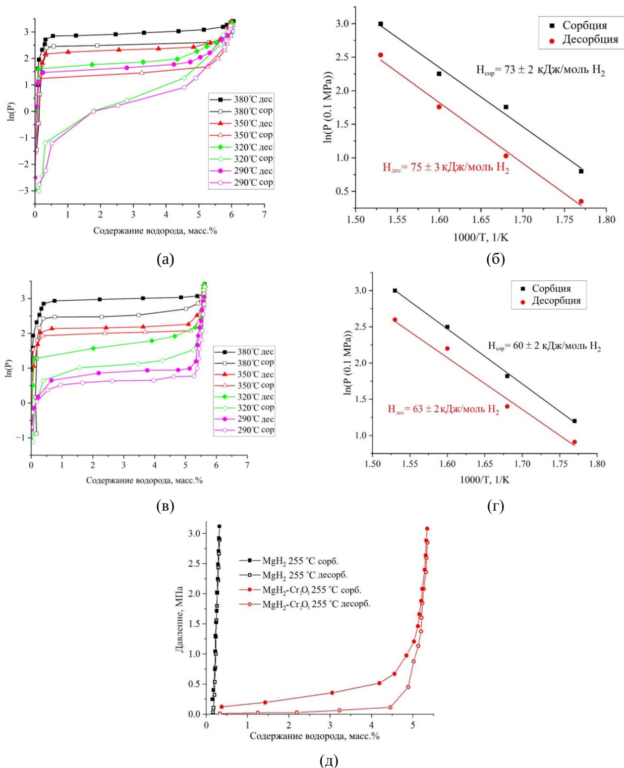
Рисунок 6 – PCT-кривые сорбции/десорбции водорода
