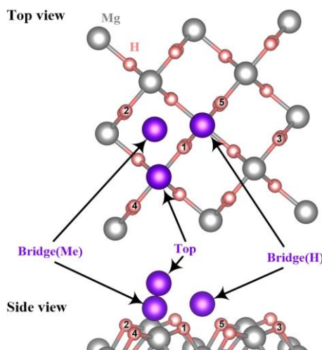
Рисунок 5 – Вид сверху и сбоку пленки \text{MgH}_2 с атомом Cr или O, адсорбированным на поверхности.
