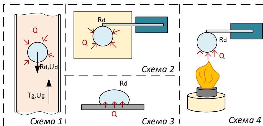
Рисунок 14 - Схемы нагрева капль с доминированием кондуктивного, конвективного, радиационного, а также смешанного теплообмена
