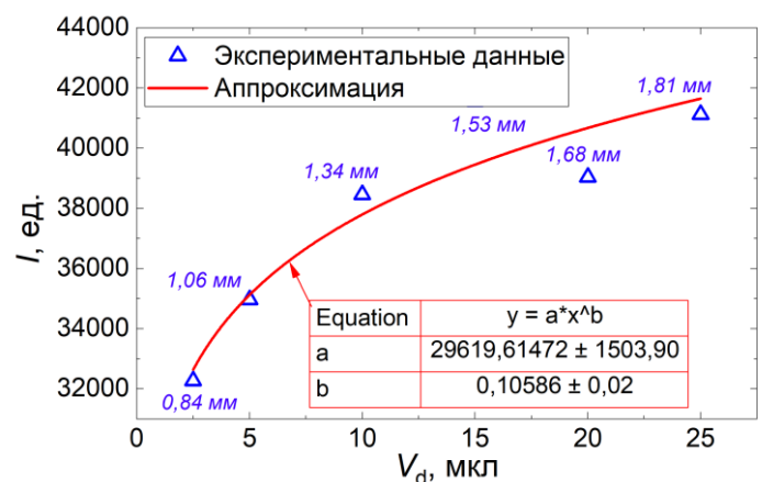
Рисунок 3 - Зависимость интенсивности свечения капли от ее объема
