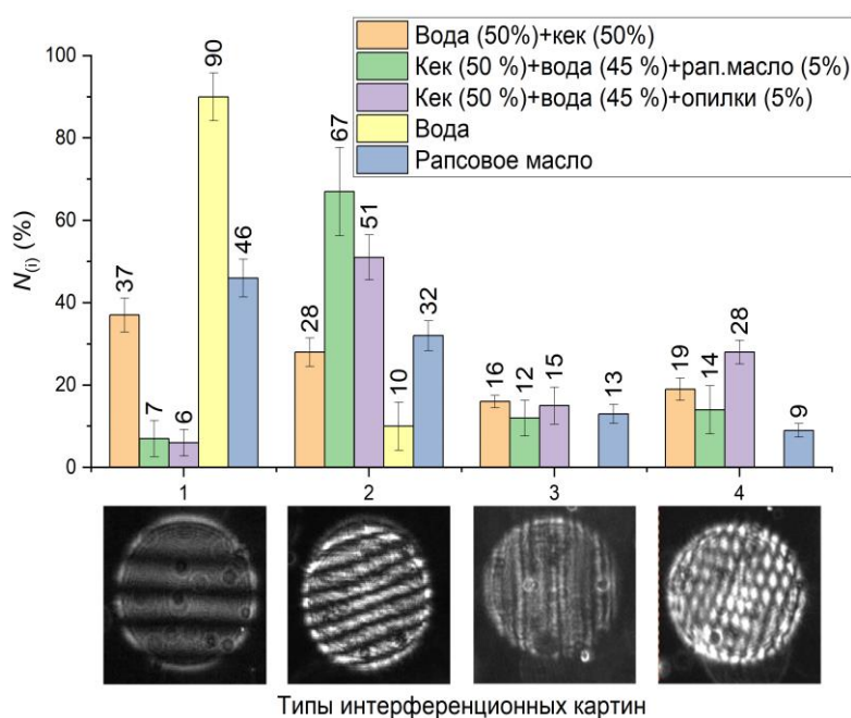
Рисунок 10 - Содержание образов четырех типов интерференционных картин в аэрозольном потоке исследуемых составов ( G_a=50 кг/ч)
