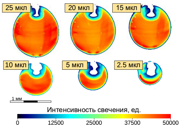
Рисунок 2 - Видеограммы капель воды без примесей при варьировании объема последних в диапазоне V_d=2,5\text{--}25 мкл
