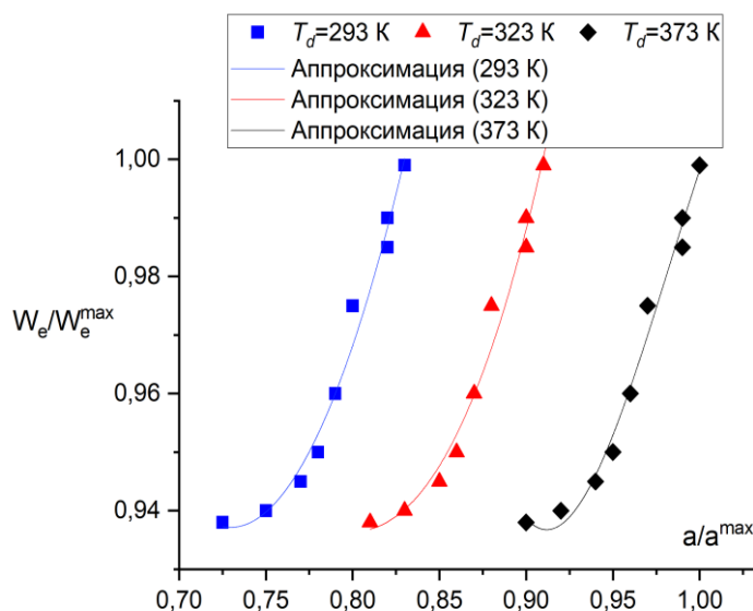
Рисунок 13 - Зависимости относительных массовых скоростей испарения капель исследованных составов от их относительной температуропроводности для трех начальных температур жидкости ( R_d \approx 1\text{ мм} , T_g \approx 573\text{ К} )
