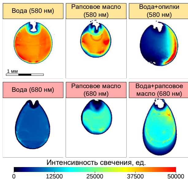
Рисунок 6 - Видеограммы капель исследовавшихся составов, полученные при использовании двух различных типов оптических светофильтров
