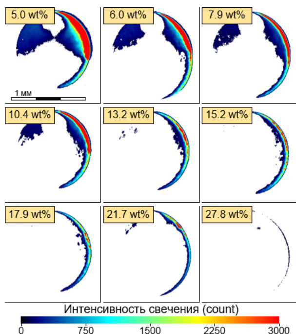
Рисунок 4 - Видеограммы капель суспензии при варьировании массовых концентраций (5–27.8 %) кека
