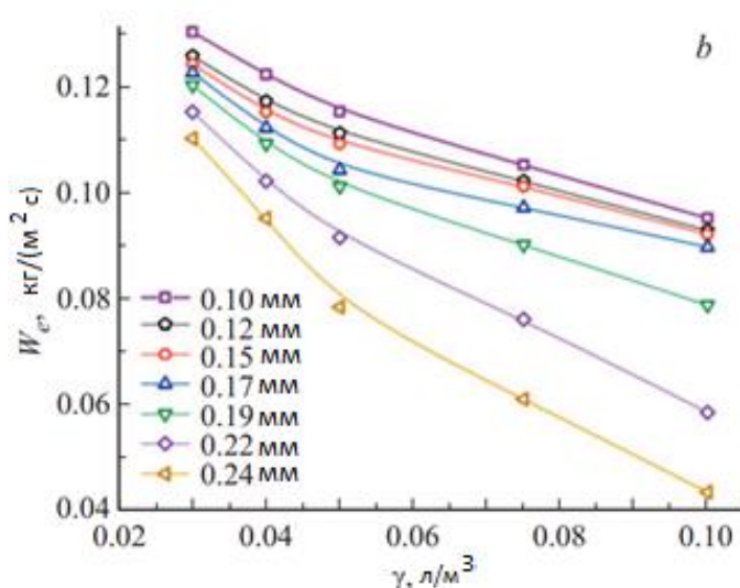
Рисунок 19 - Зависимости скорости испарения каплей от концентрации при разных начальных размерах
