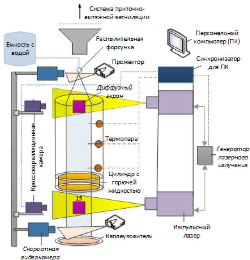
Рисунок 12 - Схема экспериментального стенда
