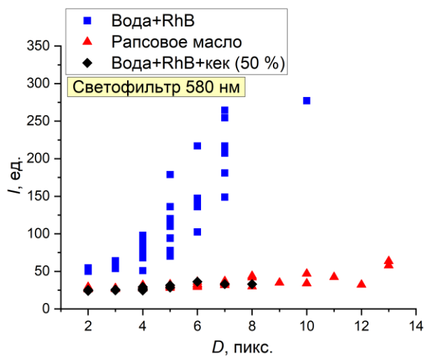
Рисунок 8 - Зависимости интенсивности свечения отдельных капель в потоке от их размеров
