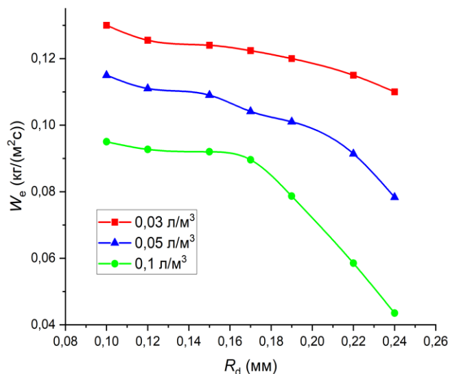
Рисунок 18 - Значения скоростей испарения каплей воды в высокотемпературной газовой среде при разных начальных размерах
