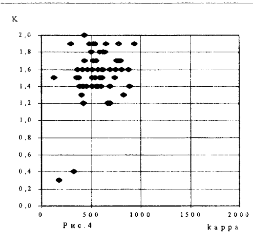
Поля корреляций магнитной восприимчивости ( \cdot 10^{-4} ед.СИ) с радиоактивностью (мкР/ч) (рис.1), ураном (г/т) (рис.2), торием (г/т) (рис.3) и калием (%) (рис. 4).
