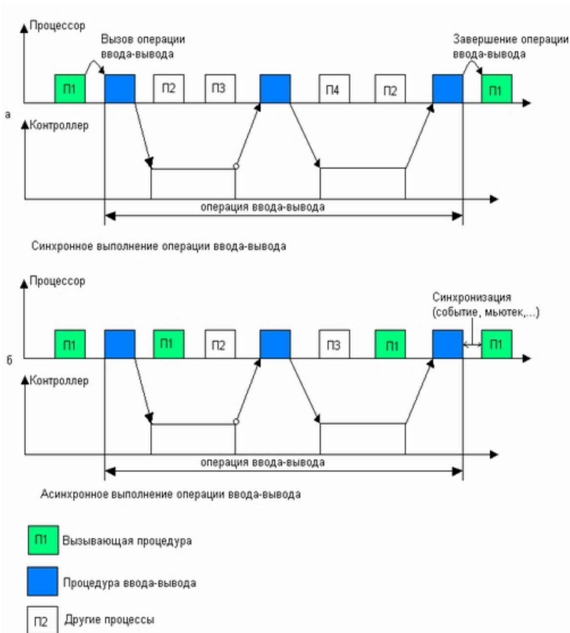
Рис. 4.12. Два режима выполнения операций ввода-вывода
