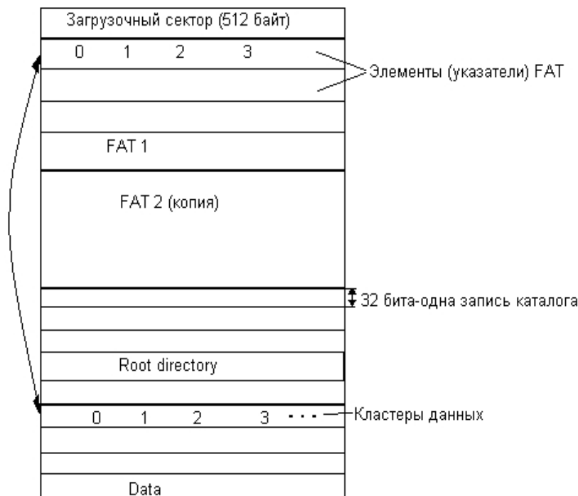
Рис. 4.21. Физическая структура файловой системы FAT
