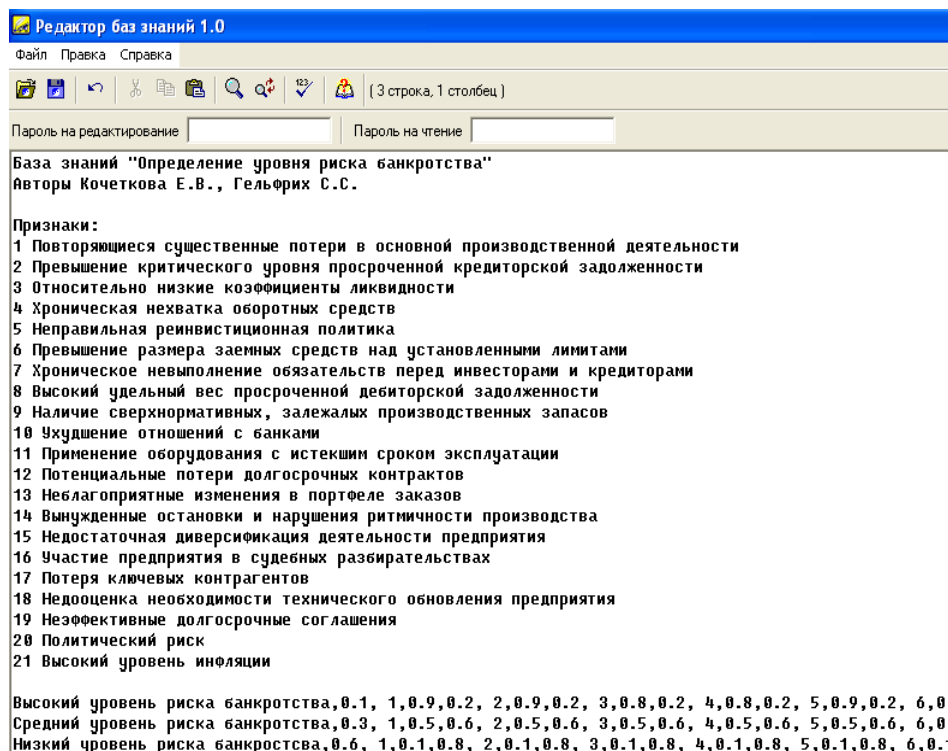
Рис. 5.24. Окно редактора базы знаний «Малой экспертной системы» v 2.0
