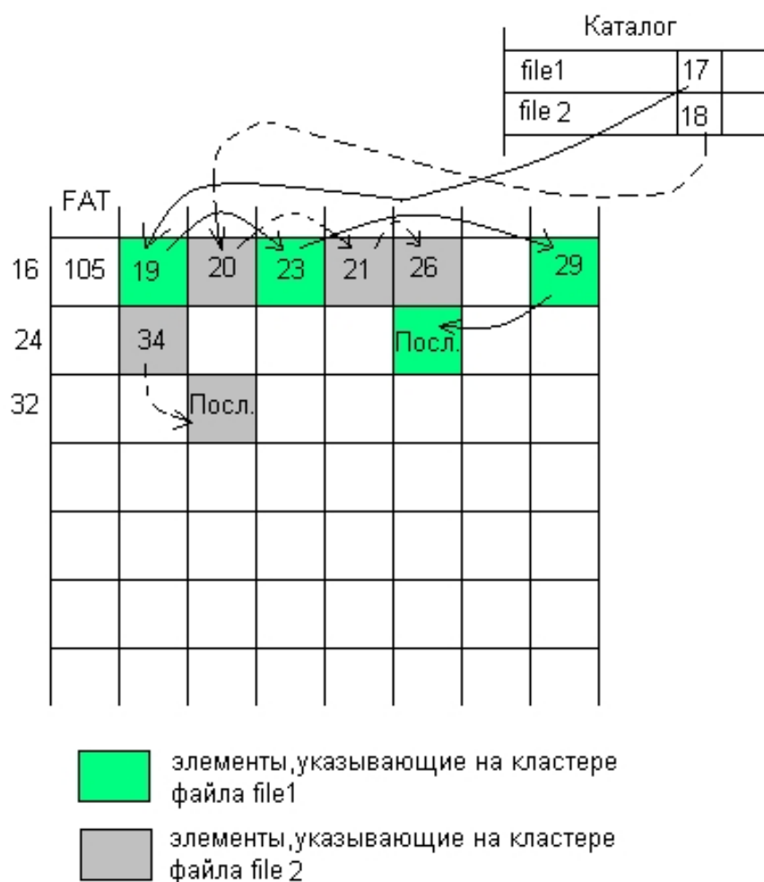
Рис. 4.22. Списки указателей файлов в FAT
