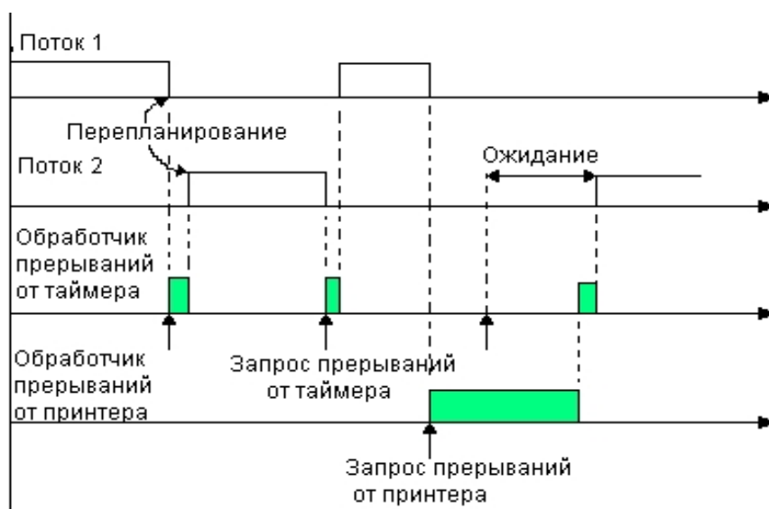
Рис. 4.11. Неупорядоченная обработка прерываний
