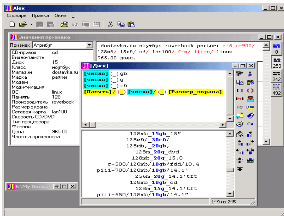
Рис. 5.17. Визуальная среда ALEX
