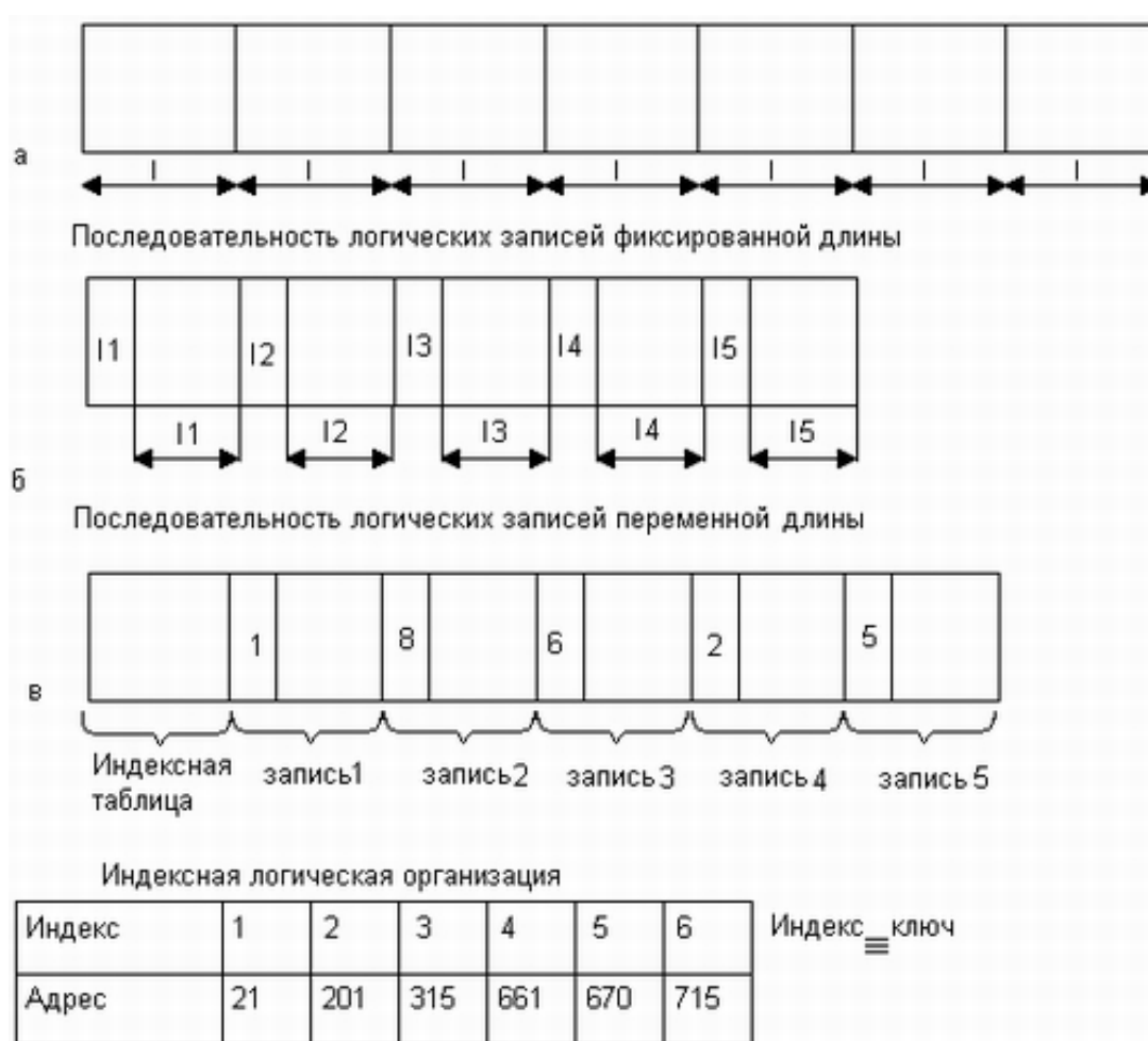
Рис. 4.16. Способы логической организации файлов
