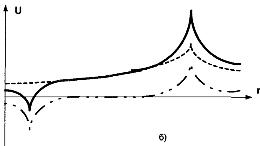
Рис. 5.2. Однофазное короткое замыкание на шинах ПС высокого напряжения:
