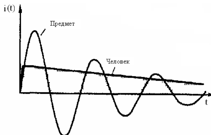
Рис. 2.6. Кривая изменения тока при разряде тела человека или проводящего предмета (например, малогабаритной мебели)
