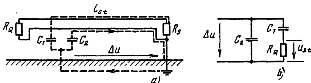
Рис. 3.19. Односторонне заземленная линия с большими емкостями на землю C_1 и C_2 (а) и ее схема замещения при R_S \gg R_Q (б)
