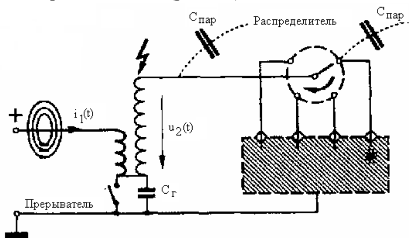
Рис. 2.3. Возбуждение импульса высокого напряжения в автомобильных устройствах зажигания:
