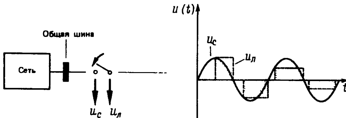
Рис. 2.8. Возникновение перенапряжения при включении короткой ненагруженной линии (идеальный случай)
