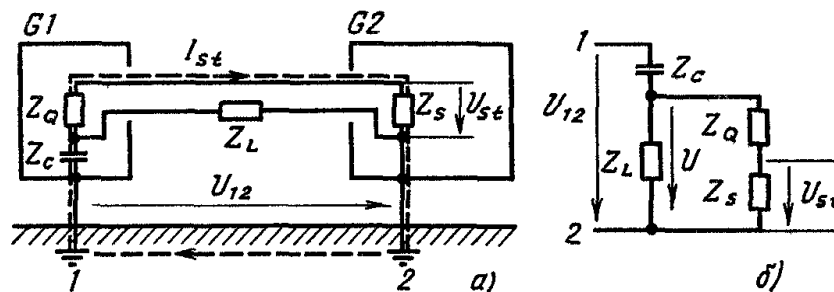
Рис. 3.11. Гальваническое влияние через разомкнутую петлю заземлений: а – схема устройства; б – схема, поясняющая формирование напряжений помехи U_{st}
