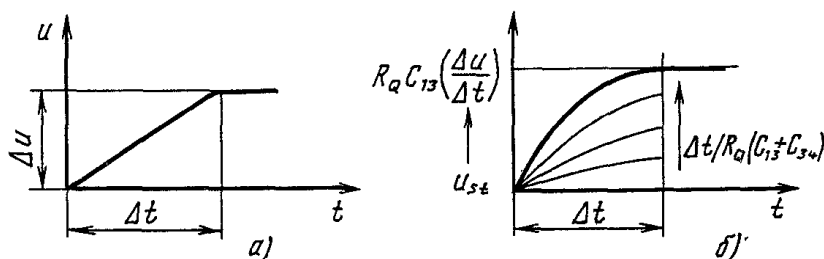
Рис. 3.14. Выходной сигнал элемента А на рис. 3.13, а (а) и сигнал помехи u_{st} в интервале времени 0 \leq t \leq \Delta t (б)
