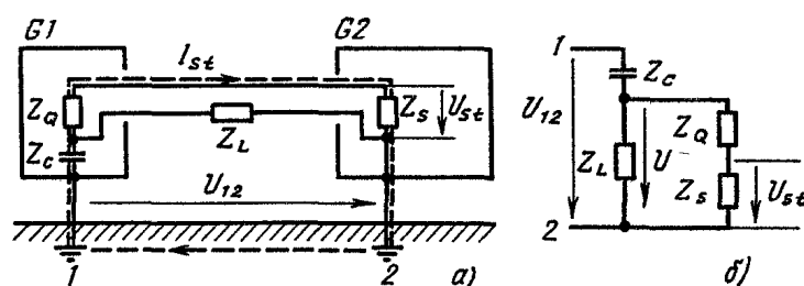
Рис. 3.9. Гальваническое влияние через замкнутую петлю заземления: а – схема устройства; б – схема, поясняющая формирование напряжения помехи U_{st}
