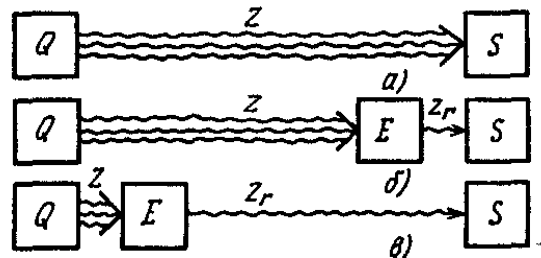
Рис. 4.1. Взаимные расположения источника помех Q , приемника S и защитного компонента E : а – защита отсутствует; б – защита приемника; в – подавление помехи у источника
