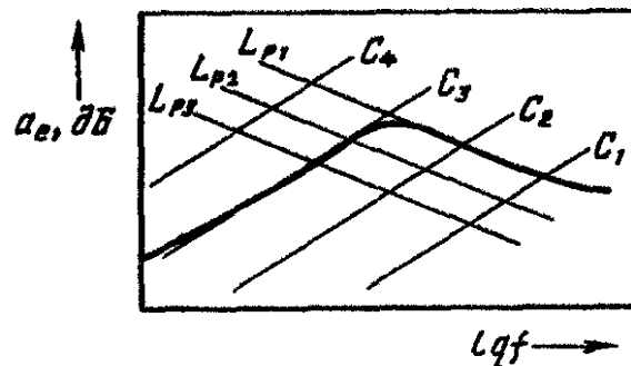
Рис. 4.11. Коэффициент затухания a_e фильтра, состоящего из реальных конденсаторов, в зависимости от частоты f : L_{p3} > L_{p2} > L_{p1} ; C_4 > C_3 > C_2 > C_1
