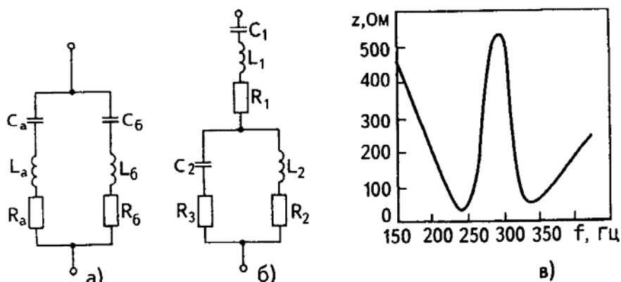
Рис. 6.6. Одночастотный фильтр (а), фильтр двойной настройки (б) и расчетная зависимость сопротивления от частоты фильтра 5-й и 7-й гармоник на подстанции Эчинген (в)
