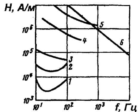
Рис. 7.2. Эффекты воздействия магнитного поля разной частоты на человека: 1 – появление мерцания на периферийных участках поля зрения; 2 – ощущение наличия поля; 3 – объективно регистрируемые нарушения зрения, недомогание, головные боли; 4 – нарушение работы сердца; 5 – нарушение работы нервной системы; 6 – джоулев нагрев тканей при мощности 4 Вт/кг
