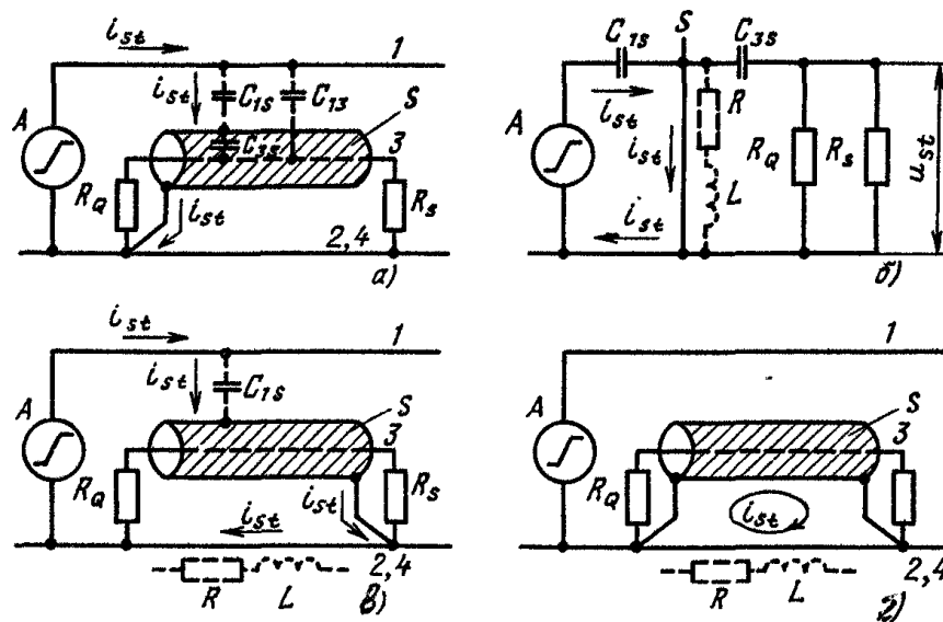
Рис. 3.16. Экранирование линии: a – целесообразное соединение экрана S с системой опорного потенциала 2, 4; б – схема замещения; в – нецелесообразное соединение экрана с системой опорного потенциала; г – двустороннее соединение экрана с проводом опорного потенциала; A – источник помех ( \Delta u / \Delta t ); r_q – выходное сопротивление источника помех; R_s – входное сопротивление ступени в экранированном контуре
