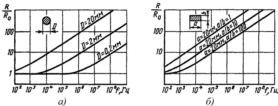
Рис. 3.3. Влияние проникновения тока на сопротивление проводов круглого (а) и прямоугольного (б) сечений
