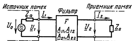
Рис. 4.3. Токовый контур с фильтром
