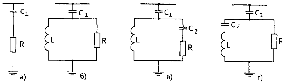
Рис. 6.7. Широкополосные высокочастотные фильтры: а) первого порядка; б) второго порядка; в) третьего порядка; г) С-типа
