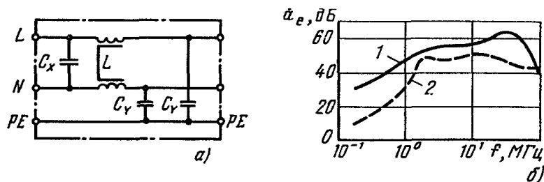
Рис. 4.14. Пример сетевого фильтра на 250 В, 1А: а – схема: C_X = 0,1 \text{ мкФ} , C_Y = 2 \times 3 \text{ нФ} , L = 2 \times 3,7 \text{ мГн} ; б – частотная зависимость \alpha_e , схемы измерений, согласно рис. 4.5: 1 – асимметричные помехи, 2 – симметричные помехи
