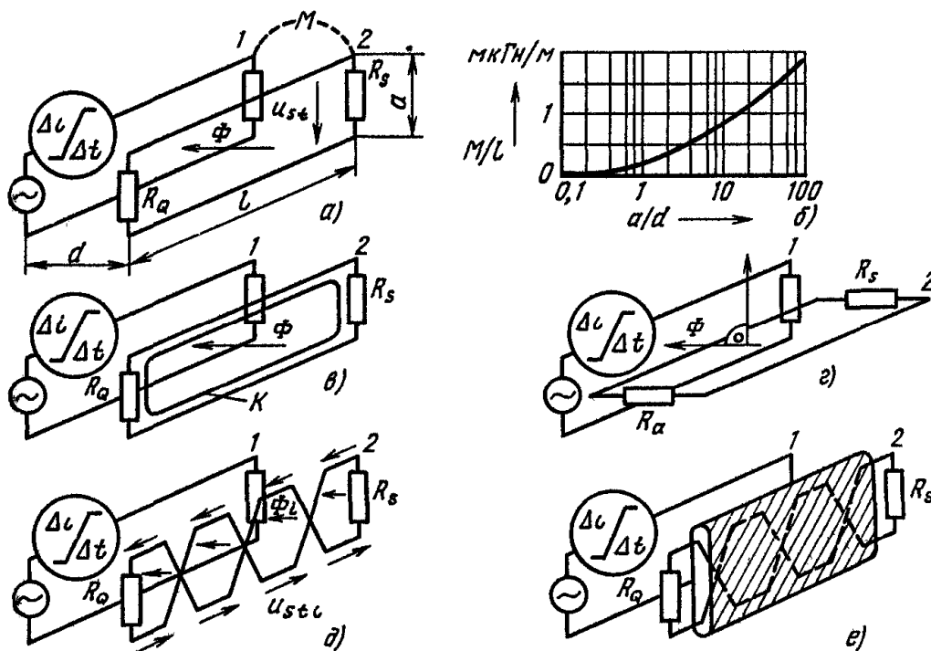
Рис. 3.22. Индуктивное влияние между промышленными токовыми контурами: а – принципиальная схема двух токовых контуров 1 и 2 с расстоянием d между ними; б – погонная взаимная индуктивность M/l в зависимости от a/d ; в-е – меры по снижению влияния (пояснения см. в тексте)
