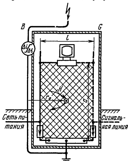
Рис. 3.25. Индуктивное влияние тока молнии на электрический контур внутри здания G , образованный проводами питания и сигнальными линиями при ударе молнии в молниеприемник здания B
