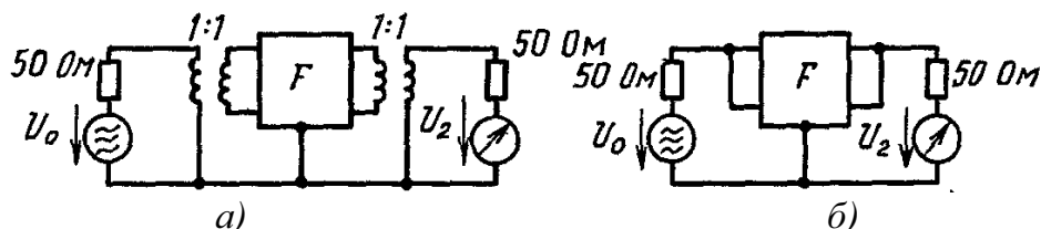
Рис. 4.5. Схемы для измерений симметричного (а) и асимметричного коэффициентов затуханий (б) a_e фильтров: при \dot{Z}_O = \dot{Z}_S = 50 \text{ Ом} , из выражения (4.10) следует a_e = 20 \lg U_0/2 U_2 , дБ, так как U_{20} = U_0/2 согласно (4.9)
