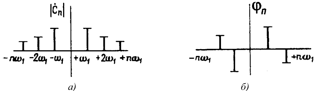
Рис. 1.9. Амплитудный и фазовый спектры комплексного ряда Фурье
