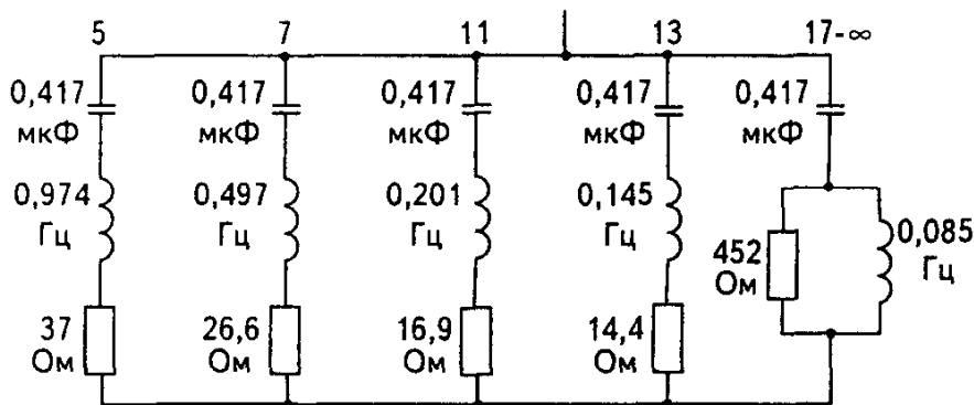
Рис. 6.8. Фильтр переменного тока
