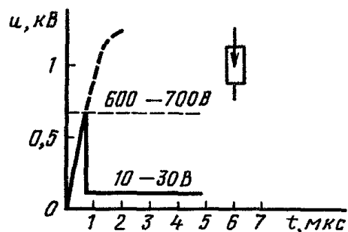
Рис. 4.19. Типичная характеристика зажигания газонаполненного разрядника
