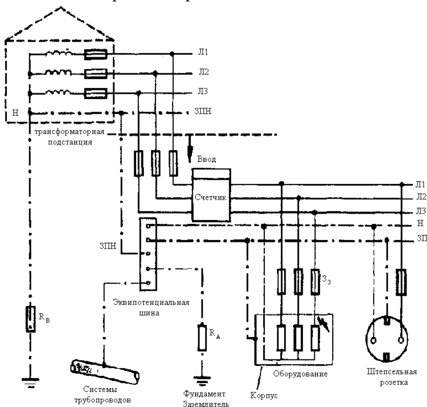
Рис. 1.4. Заземление в низковольтной сети:
