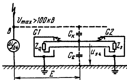
Рис. 3.21. Емкостное влияние молнии на линию: B – канал разряда молнии; G1, G2 – приборы; C_K, C_E – емкости связи относительно земли
