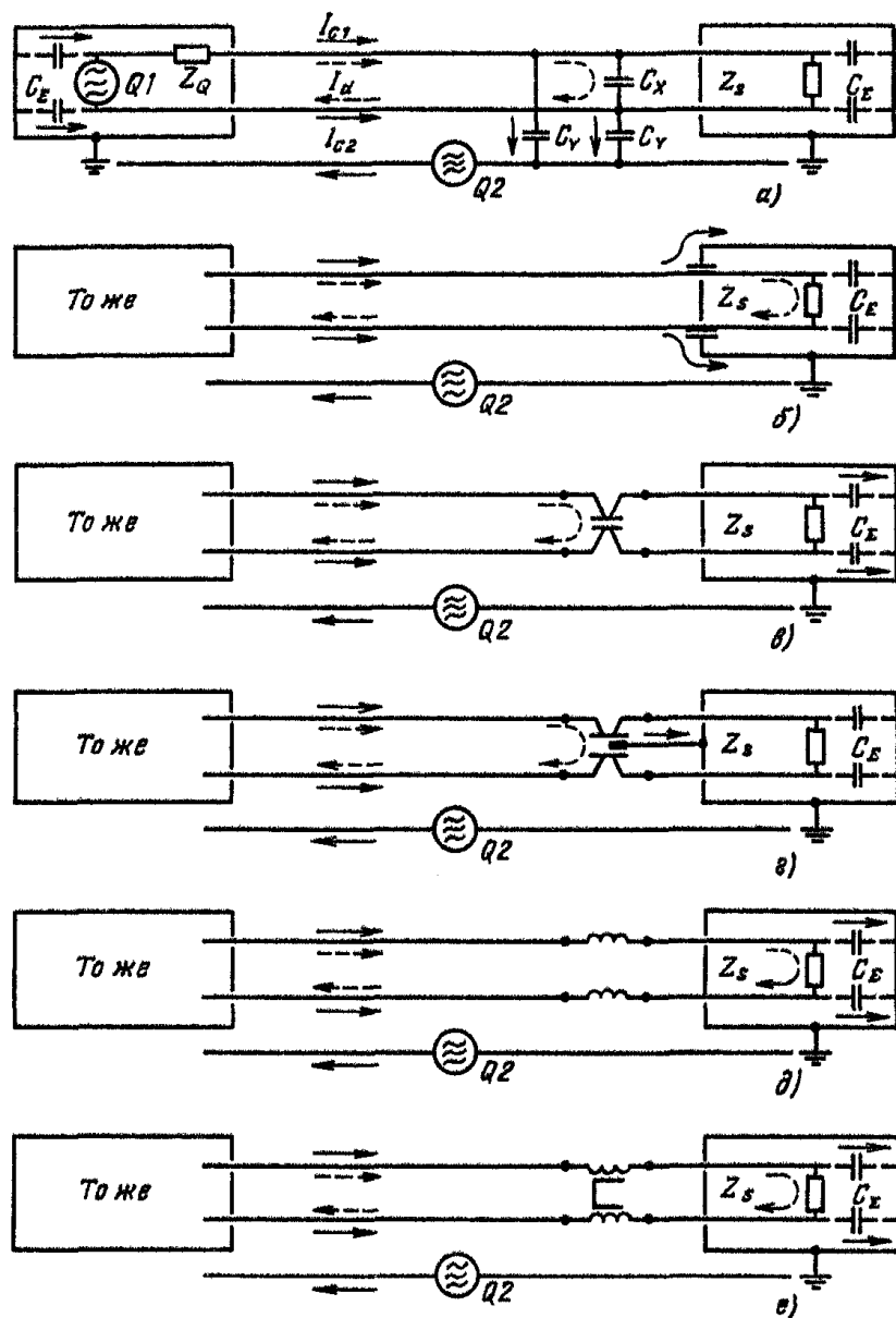
Рис. 4.8. Защита катушками индуктивности и конденсаторами от синфазных и противофазных токов помех (пояснения см. в тексте): Q_1, Q_2 – источники противофазных I_d и синфазных I_c токов помех; C_E – паразитные емкости участка схемы относительно заземленного корпуса
