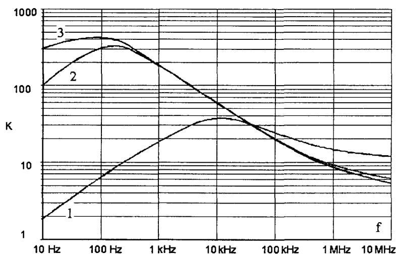
Рис. 5.5. Расчетные коэффициенты экранирования:
