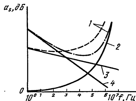
Рис. 4.25. Принципиальные зависимости коэффициентов затухания от частоты для электромагнитного поля в дальней зоне и для электрического в ближней: 1 – a_S = a_{SA} + a_{SR} ; 2 – a_{SA} ; 3 – a_{SR} для электромагнитного поля в дальней зоне (4.30); 4 – a_{SR} для электрического поля в ближней зоне (4.29)
