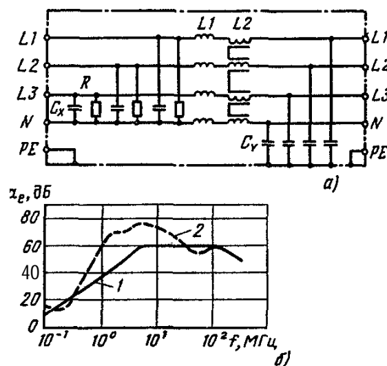
Рис. 4.15. Пример трехфазного сетевого фильтра на 440 В, 16 А: а – схема: L1 = 60 \text{ мГн} , L2 = 4,4 \text{ мГн} , C_X = 2,2 \text{ мкФ} , C_Y = 15 \text{ нФ} , R – разрядные сопротивления; б – частотная зависимость \alpha_e : 1 – асимметричные помехи, 2 – симметричные помехи
