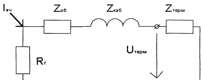
Рис. 5.4. Схема замещения для расчета синфазного напряжения на терминале при однофазном КЗ
