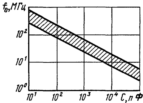
Рис. 4.10. Значения собственных резонансных частот f_0 помехоподавляющих конденсаторов в зависимости от их емкости C
