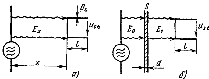
Рис. 3.26. Электромагнитное влияние на контур длиной l без экрана (а) и с экраном S толщиной d (б)
