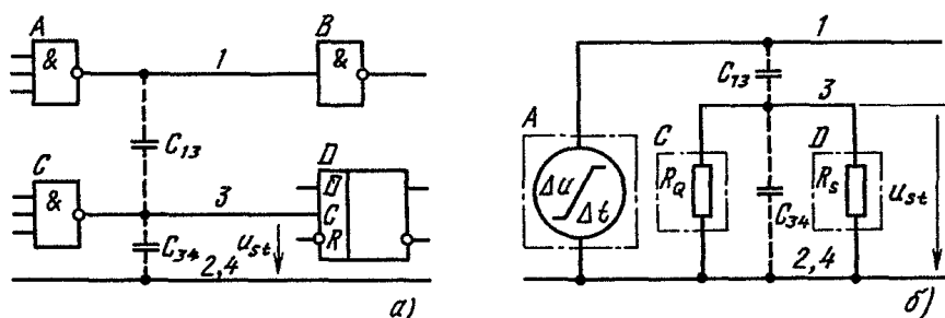
Рис. 3.13. Емкостное влияние контуров
