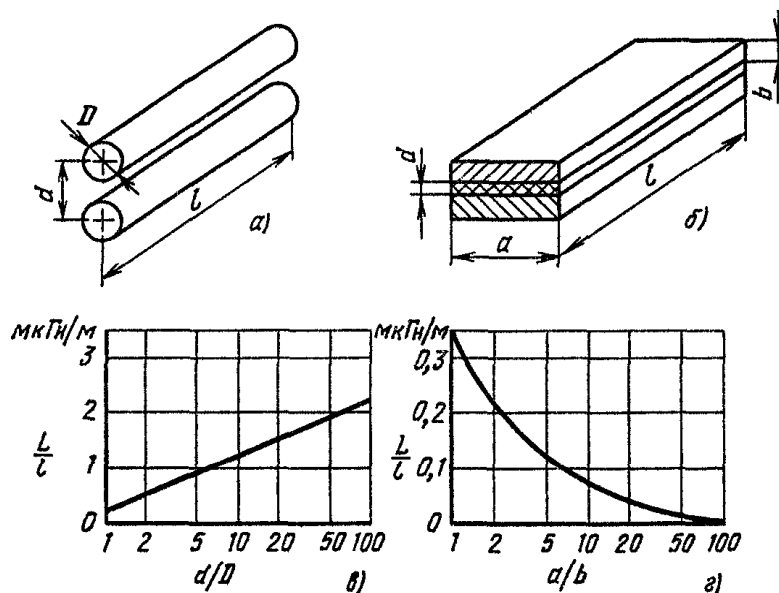
Рис. 3.5. Зависимости погонных индуктивностей ( \nu , \nu ) от соотношений размеров линий с проводами круглого (а) и прямоугольного (б) сечений
