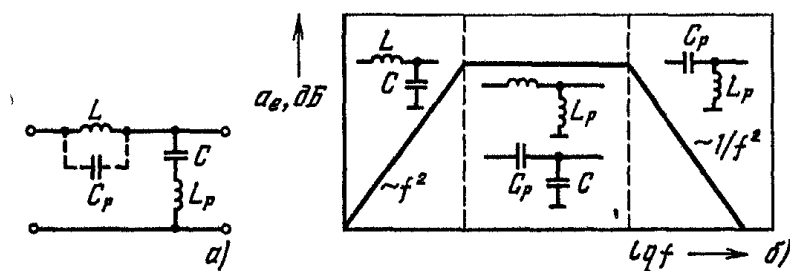
Рис. 4.12. Коэффициент затухания a_e фильтра LC:
