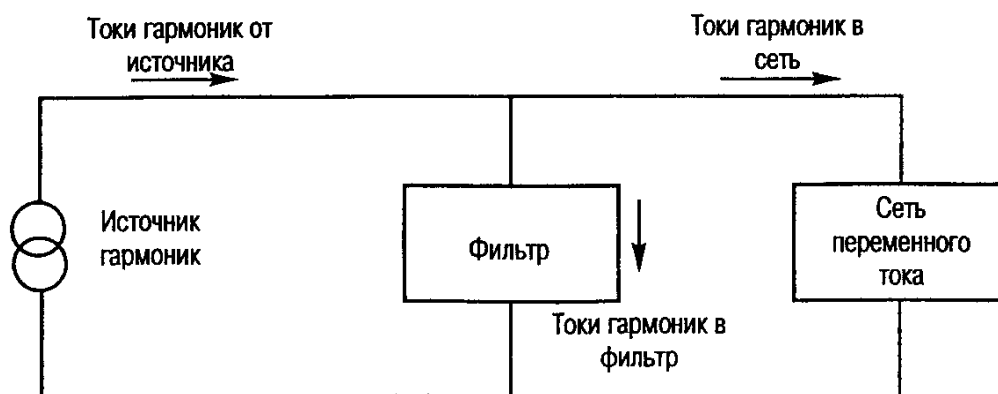
Рис. 6.5. Схема определения коэффициента искажения напряжения
