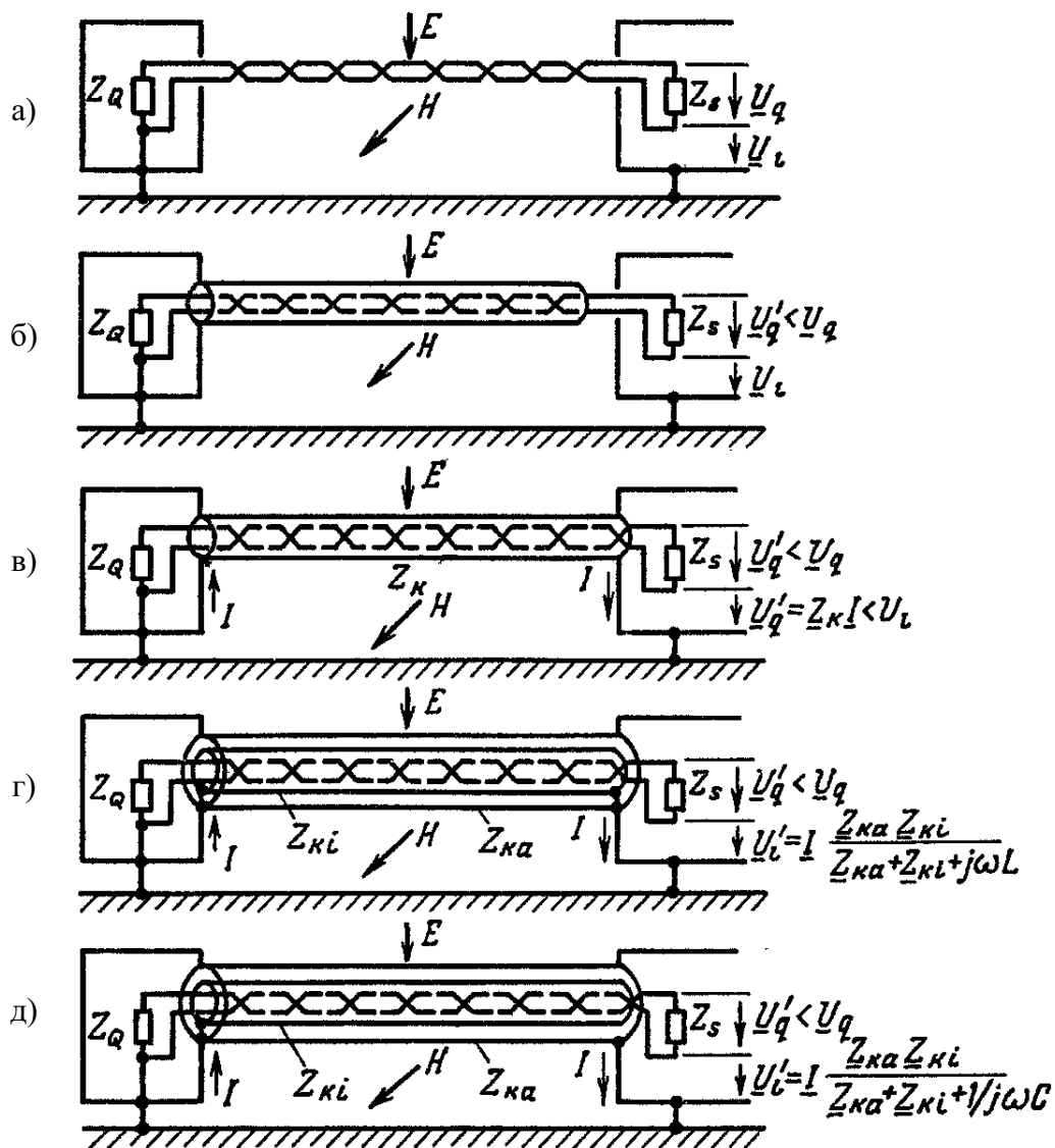
Рис. 4.26. Воздействие экранов кабелей:
