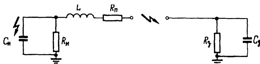
Рис. 2.5. Схема замещения цепи разряда заряженного тела человека или заряженного проводящего предмета: C_u , R_u – эквивалентные параметры замещения статически заряженного тела; R_n – последовательное сопротивление; C_3 , R_3 – емкость и сопротивление по отношению к земле объекта, через который происходит разряд или перезаряд
