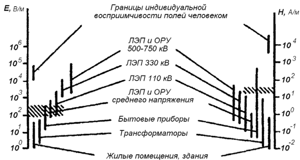
Рис. 7.1. Характерные напряженности электрических и магнитных полей промышленной частоты
