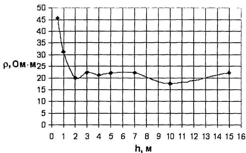
Рис. 5.1. Удельное сопротивление грунта
