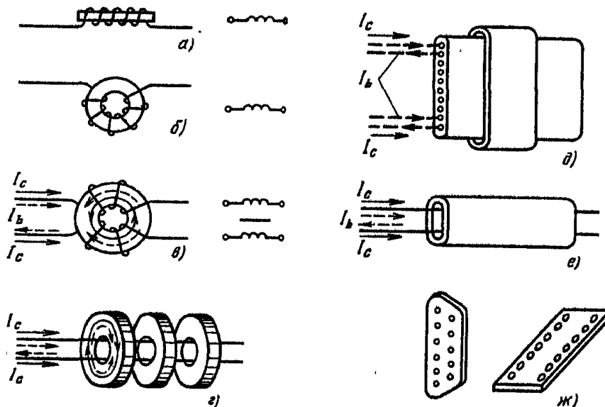
Рис. 4.7. Примеры выполнения помехозащитных катушек с рабочим током I_b , и синфазным током помехи I_c : а – стержневая катушка; б – простейшая катушка с кольцевым сердечником; в – кольцевая катушка с двумя встречными обмотками и компенсацией магнитного потока, создаваемого рабочим током I_b ; г – ферритовые кольца; д – ферритовые сердечники для плоских жгутов; е – линии с повышенным затуханием, с охватывающей оболочкой из материала с высоким затуханием; ж – ферритовые пластины с несколькими отверстиями для штекерных соединений и интегральных схем
