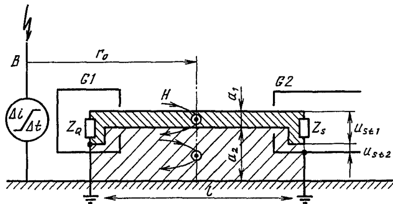
Рис. 3.24. Индуктивное влияние тока молнии на электрические контуры в устройстве автоматизации: B – канал молнии; G_1, G_2 – приборы устройства
