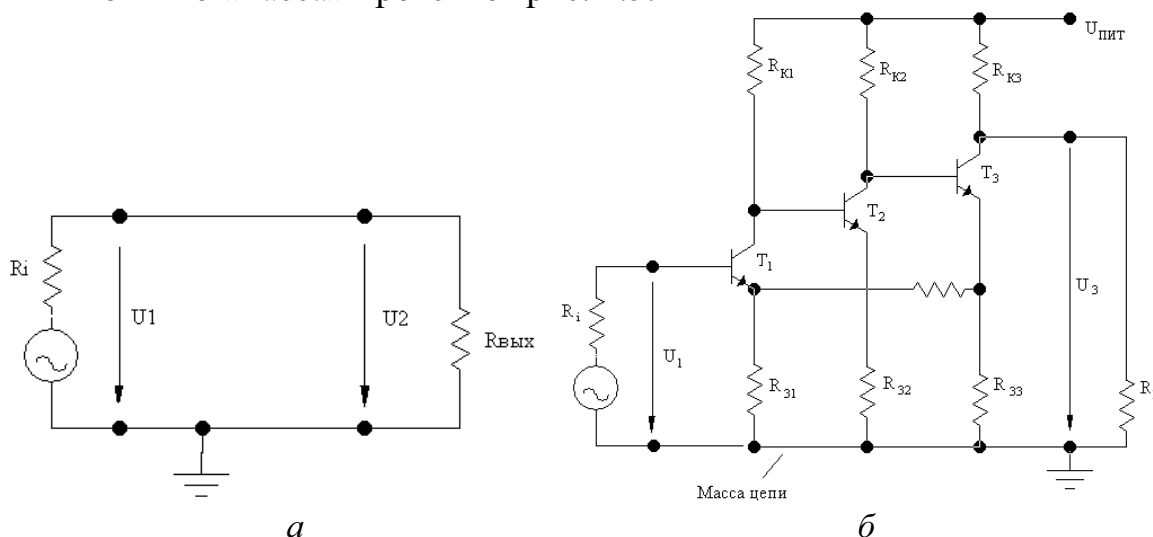
Рис. 1.5. Пояснение понятия «масса»
