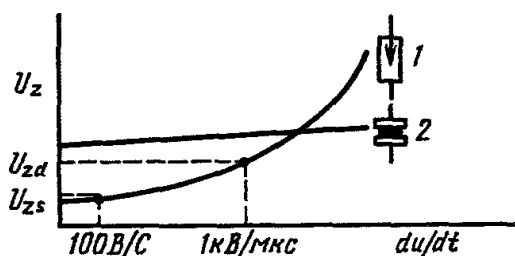
Рис. 4.18. Характеристики зажигания газонаполненного разрядника (1) и разрядника со скользящим разрядом (2) U_{zs} – статическое напряжение срабатывания; U_{zd} – динамическое напряжение срабатывания
