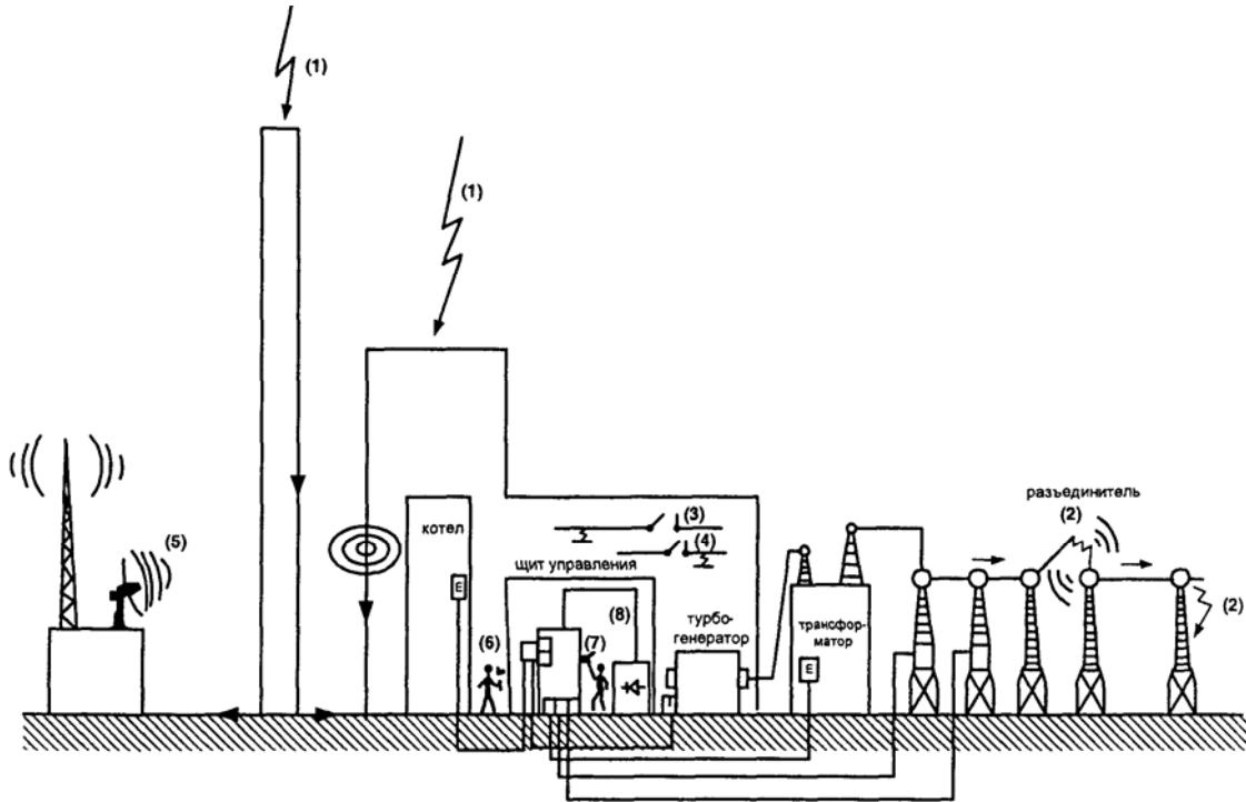
Рис. 1.1. Источники электромагнитных воздействий на электрических станциях и подстанциях: 1 – удар молнии; 2 – переключения и короткие замыкания (КЗ) в сети высокого напряжения; 3 – переключения и КЗ в сети среднего напряжения (СН); 4 – переключения и КЗ в сети низкого напряжения (НН); 5 – внешние источники радиочастотных излучений; 6 – внутренние источники радиочастотных излучений; 7 – разряды статического электричества; 8 – источники кондуктивных помех по цепям питания
