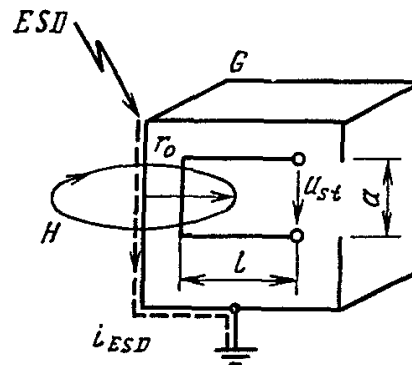
Рис. 3.23. Индуктивное влияние разряда статического электричества ESD на петлю l внутри прибора G
