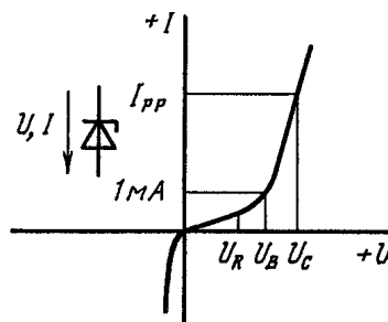
Рис. 4.22. Вольт-амперная характеристика стабилитрона и его важнейшие параметры
