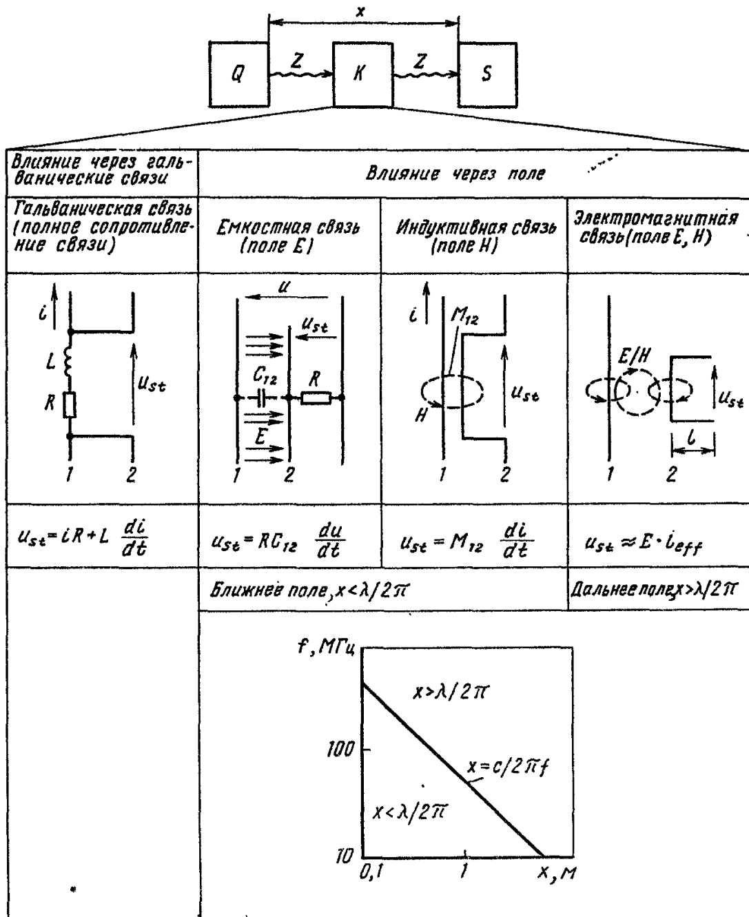
Рис. 3.1. Механизмы связи между контурами:
