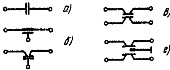
Рис. 4.6. Примеры выполнения помехозащитных конденсаторов: а – конденсатор с двумя выводами; б – конденсатор-ввод с тремя выводами; в – конденсатор-четырёхполюсник; г – многоэлементный конденсатор
