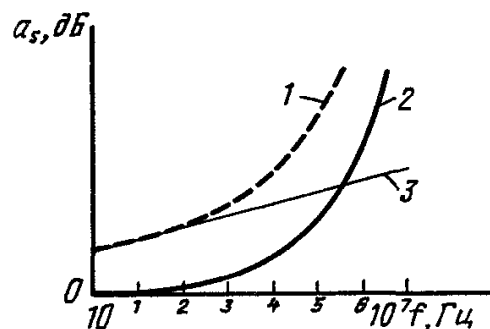
Рис. 4.24. Принципиальные зависимости коэффициентов: a_S = a_{SA} + a_{SR} (1), a_{SA} (2) и a_{SR} (3) от частоты f для магнитного поля в ближней зоне
