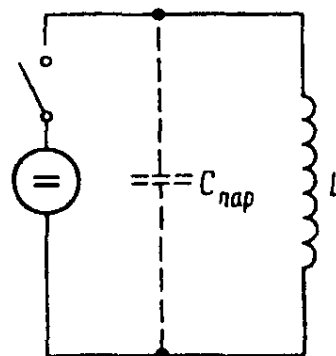
Рис. 2.7. Схема для приближенного определения максимального значения напряжения самоиндукции с учетом емкости катушки индуктивности
