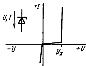
Рис. 4.21. Вольт-амперная характеристика Z-диода с напряжением U_g = 3 + 200 В
