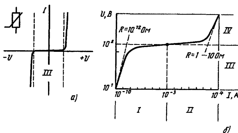
Рис. 4.20. Типичные вольт-амперные характеристики варисторов в линейных (а) и логарифмических (б) координатах: I – область токов утечек; II – область импульсных токов; III – диапазон рабочих напряжений; IV – область перенапряжений
