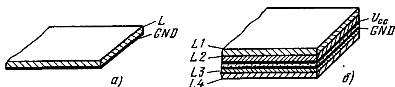
Рис. 3.6. Многослойные платы с плоскими шинами системы опорного потенциала GND (а) и шинами электропитания GND и U_{CC} (б):
