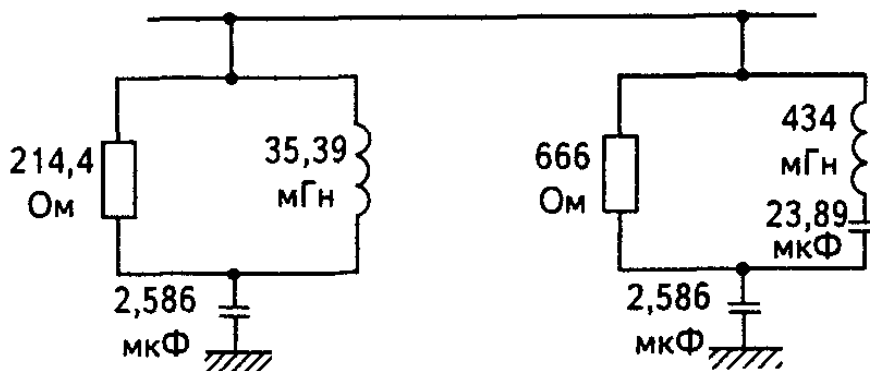
Рис. 6.9. Смешанный фильтр второго порядка и С-типа
