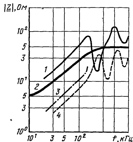
Рис. 4.4. Кажущееся сопротивление электроэнергетических сетей:
