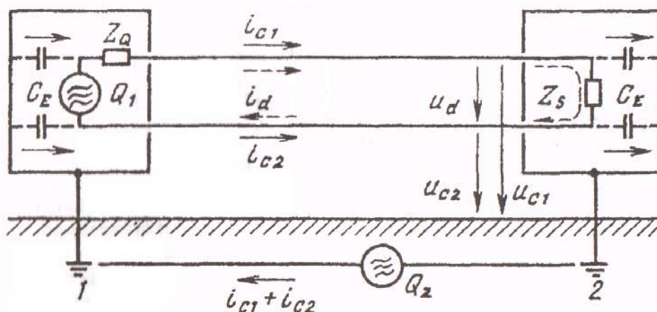
Рис. 1.3. Помехи, связанные с передачей сигналов по линии: C_E – паразитные емкости относительно заземленного корпуса; Q_1 – источник противофазных помех; Q_2 – источник синфазных помех; Z_Q, Z_S – полные сопротивления источника и приемника помех; i_{C1}, i_{C2} – синфазные токи, i_d – противофазный ток; u_{C1}, u_{C2} – синфазные напряжения помех; u_d – противофазное напряжение помех
