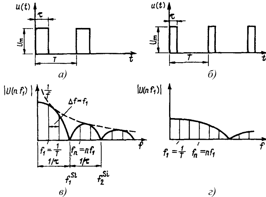
Рис. 1.10. Линейчатые спектры двух периодических последовательностей прямоугольных импульсов напряжений с личной скважностью (1:2): функция Si(x) – огибающая спектральных амплитуд (сплошная кривая); функция 1/f – огибающая функции Si(x) (пунктирная кривая)
