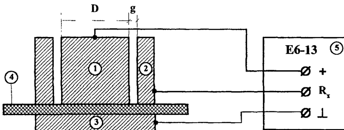
Рис. 5.6. Схема измерений поверхностного сопротивления полимерного диэлектрика:
