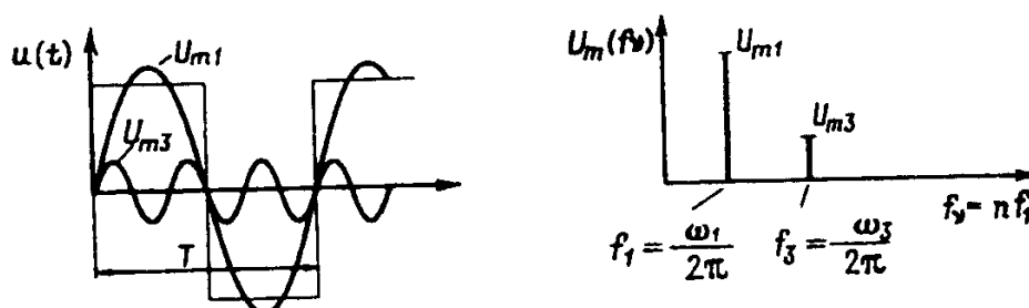
Рис. 1.8. Периодическая несинусоидальная функция
