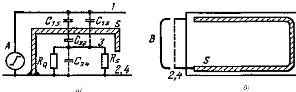
Рис. 3.17. Экранирующие дорожки на печатных платах: а – экранирующая дорожка S (схема замещения такая же, что и на рис. 3.16, б); б – короткозамкнутая дорожка (экран S с перемычкой B служит также защитой от индуктивного влияния)
