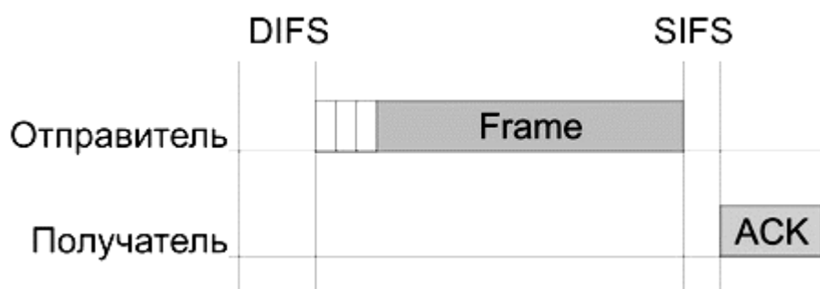
Рис. 61. Кадры квитанции, отсылаемые в случае успешной передачи данных
