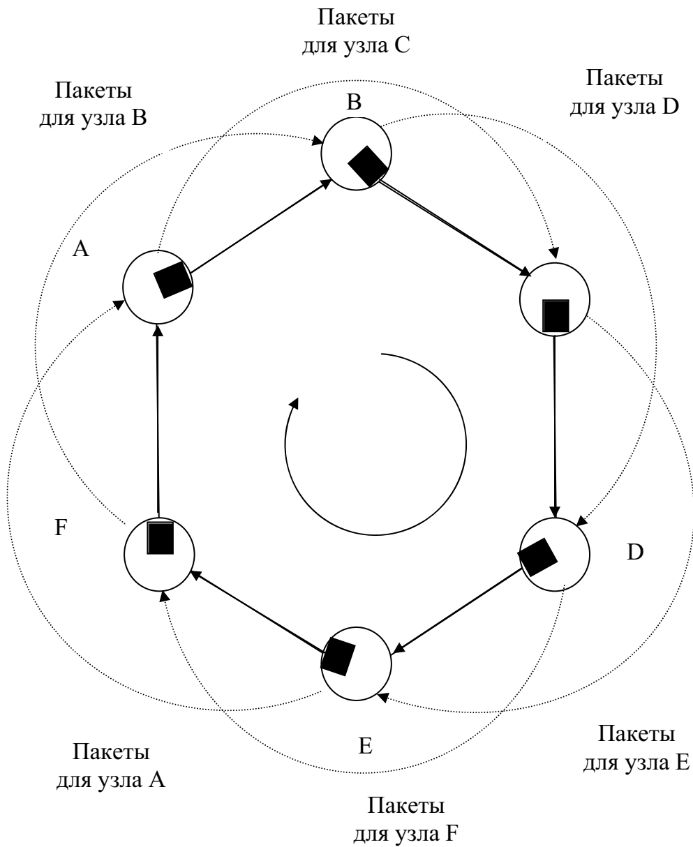
Рис. 15. Пример косвенной блокировки передачи
