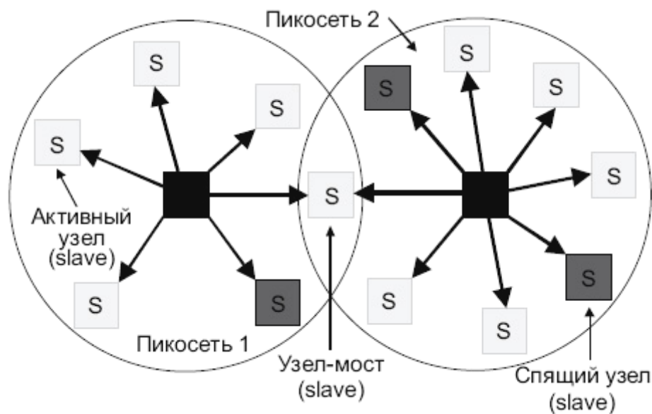
Рис. 68. Две пикосети, образующие рассеянную сеть
