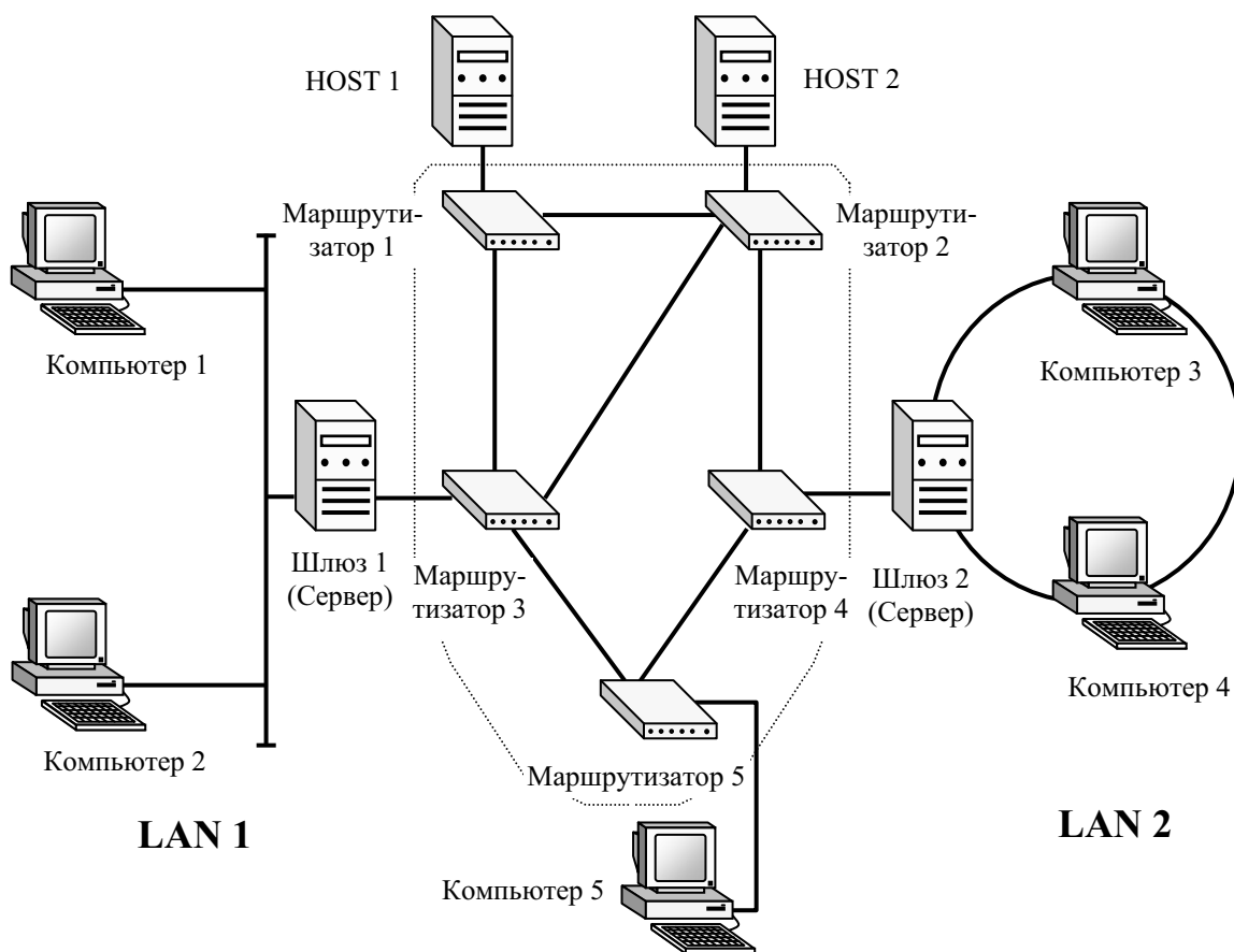
Рис. 4. Пример конфигурации компьютерной сети
