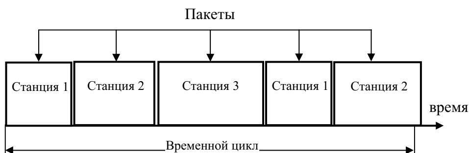
TDMA – Множественный доступ с временным разделением
