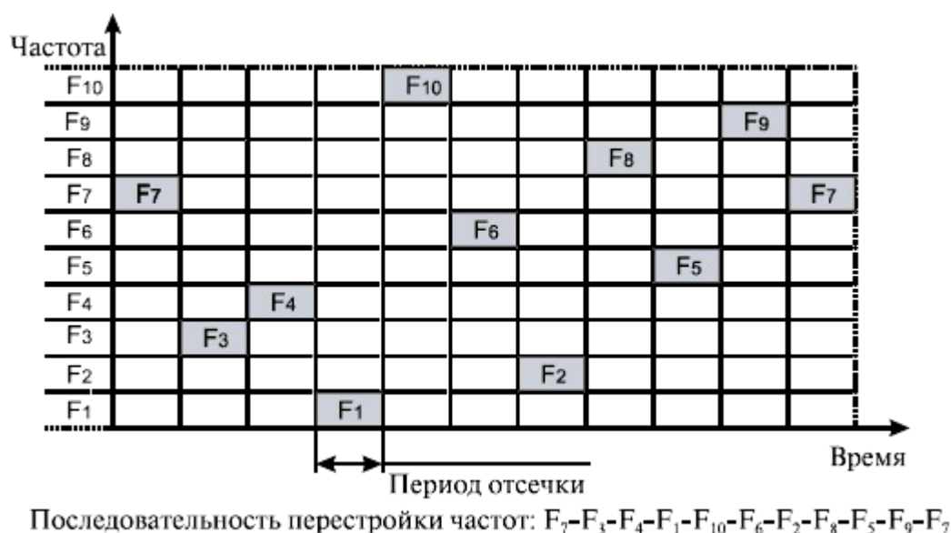
Рис. 55. Расширение спектра скачкообразной перестройкой частоты
