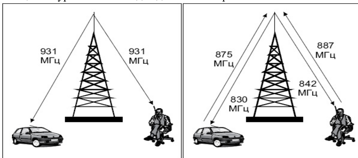
Рис. 71. Каналы пейджерной и мобильной телефонной сети
