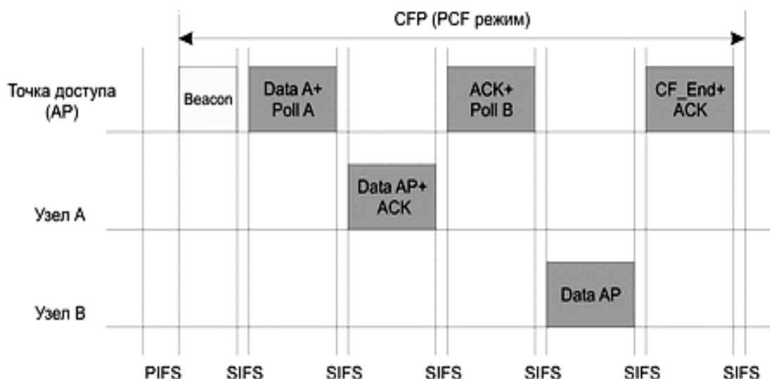
Рис. 67. Организация передачи данных между узлами сети в режиме PCF
