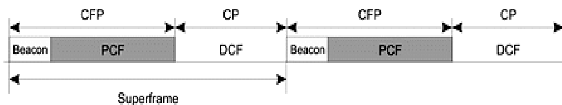
Рис. 66. Объединение режимов PCF и DCF в одном суперфрейме
