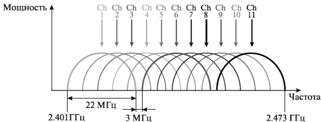
Рис. 56. Каналы, используемые в технологии DSSS
