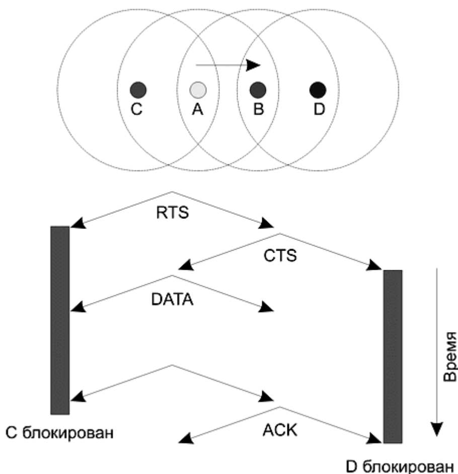
Рис. 63. Решение проблемы скрытых узлов в алгоритме RTS/CTS
