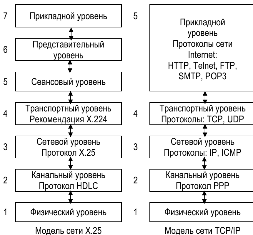
Рис. 44. Модели сетей X.25 и TCP/IP
