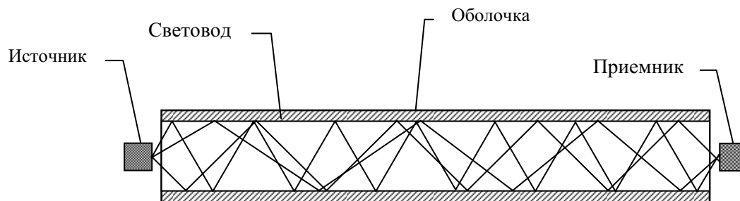
Рис. 7. Распространение света в многомодовом оптоволоконном световоде
