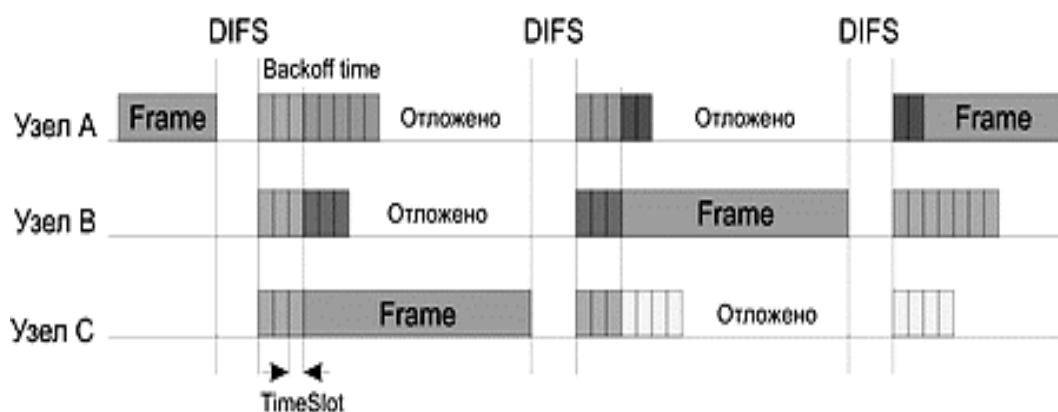
Рис. 60. Реализация равноправного доступа к среде передачи данных в методе DCF
