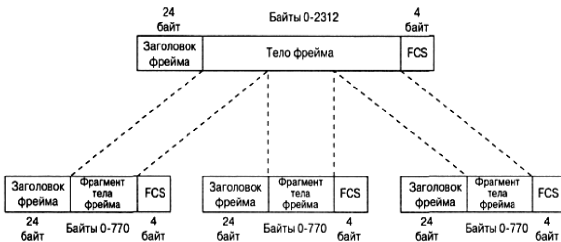
Рис. 65. Фрагментация фрейма
