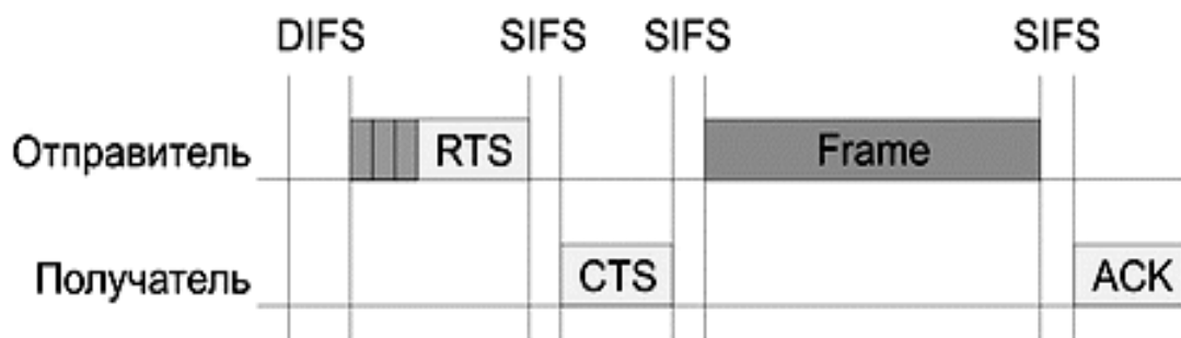
Рис. 62. Взаимодействие между двумя узлами сети в соответствии с алгоритмом RTS/CTS
