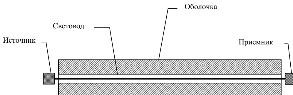
Рис. 6. Распространение света в одномодовом оптоволоконном световоде
