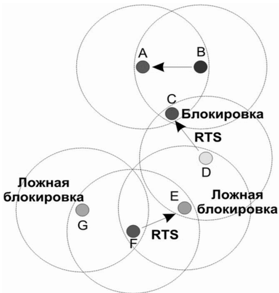
Рис. 64. Возникновение ложных блокировок узлов сети
