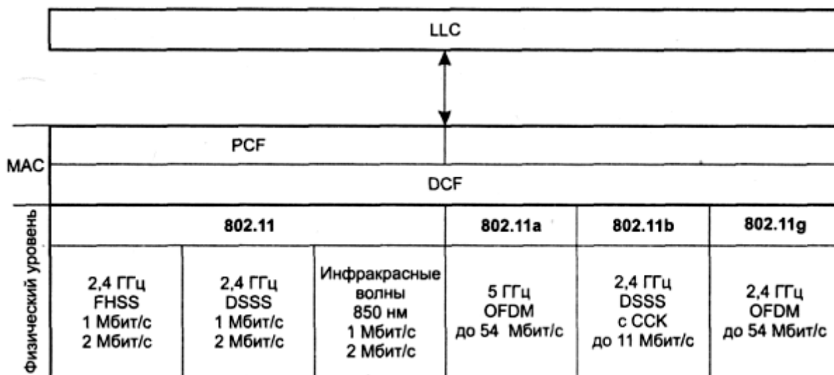
Рис. 54. Стек протоколов IEEE 802.11
