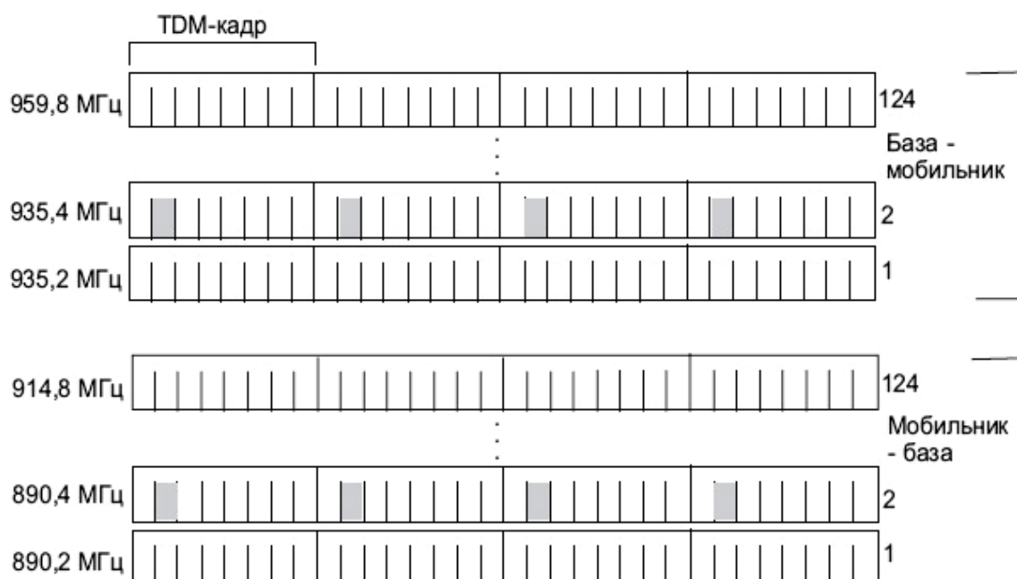
Рис. 72. Частотные каналы GSM
