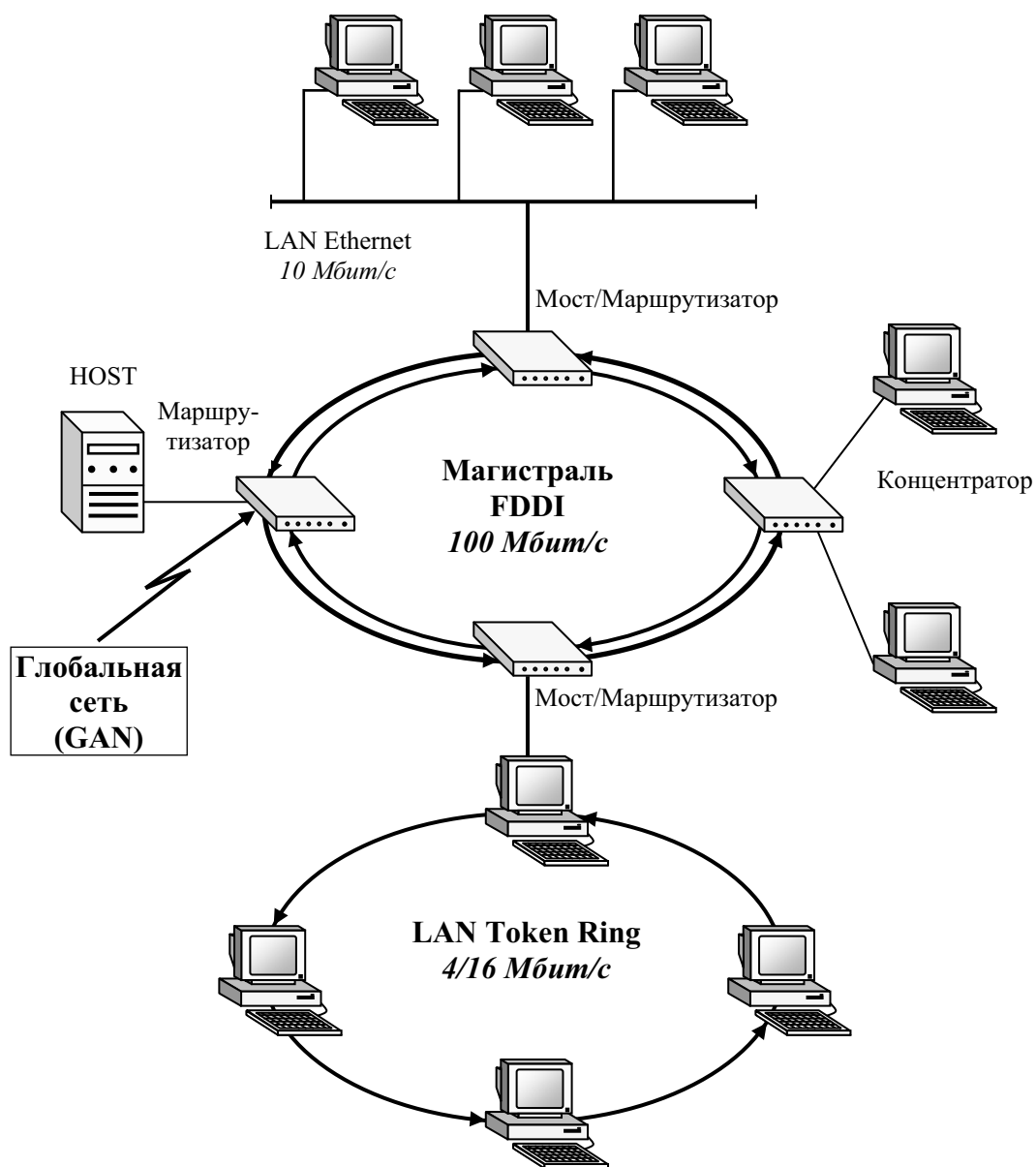
Рис. 37. Пример применения технологии FDDI для построения WAN
