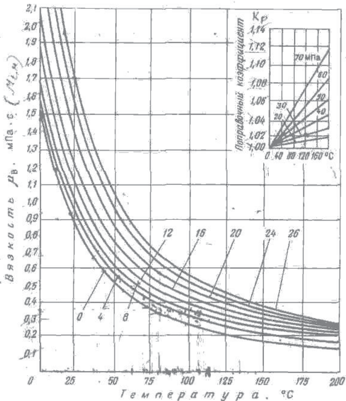
Зависимость вязкости воды \eta_{sp} от температуры при различных концентрациях NaCl. Шифр кривых — концентрация NaCl в г/100 г
