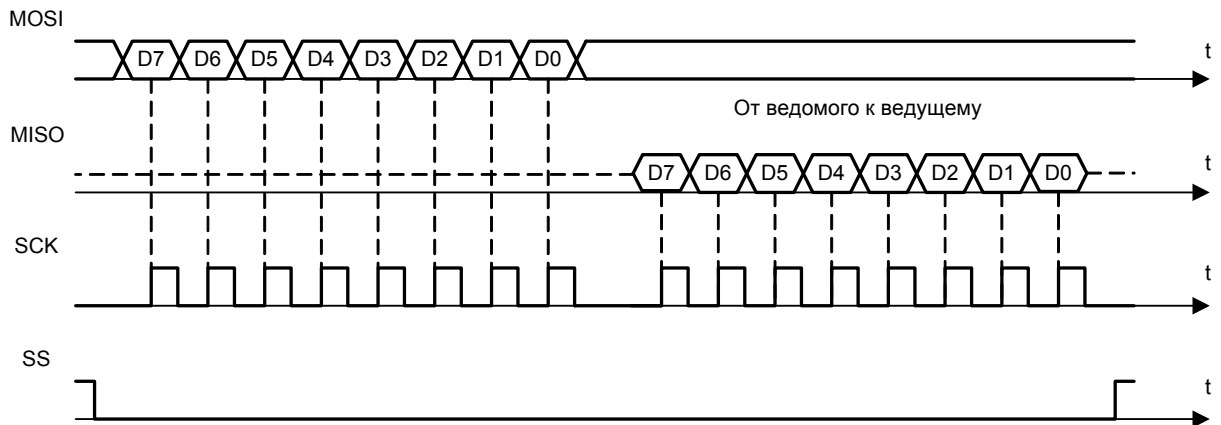
Рис. 13. Временные диаграммы, поясняющие принцип действия SPI-интерфейса.
