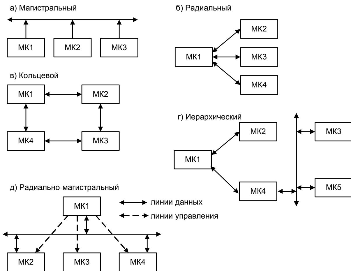
Рис. 2. Способы организации связи.
