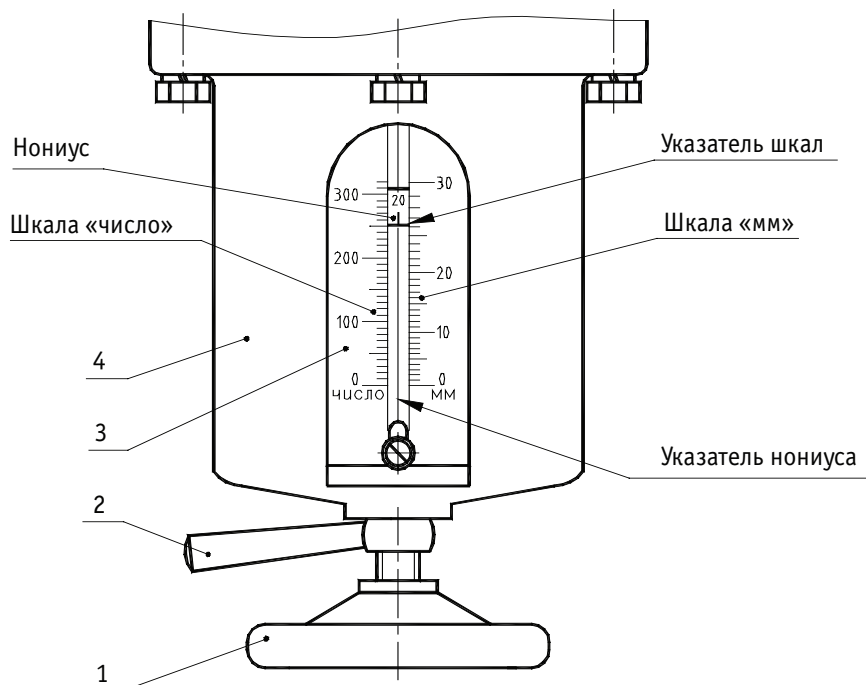
1 — маховичок; 2 — стопор; 3 — линейка; 4 — стакан передний
