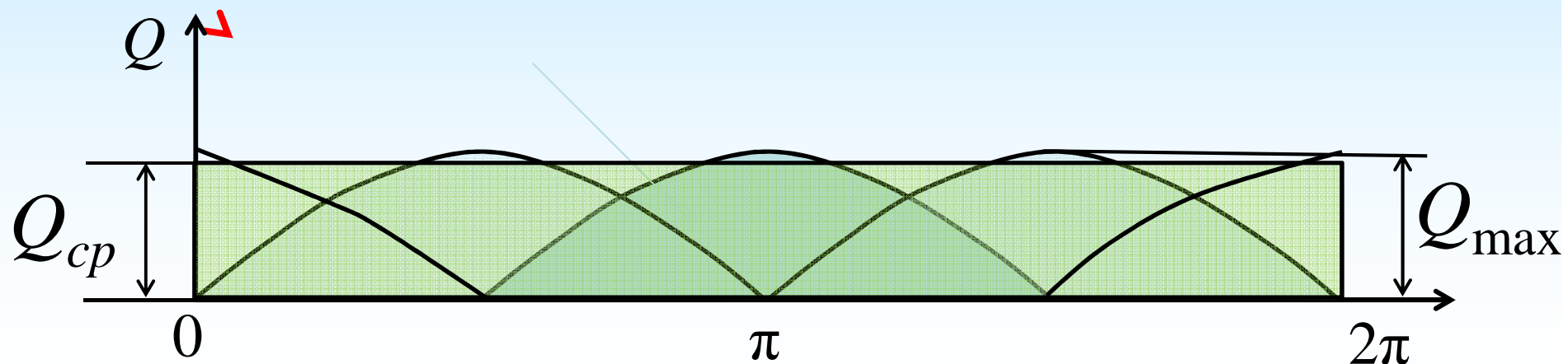
Трехцилиндровый насос одинарного действия
