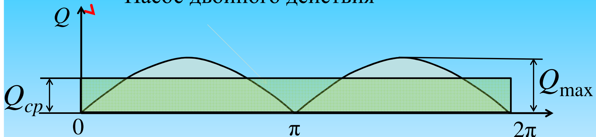
Насос двойного действия
