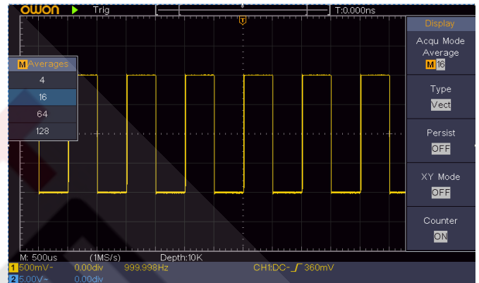
Рисунок 6.5. Подавление шума с помощью функции усреднения Average
