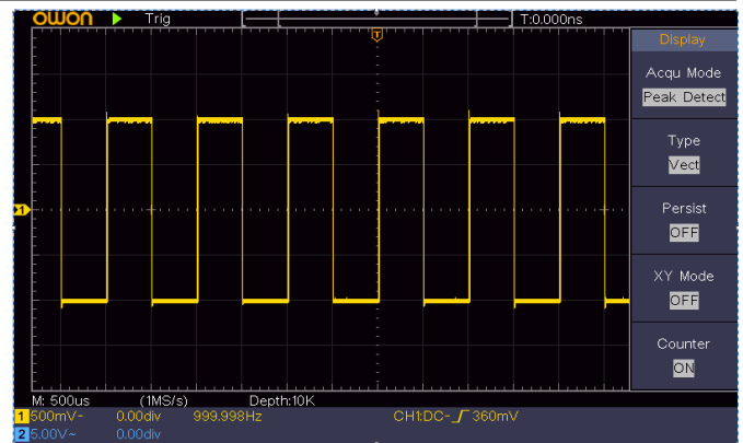
Рисунок 6.4. Сигнал, содержащий шум
