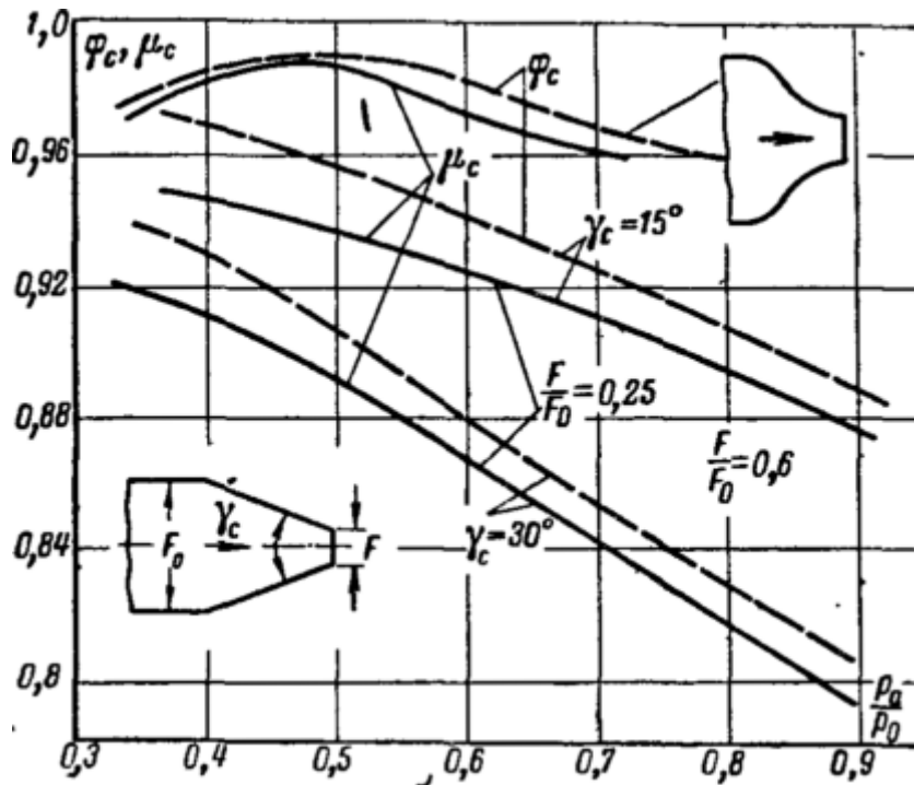
Рисунок 1. Коэффициенты скорости и расхода суживающегося сопла в зависимости от отношения давлений.
