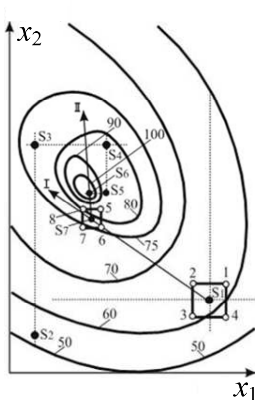
Рис. 8.3. Движение по поверхности отклика к экстремуму в традиционном эксперименте ( S_2 - S_3 - S_4 - S_5 - S_6 ) и в методе крутого восхождения ( S_1 - S_7 - S_6 )
