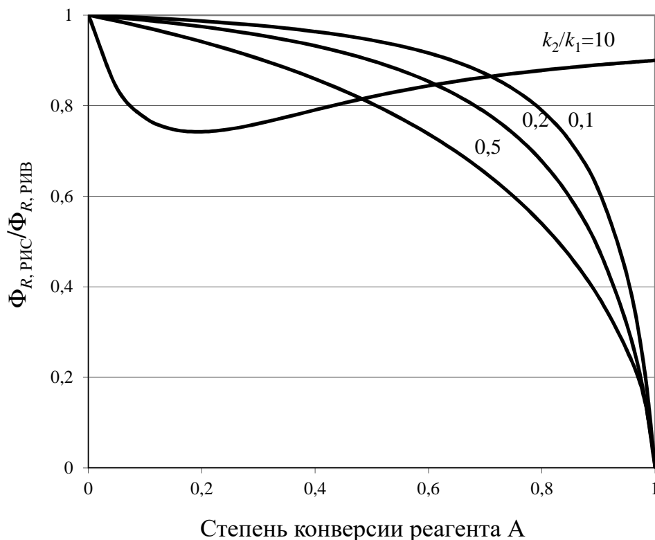
Рис. 4.31. Сравнительная эффективность реакторов полного смешения и идеального вытеснения по их селективности для последовательных реакций при разных степенях конверсии и соотношениях констант скорости
