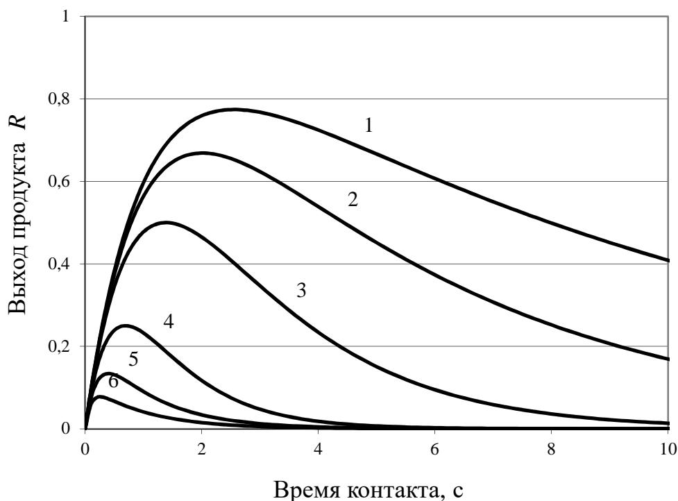
Рис. 4.28. Кинетические кривые накопления промежуточного продукта для последовательной реакции при различных отношениях констант скорости расходования ( k_2 ) и образования ( k_1 = 1,0 \text{ с}^{-1} ) k_2/k_1 = : 1 – 0,1; 2 – 0,2; 3 – 0,5; 4 – 2,0; 5 – 5,0; 6 – 10,0
