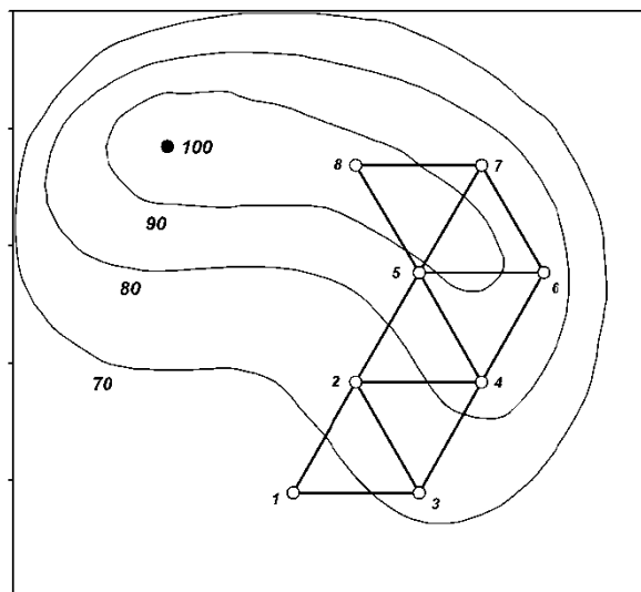
Рис. 8.1. Оптимизация по симплексному методу
