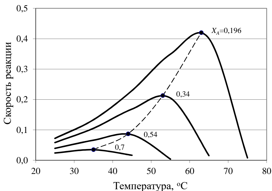
Рис. 3.12. Зависимость скорости обратимой экзотермической реакции от температуры при разной степени конверсии
