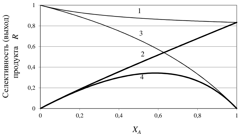
Рис. 4.16. Зависимость селективности и выхода целевого продукта от степени конверсии для сложного последовательного процесса с обратимой реакцией ( K_2=0,2 ) образования побочного продукта (кривые 1, 2; k_1:k_2:k_{.2}=2:1:5 ) и сложной последовательной необратимой реакции (кривые 3, 4; k_1:k_2=2:1 )
