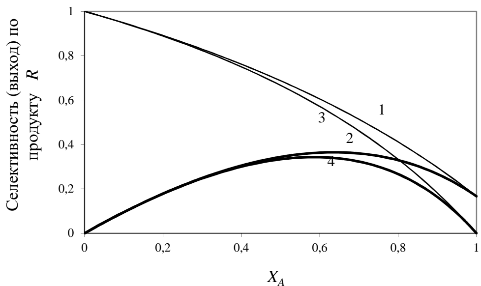
Рис. 4.16. Зависимость селективности и выхода целевого продукта от степени конверсии для сложного последовательного процесса с обратимой реакцией ( K_2=0,2 ) образования побочного продукта (кривые 1, 2; k_1:k_2:k_{.2}=2:1:5 ) и сложной последовательной необратимой реакции (кривые 3, 4; k_1:k_2=2:1 )
