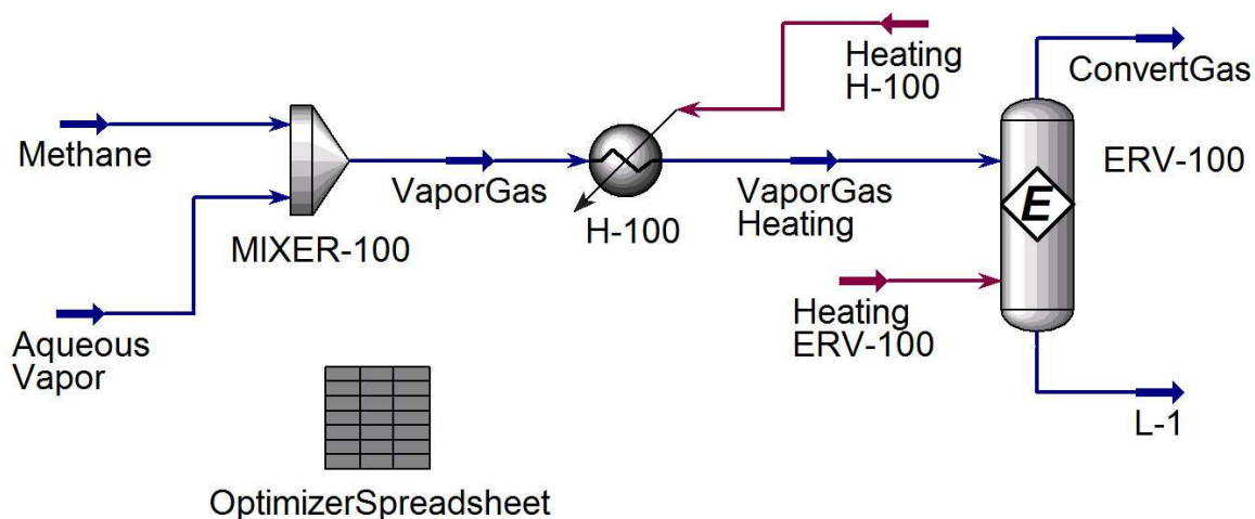
Рис. 7.1. Технологическая схема конверсии метана водяным паром
