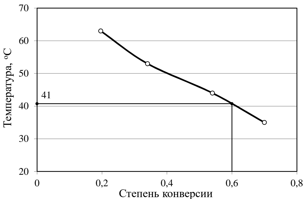
Рис. 3.13. Оптимальный профиль температур для обратимой экзотермической реакции
