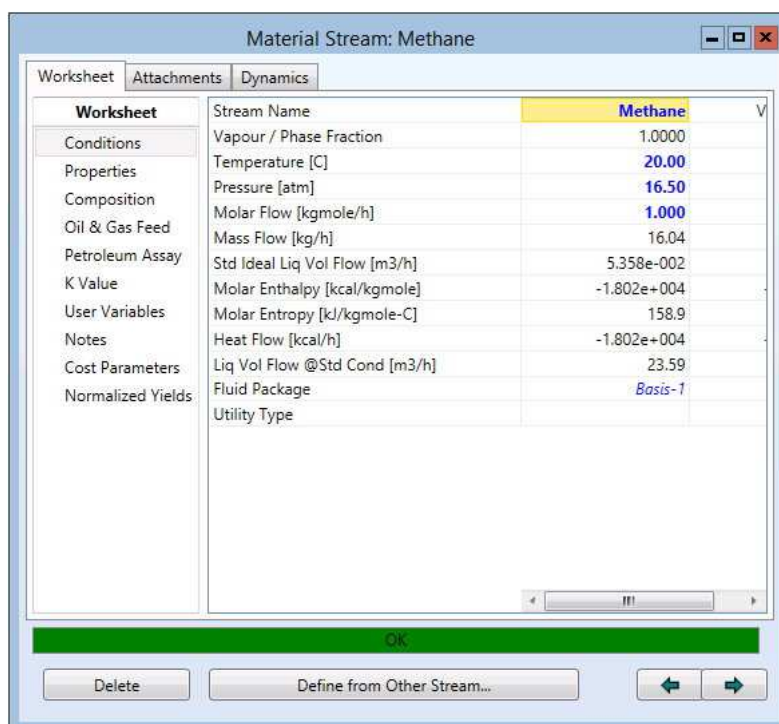
Рис. 7.17. Специализированное окно «Material Stream: Methane»
