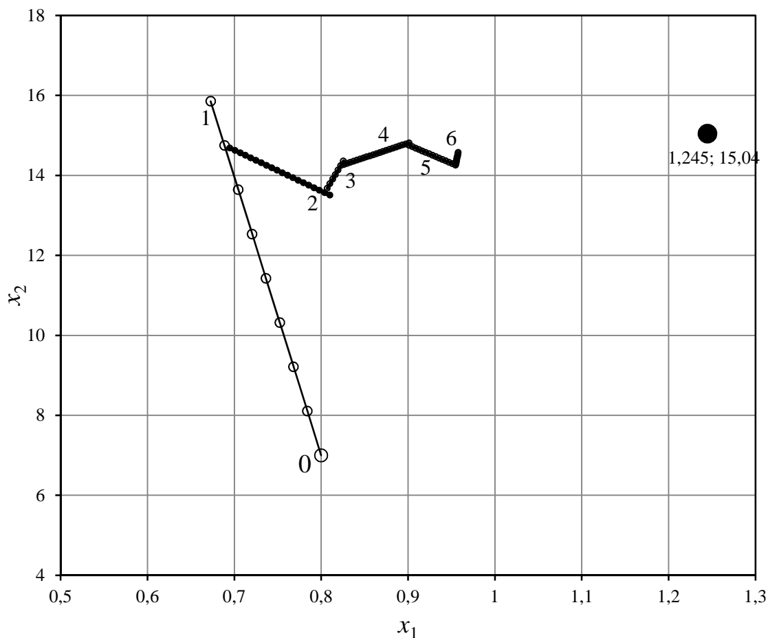
Рис. 8.4. Результаты поиска оптимальных условий проведения процесса методом наискорейшего спуска. 0 – исходная точка; 1, 2, 3, 4, 5, 6 – этапы (направления) продвижения
