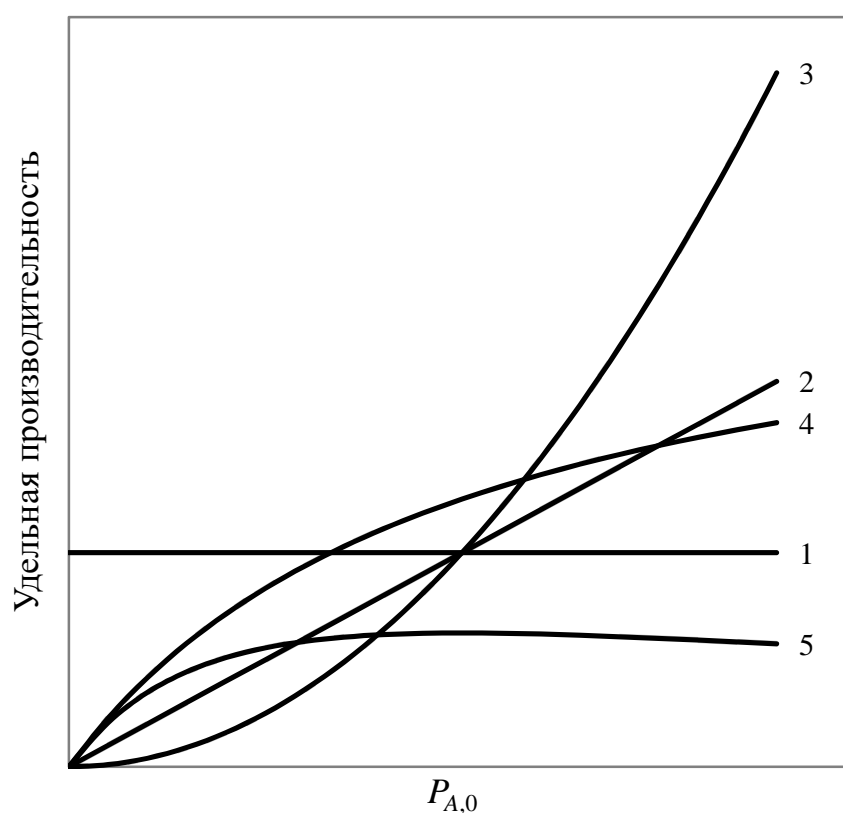
Рис. 3.10. Зависимость удельной производительности реакторов от начального парциального давления (концентрации) основного реагента при прочих равных условиях для реакции нулевого (1), первого (2) и второго (3) порядка, а также для реакций с кинетическим уравнением r = k' \cdot P_A / (1 + b_A P_A) (4) и для реакций с кинетическим уравнением r = k' \cdot P_A / (1 + b_A P_A)^2 (5)
