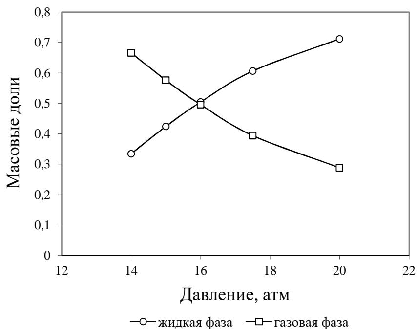
Рис. 5.10. Относительное количество жидкой и газовой фаз при 600 К
