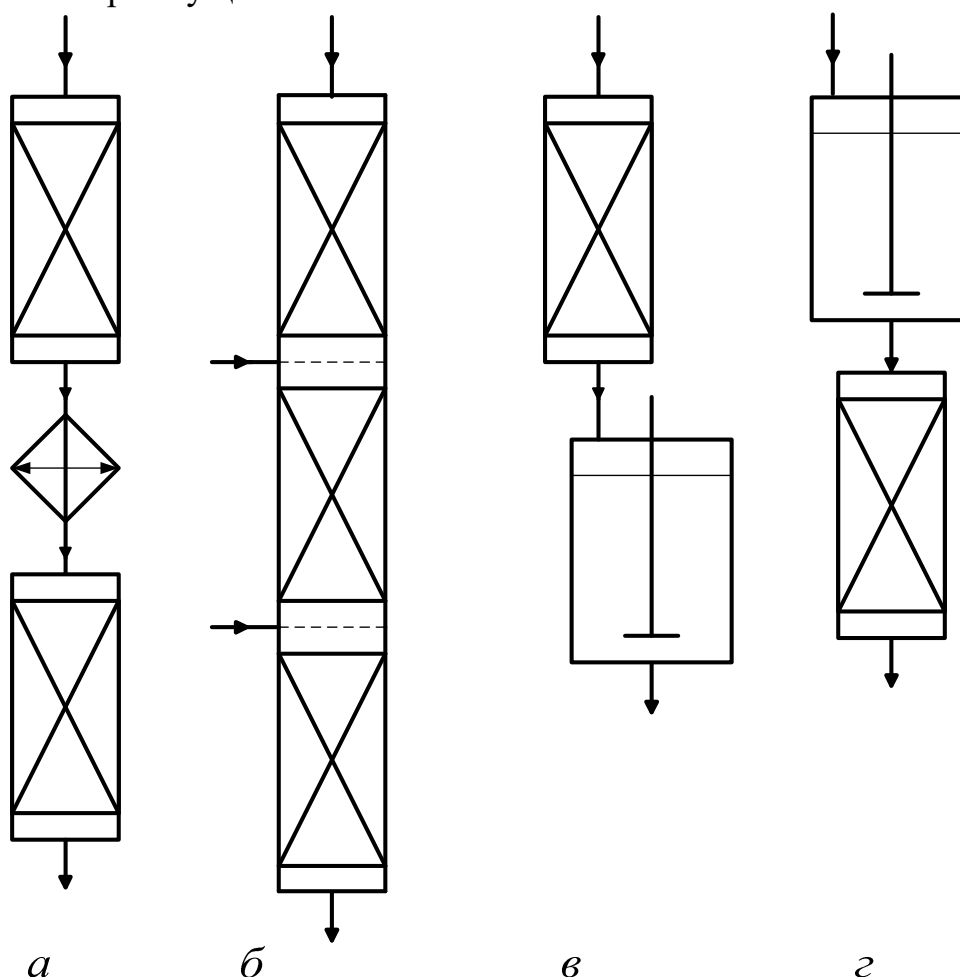
Рис. 3.8. Сочетание реакторов:
