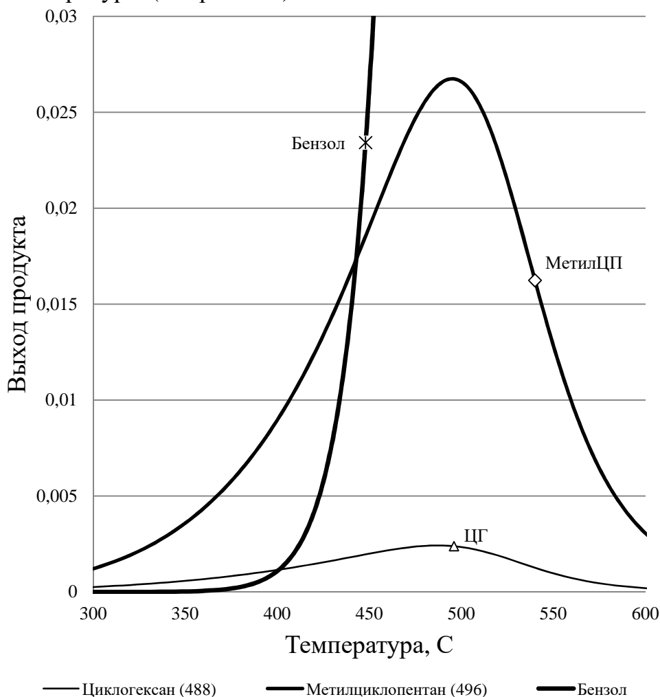
Рис. 5.5. Зависимость выхода продуктов реакции риформинга от температуры
