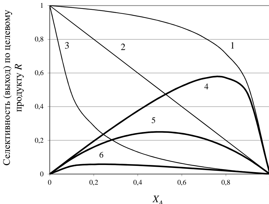
Рис. 4.6. Зависимость селективности (1,2,3) и выхода (4,5,6) по промежуточному продукту последовательных реакций от степени конверсии в реакторе полного смешения при k_2/k_1=0,1 (1,4), k_2/k_1=1,0 (2,5) и k_2/k_1=10 (3,6)
