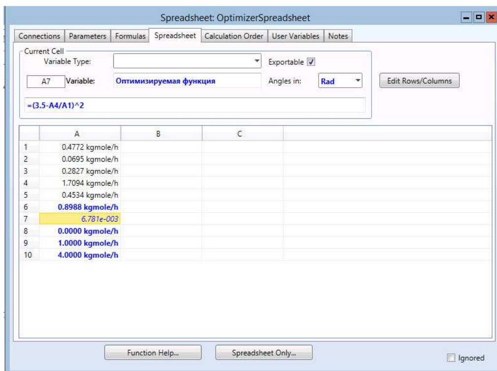
Рис. 7.32. Электронная таблица Оптимизатора, закладка «Spreadsheet»
