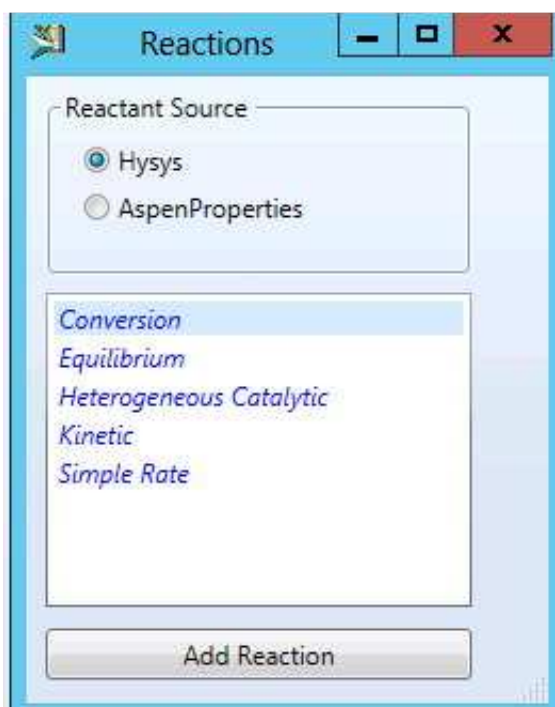
Рис. 7.7. Окно выбора типа реакций « Reactions »
