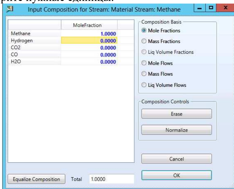
Рис. 7.16. Специализированное окно «Input Composition for Stream» после нормализации
