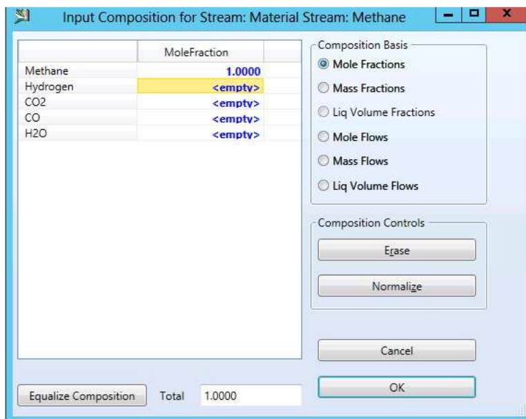
Рис. 7.15. Специализированное окно « Input Composition for Stream »
