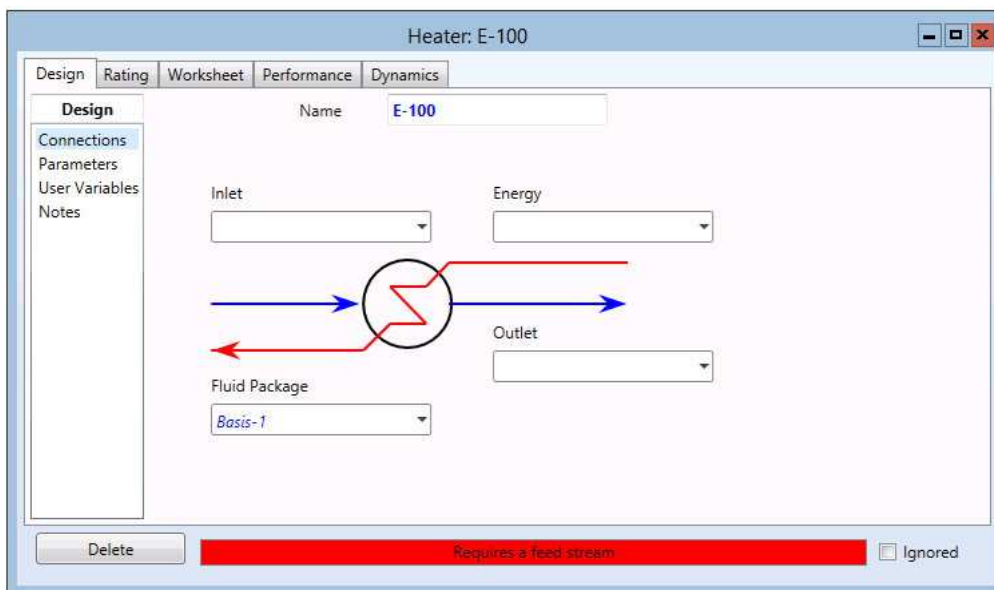
Рис. 7.21. Окно операции Подогреватель «Heater», страница «Design»
