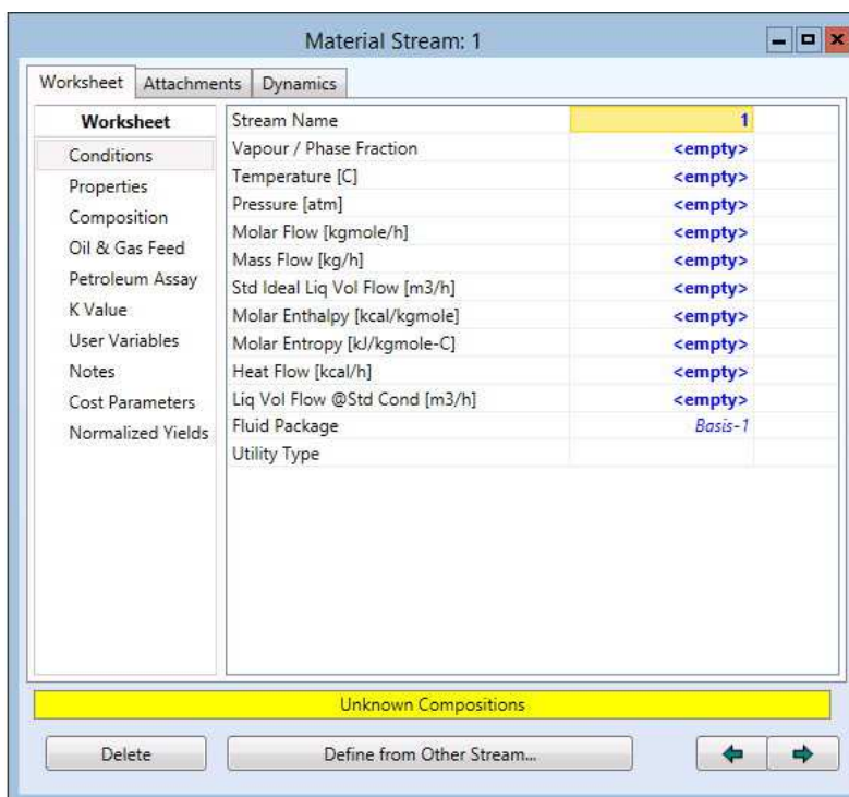
Рис. 7.14. Специализированное окно « Material Stream 1 »
