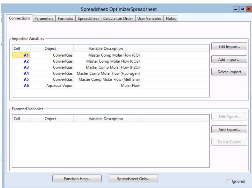
Рис. 7.31. Электронная таблица Оптимизатора, закладка «Connections»
