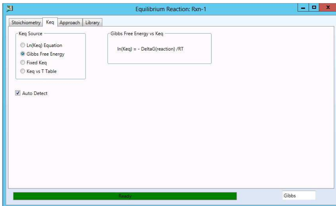
Рис. 7.9. Дочернее окно « Equilibrium Reaction: Rxn-1 », лист « КЕq »
