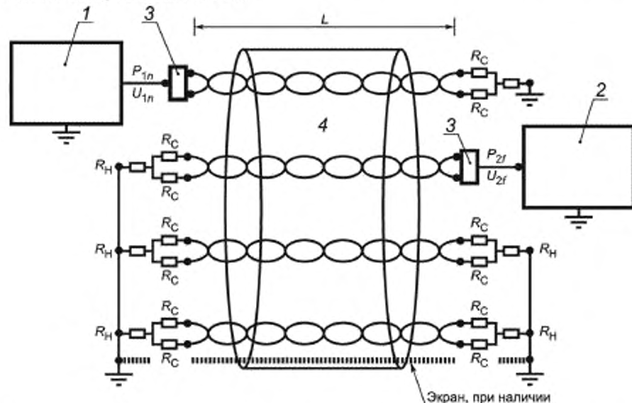
1 — анализатор цепей или генератор сигналов; 2 — анализатор цепей или измерительный приемник; 3 — симметрирующий трансформатор; 4 — измеряемый кабель; R_C и R_N — нагрузки симметричной и несимметричной цепей соответственно; L — длина измеряемого кабеля; P_{1n}(U_{1n}) — мощность (напряжение) сигнала на ближнем конце влияющей пары; P_{2f}(U_{2f}) — мощность (напряжение) сигнала на дальнем конце подверженной влиянию пары
