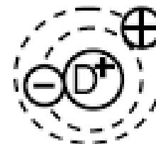
связанный экситон (на доноре)
