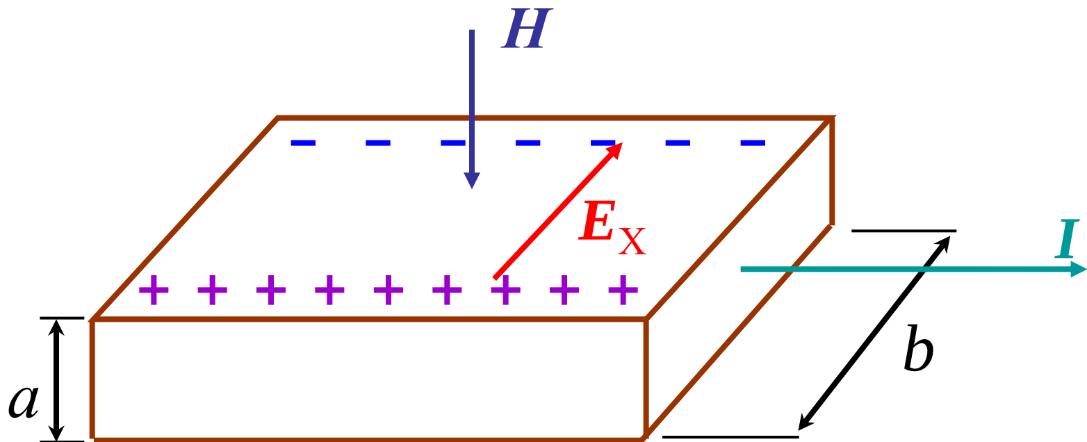
Схема возникновения ЭДС Холла U_x
