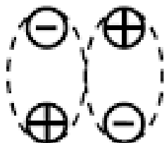
бизекситон (экситонная молекула)
