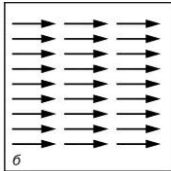
Ферромагнитное вещество — атомные магниты упорядочены
