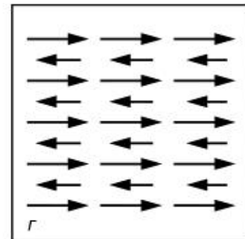
Ферримагнитное вещество — нескомпенсированная антипараллельная ориентация
