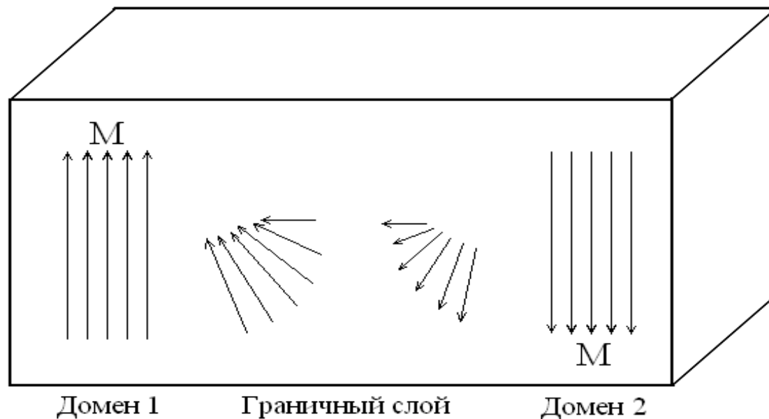
Магнитная структура граничного слоя в кристалле
