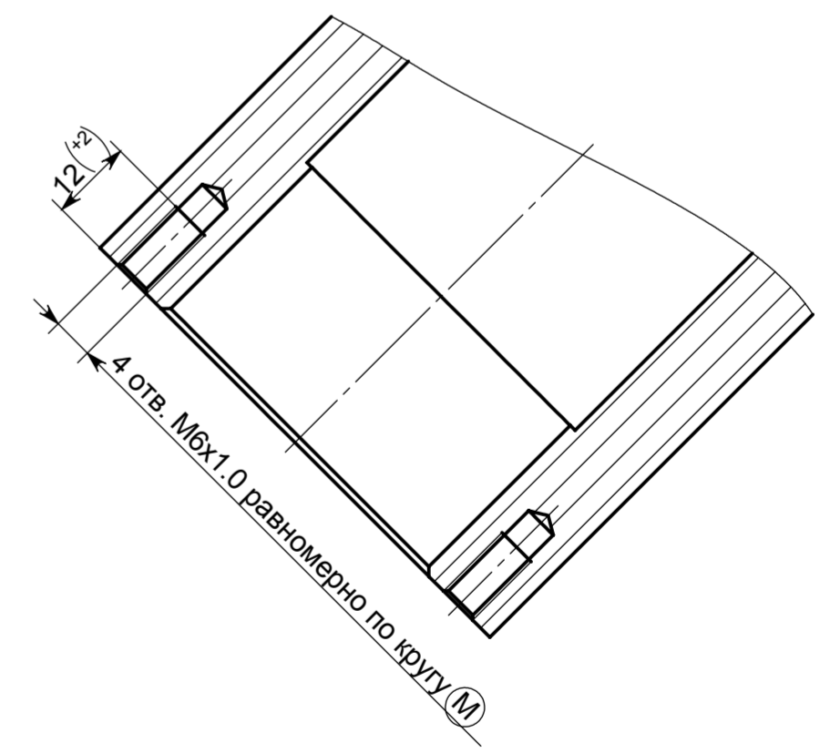
СЕЧЕНИЕ И-И
