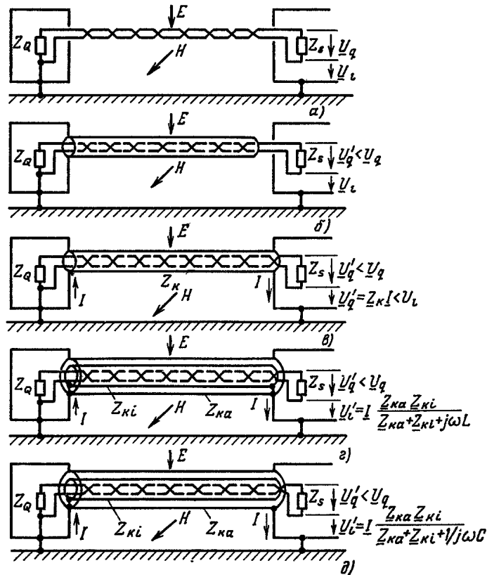
Рис. 4.26. Воздействие экранов кабелей:
