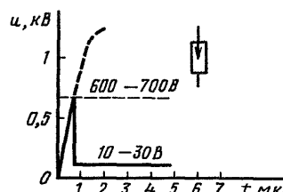
Рис. 4.19. Типичная характеристика зажигания газонаполненного разрядника
