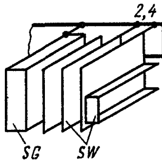
Рис. 3.18. Экранирование функциональных блоков печатных плат перегородками SW или функциональных модулей коробками SG : 2, 4 — пластина опорного потенциала
