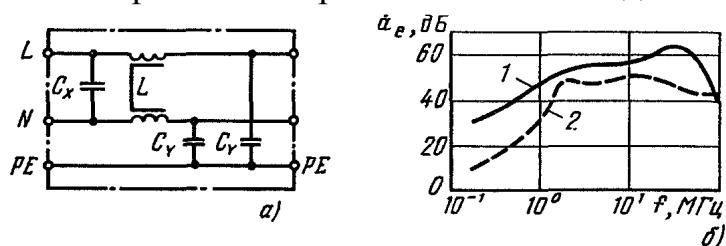
Рис. 4.14. Пример сетевого фильтра на 250 В, 1 А:
