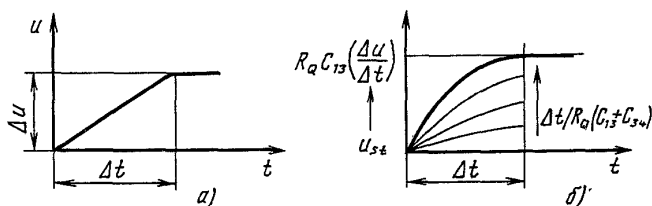
Рис. 3.14. Выходной сигнал элемента A на рис. 3.13, а (а) и сигнал помехи u_{st} в интервале времени 0 \leq t \leq \Delta t (б)
