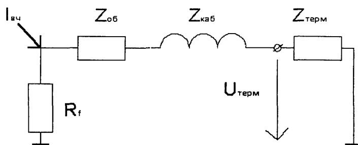
Рис. 5.4. Схема замещения для расчета синфазного напряжения на терминале при однофазном КЗ на шинах ВН энергообъекта:
