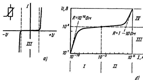
Рис. 4.20. Типичные вольт-амперные характеристики варисторов в линейных (а) и логарифмических (б) координатах:
