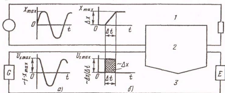
Рис. 1.6. Пояснение параметров периодических (а) и непериодических переходных (б) помех: E – приемник сигналов; G – источник сигналов; x – помеха (напряжение или ток); u_s – напряжение помехи, обусловленное связью; 1 – влияющий контур; 2 – гальваническая, емкостная или индуктивная связь; 3 – контур, подверженный влиянию
