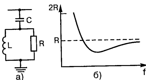
Рис. 6.4. Схема параллельного фильтра второго порядка подавления частот (а) и зависимость его полного сопротивления R от частоты (б)
