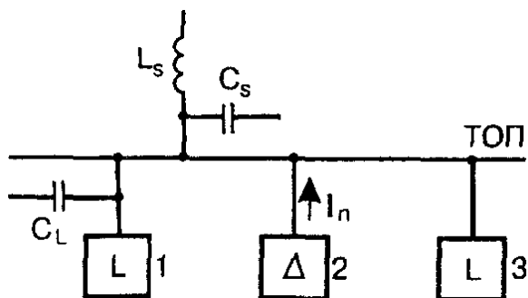
Рис 6.1. Параллельный резонанс: 1,3 – нагрузки; 2- источник гармоник; ТОП – точка общего присоединения.
