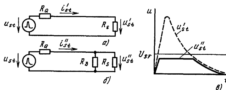
Рис. 4.16. Ограничение перенапряжений при помощи нелинейного сопротивления R_B : а - схема без защиты; б - схема с защитой; в - изменение напряжений во времени; U_{SF} — импульсная прочность входной цепи
