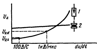
Рис. 4.18. Характеристики зажигания газонаполненного разрядника (1) и разрядника со скользящим разрядом (2):
