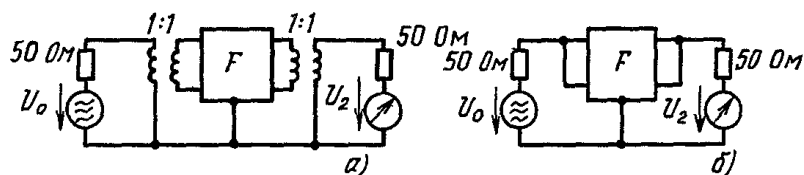
Рис. 4.5. Схемы для измерений симметричного (а) и асимметричного коэффициентов затуханий (б) a_e фильтров:
