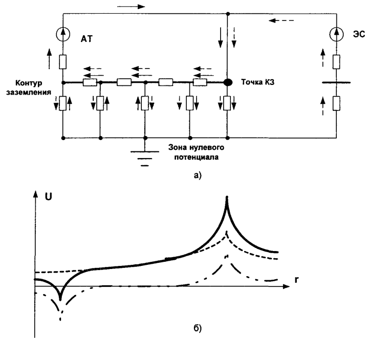
Рис 5.2. Однофазное короткое замыкание на шинах ПС высокого напряжения:
