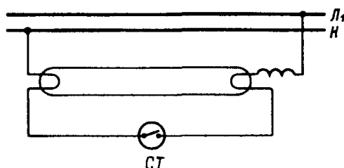
Рис. 2.4. Низковольтная люминесцентная лампа с катушкой индуктивности ограничения тока и стартером тлеющего разряда СТ
