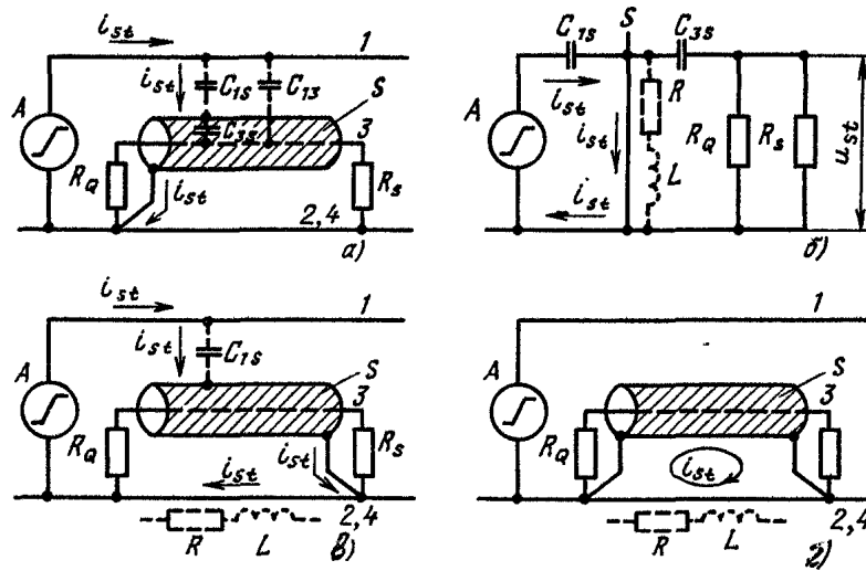
Рис. 3.16. Экранирование линии:
