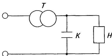
Рис. 6.2. Схема последовательного резонанса K – конденсатор, T – трансформатор, H – активная нагрузка
