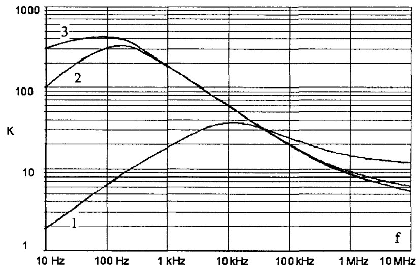
Рис. 5.5. Расчетные коэффициенты экранирования: 1 - экранированный кабель, 2 - стальной короб, 3 - кабельный канал
