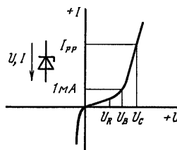
Рис. 4.22. Вольт-амперная характеристика стабилизатора и его важнейшие параметры
