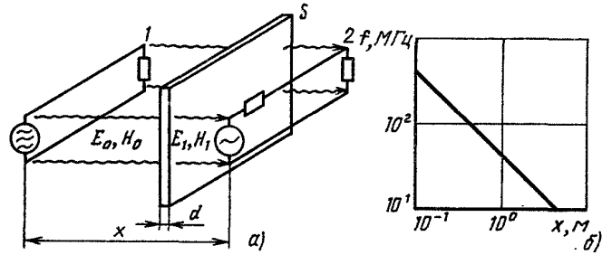
Рис. 4.23. Экранирование токовых контуров от внешних электрических и магнитных полей: а - принципиальное расположение контуров 1, 2 и экрана S; б - граница между условиями ближнего (нижняя левая часть) и дальнего (верхняя правая часть) полей
