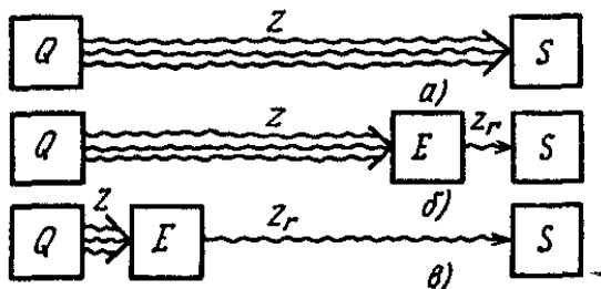
Рис. 4.1. Взаимные расположения источника помех Q , приемника S и защитного компонента E :
