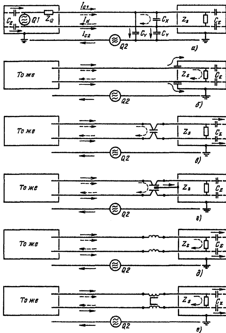
Рис. 4.8. Защита катушками индуктивности и конденсаторами от синфазных и противофазных токов помех (пояснения см. в тексте):
