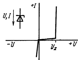
Рис. 4.21. Вольт-амперная характеристика Z-диода с напряжением U_Z = 3 + 200 \text{ В}
