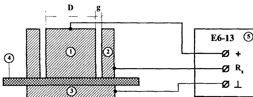
Рис. 5.6. Схема измерений поверхностного сопротивления полимерного диэлектрика:
