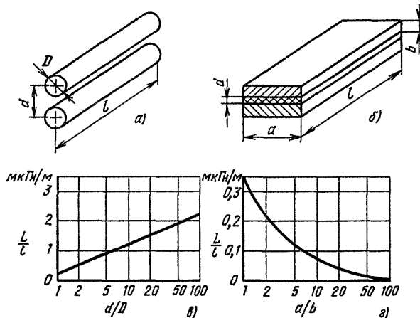
Рис. 3.5. Зависимости погонных индуктивностей (в, г) от соотношений размеров линий с проводами круглого (а) и прямоугольного (б) сечений
