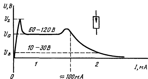
Рис. 4.17. Вольт-амперная характеристика газонаполненного разрядника с ориентировочными значениями напряжений тлеющего ( U_G ) и дугового ( U_B ) разрядов; U_Z - напряжение зажигания (см. рис. 4.18); 1 - область начальных и тлеющих разрядов; 2 - область дуговых разрядов
