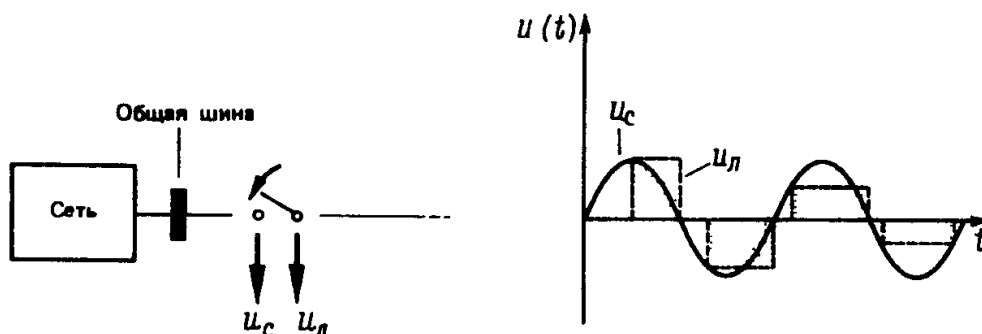
Рис. 2.8. Возникновение перенапряжения при включении короткой ненагруженной линии (идеальный случай)
