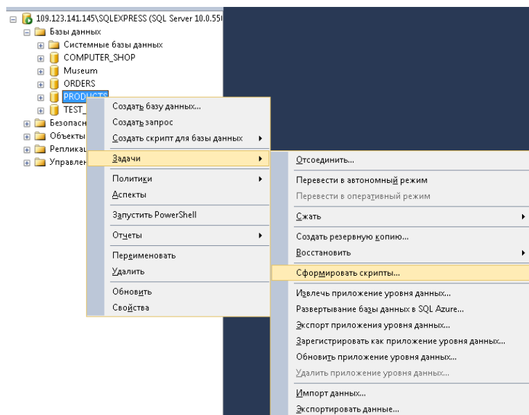
Рисунок 2 – Сформировать скрипты
