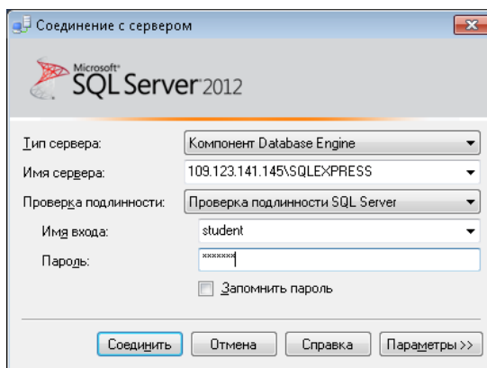
Рисунок 1 – Окно подключения
