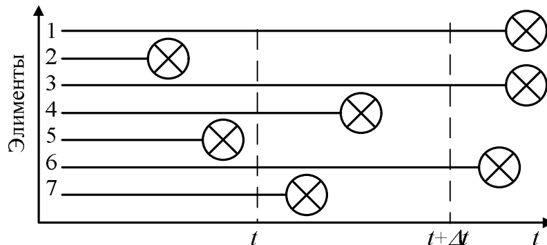
Рис. 2.2. Временная диаграмма отказов элементов
