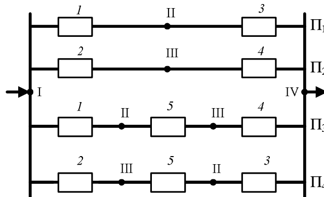
Рис. 4.9. Минимальные пути для схемы типа «мостик»
