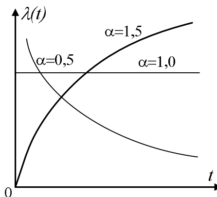
Рис. 3.22. Интенсивность отказов при распределении по закону Вейбулла
