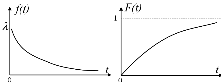
Рис. 3.5. Графики плотности f(t) и функции распределения F(t) показательного закона
