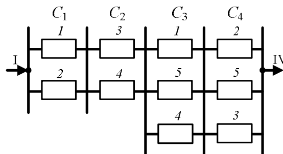
Рис. 4.10. Минимальные сечения для схемы типа «мостик»
