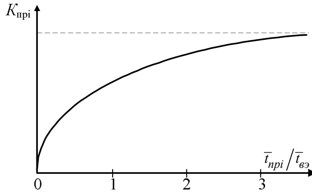
Рис. 4.3. Зависимость K_{\text{пр}} от соотношения времени преднамеренного отключения и восстановления оставшейся части системы \bar{t}_{\text{при}}/\bar{t}_{\text{вэ}}
