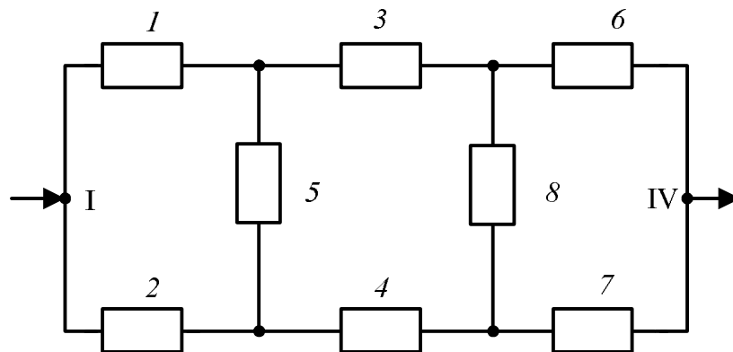
Рис. 4.7. Схема типа «двойной мостик»
