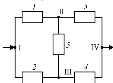
Рис. 4.5. Схема типа «мостик»
