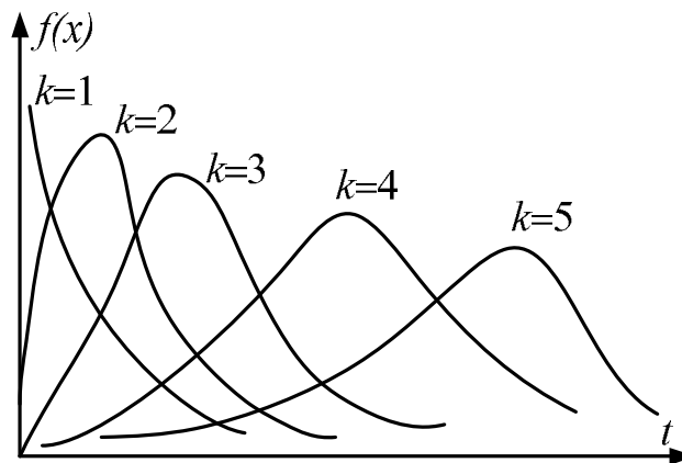
Рис. 3.17. Дифференциальная функция закона гамма-распределения времени безотказной работы при постепенных отказах
