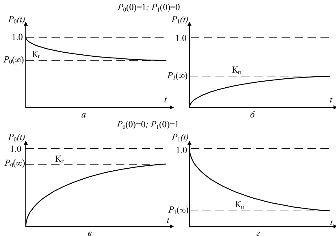
Рис. 4.2. Зависимости изменения вероятности безотказной работы и вероятности отказа одноэлементной схемы при различных начальных условиях
