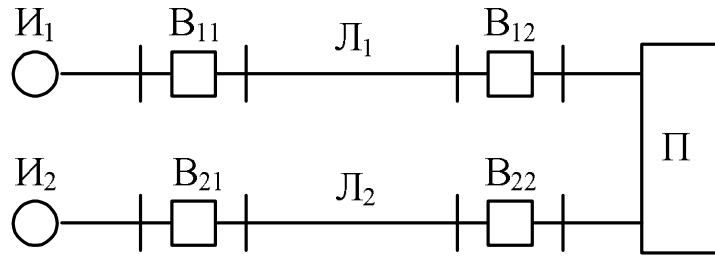
Рис. 4.4. Схема электроснабжения потребителя
