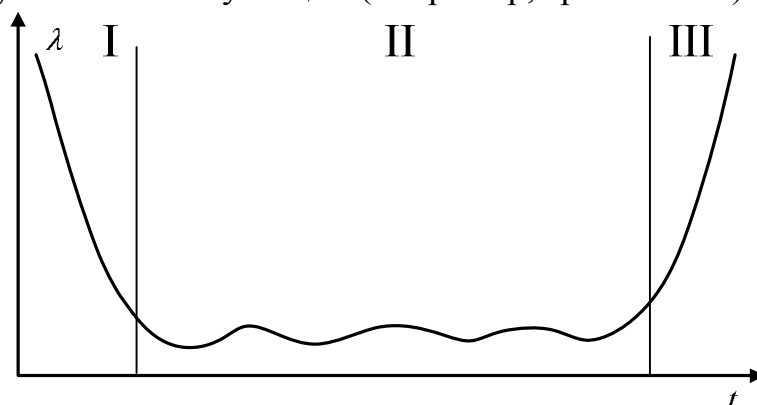
Рис. 2.3. Изменение интенсивности отказов элементов СЭС
