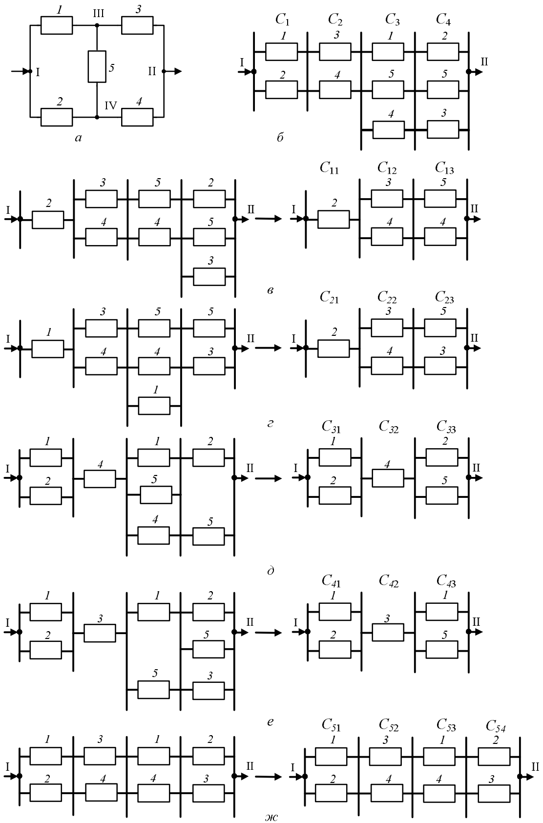
Рис. 4.11. Преобразования схемы по методу минимальных сечений
