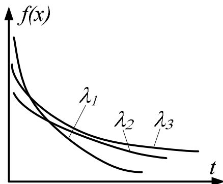
Рис. 3.16. Дифференциальная функция распределения времени безотказной работы при внезапных отказах ( \lambda_1 > \lambda_2 > \lambda_3 )
