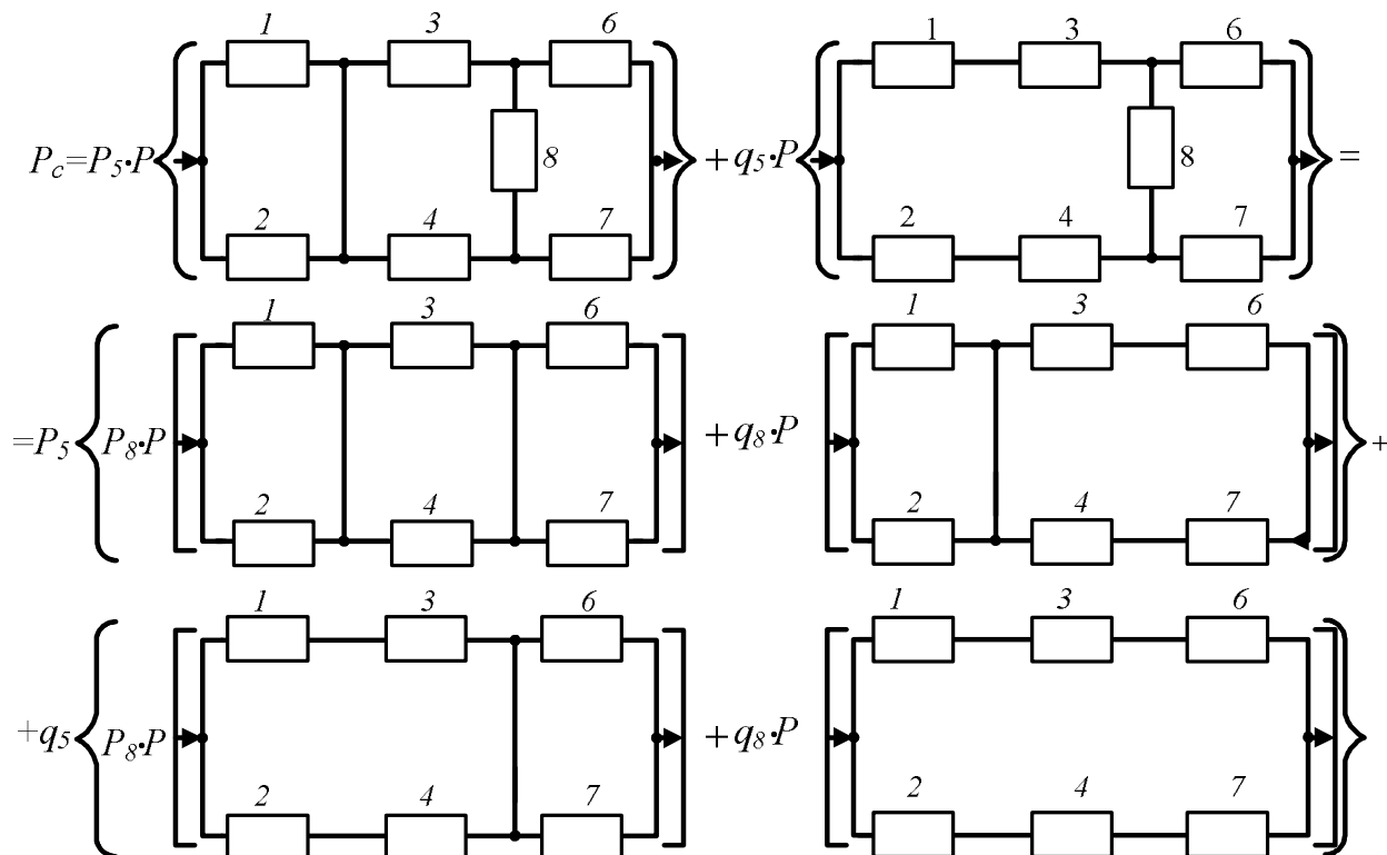
Рис. 4.8. Диаграмма, иллюстрирующая двукратное применение теоремы разложения
