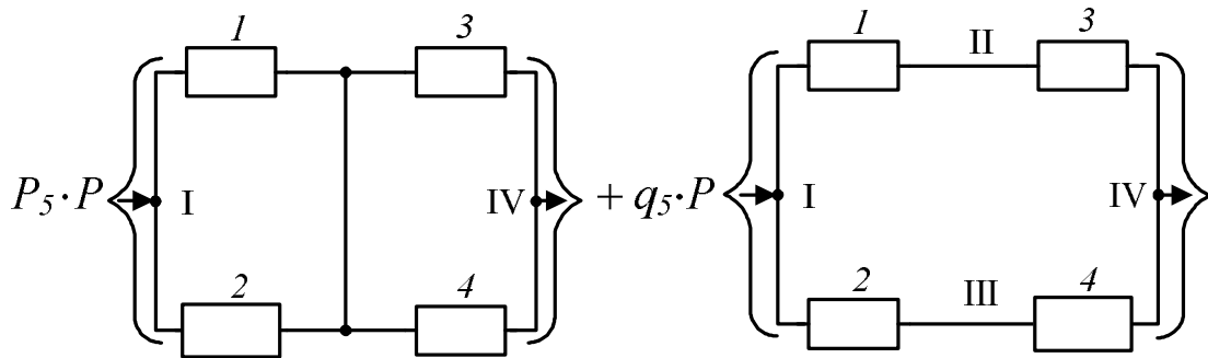
Рис. 4.6. Диаграмма, иллюстрирующая применение теоремы разложения для схемы типа «мостик»
