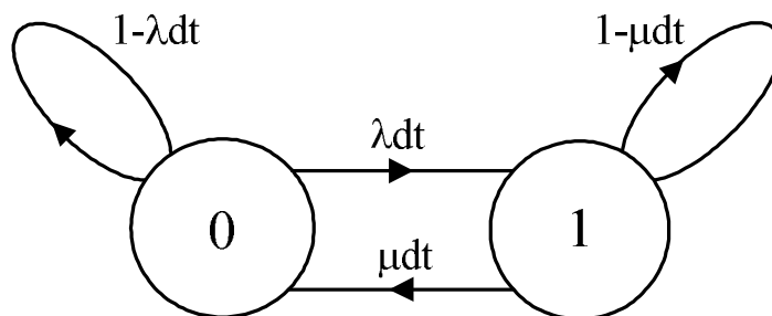
Рис. 4.1. Граф переходов для одноэлементной схемы
