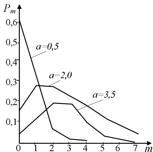
Рис. 3.3. Многоугольники распределения
