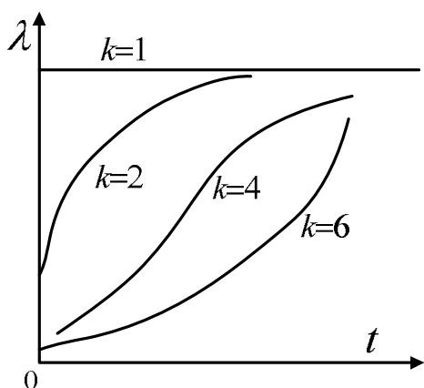
Рис. 3.18. Интенсивность отказов элемента при гамма-распределении времени безотказной работы
