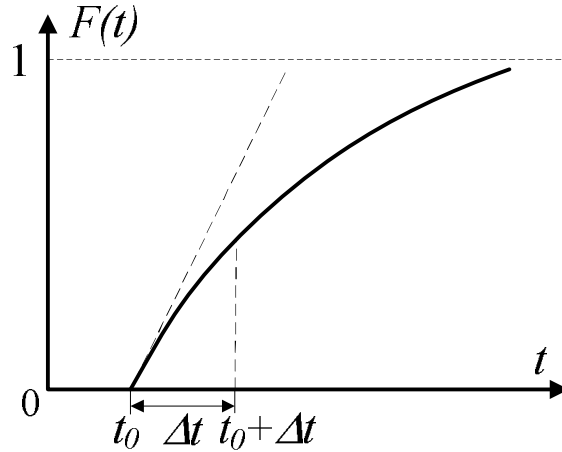
Рис. 3.20. Интегральная функция распределения времени безотказной работы участка изоляции
