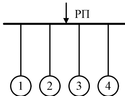
Рис. 3.1. Схема подключения электродвигателей
