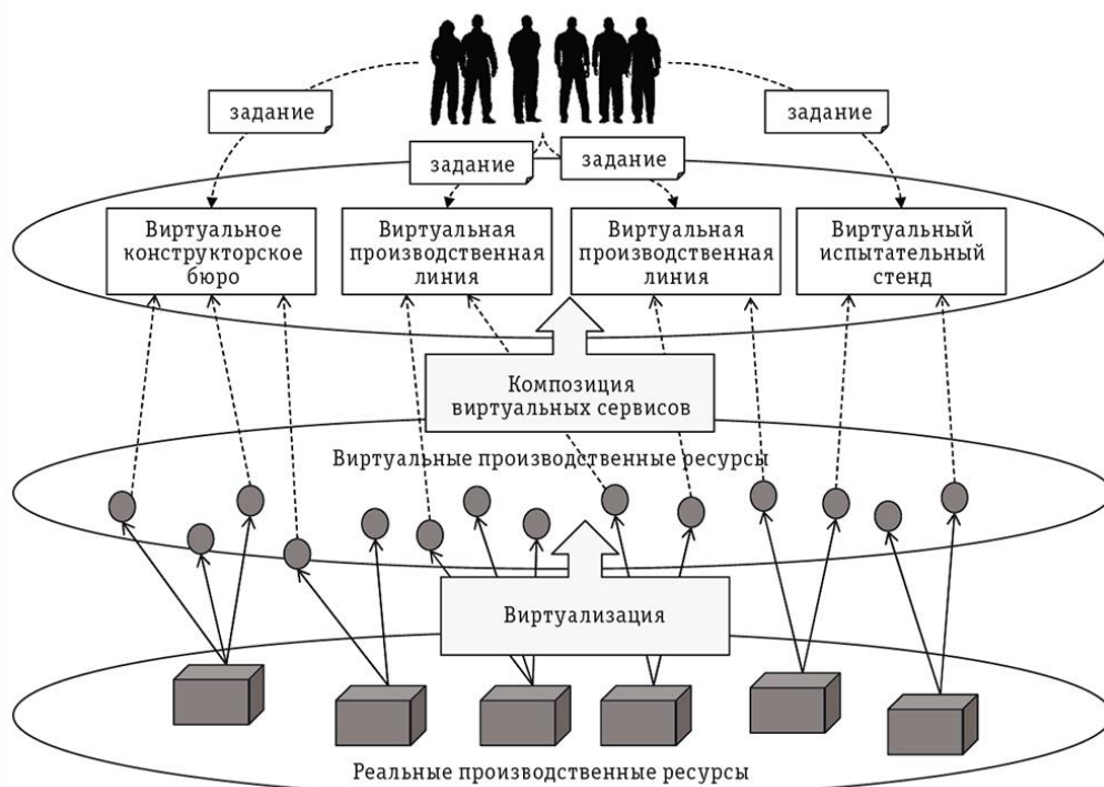
Рис. 8.5. Модель производства в концепции Industry 4
