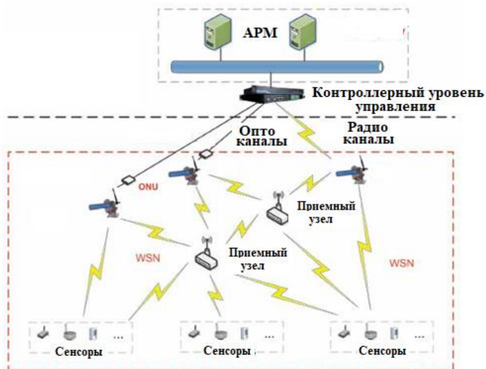
Рис. 9.12. WSN архитектура сенсорных сетей, состоящих из автономных датчиков
