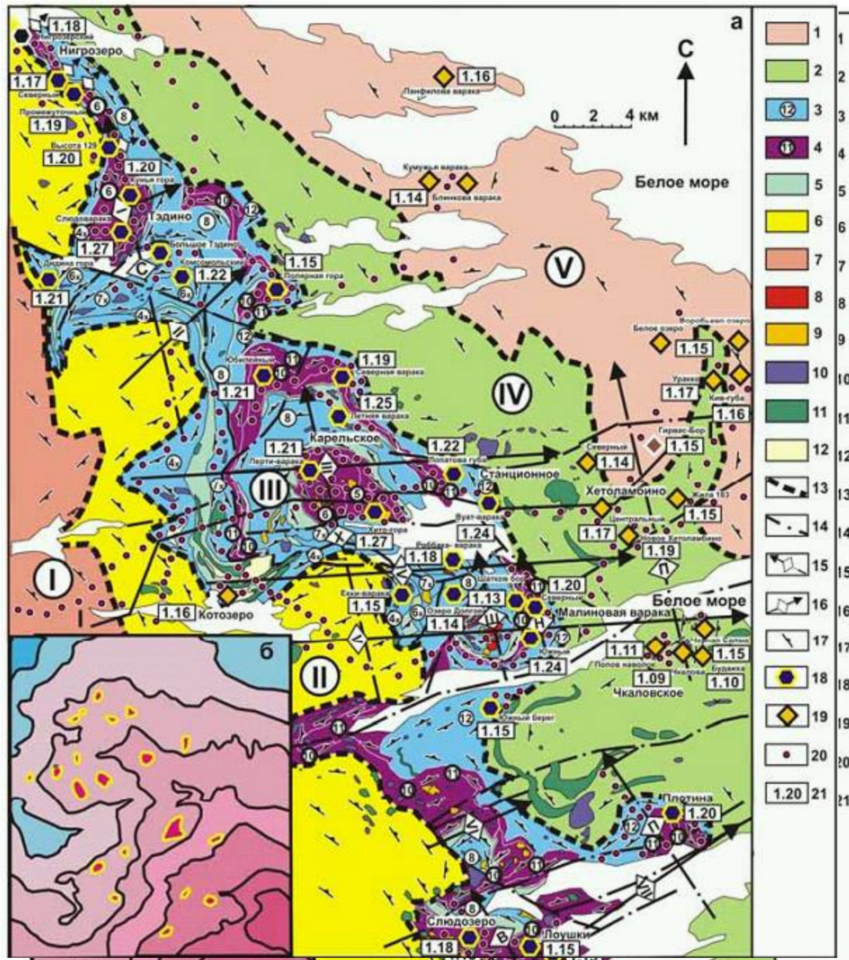
Схема геологического строения (а), гравитационного поля (б) Чупино-Лоухского слюдоносного района [Лобанов и др., 1982].
