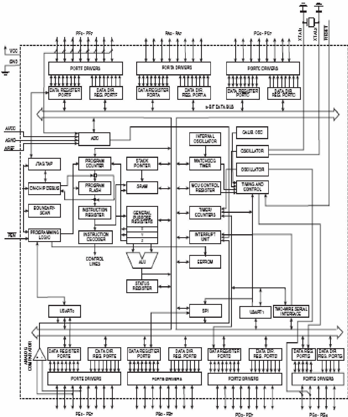
Рис. 2. Структурная схема микроконтроллера ATmega128
