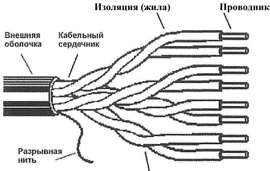
Рис. 1.2. Конструкция витой пары
