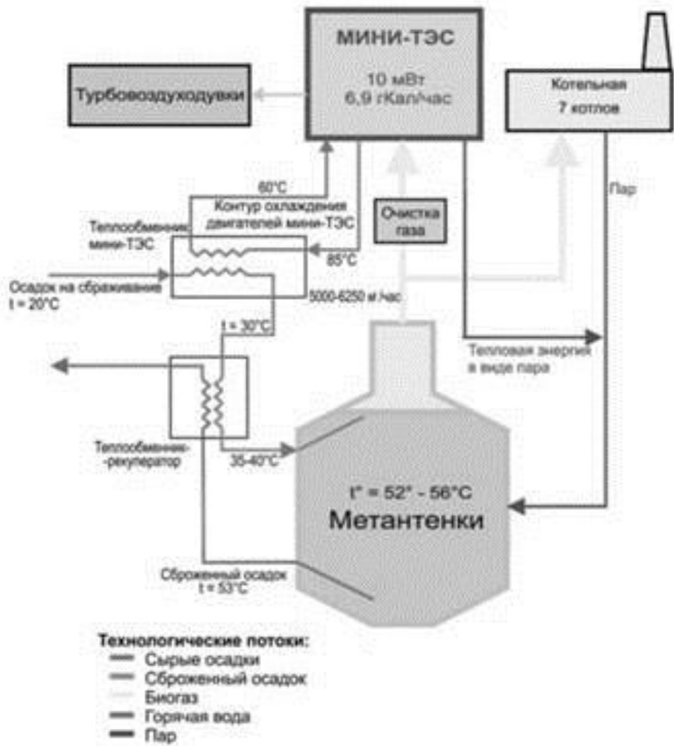
Рис. 1. Принципиальная энерготехнологическая схема мини-ТЭС
