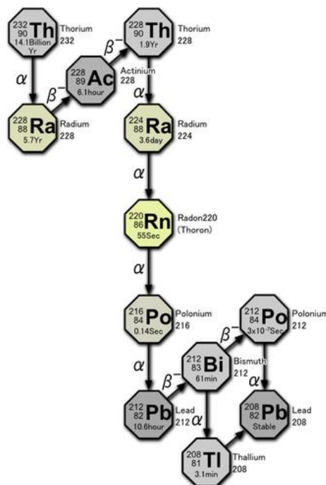
Рис. 1. Радиоактивный ряд ^{232}\text{Th}_{90}
