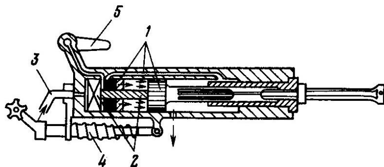
1 – воздухораспределительный механизм; 2 – механизм поворота; 3 – промывочное (продувочное) устройство; 4 – устройство для виброгашения; 5 – кран управления Рисунок 3 – Переносной перфоратор
