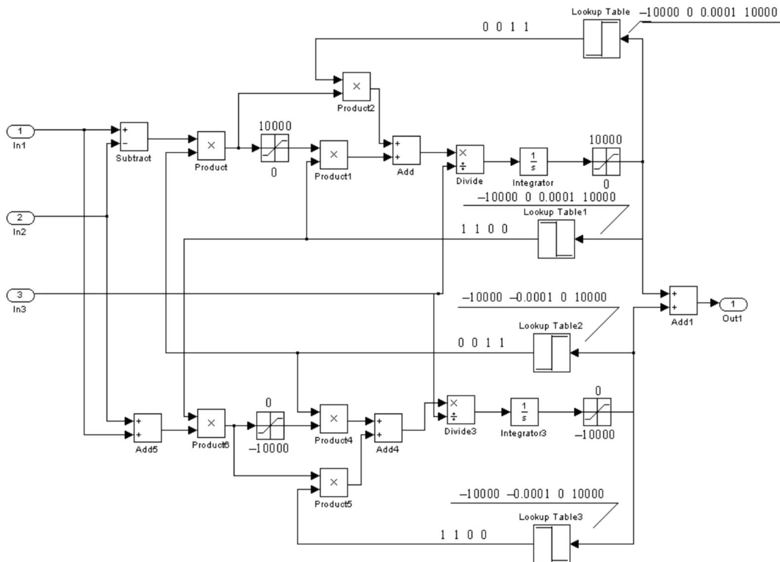
Имитационная модель реактивной нагрузки
