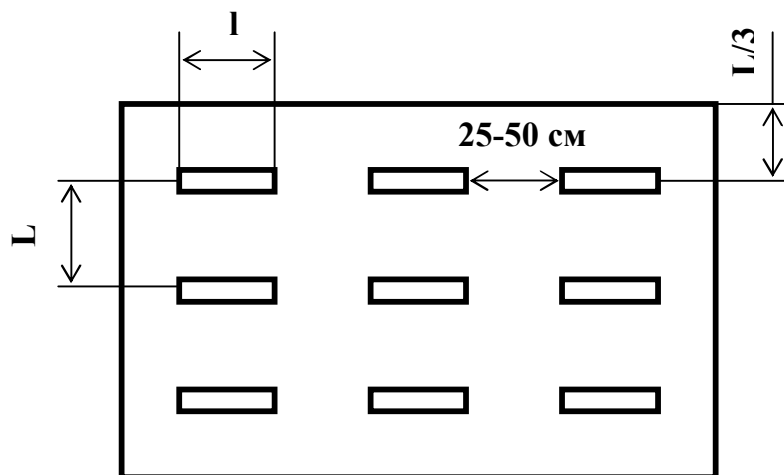
Рис. 4.3. Схема размещения светильников в помещении для люминесцентных ламп
