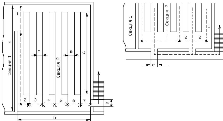
Рис. 8.1. Расчетные схемы планировки универсага.
