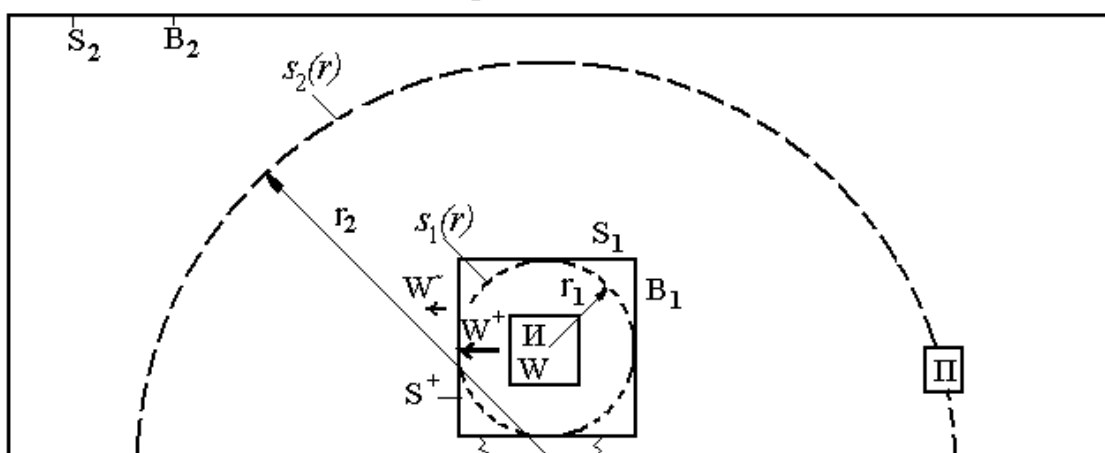
Рис.2.1. Схема потоков энергии в объеме кожуха и в объеме помещения И – источник шума, П–приемник, S+–излучающая шумовую энергию поверхность кожуха, W+–поток энергии, падающий на стенки кожуха, W~–поток энергии, выходящий из кожуха, B1–постоянная изолированного объема кожуха, B2–постоянная изолированного объема помещения.
