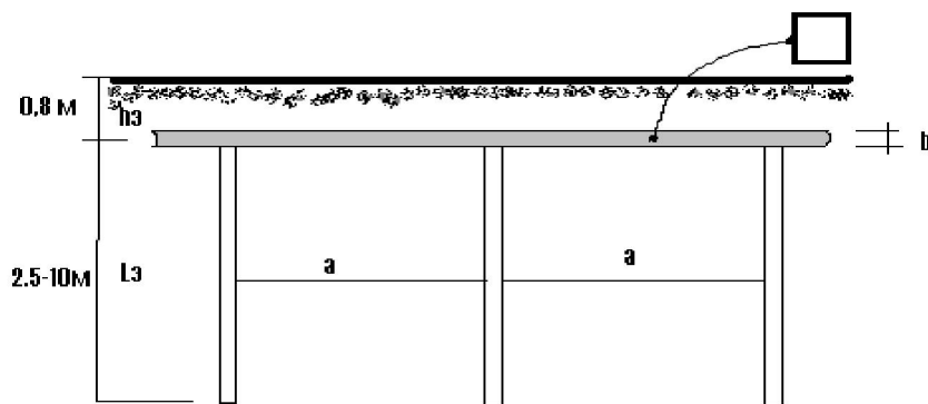
Рис. 5.2. Схема устройства искусственного группового заземления:
