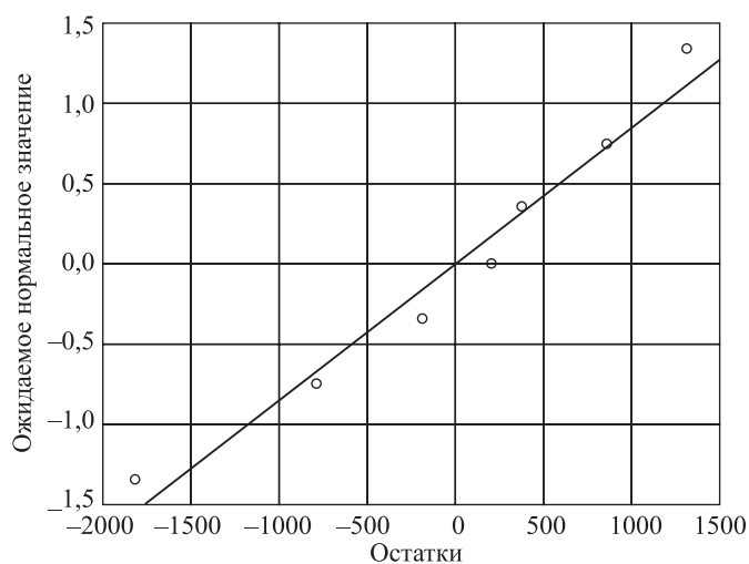
Нормальный вероятностный график остатков
