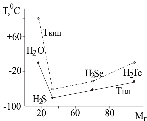
Рис 1. Зависимость температур плавления и кипения воды и её аналогов от молекулярной массы соединений.
