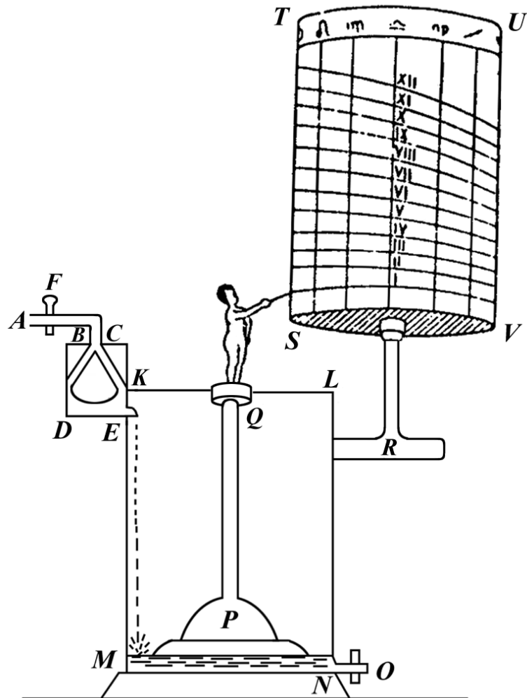
Рис. 6. Водяные часы (Архимед)
