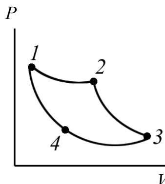
Рис. 37. Цикл Карно
