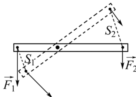
Рис. 2. Золотое правило механики:
