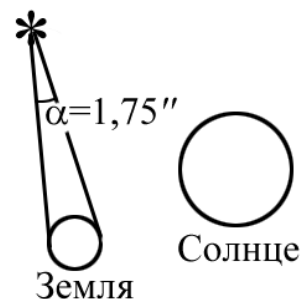
Рис. 28. Отклонение луча света вблизи солнца
