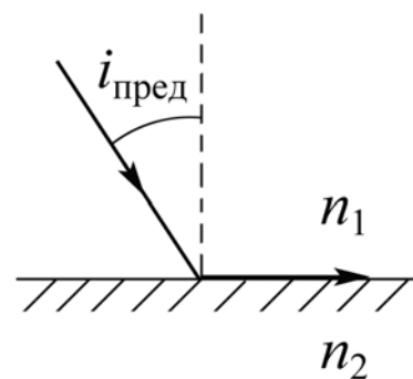
Рис. 60. Явление полного внутреннего отражения
