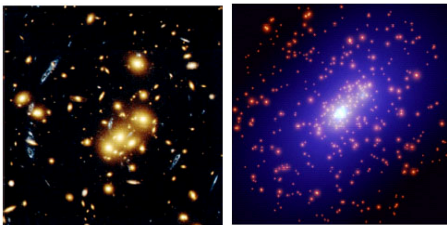
Рис. 31. Гравитационное линзирование
