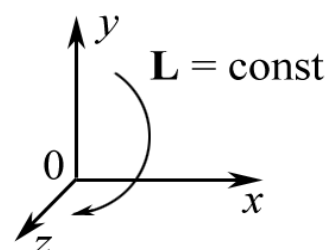
Рис. 23. Закон сохранения момента импульса
