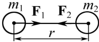
Рис. 26. Силы гравитационного взаимодействия
