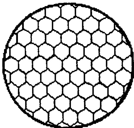
Рис. 41. Правильные шестиугольные ячейки на поверхности жидкости (ячейки Бенара)
