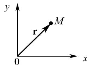
Рис. 14. Радиус-вектор ( r )
