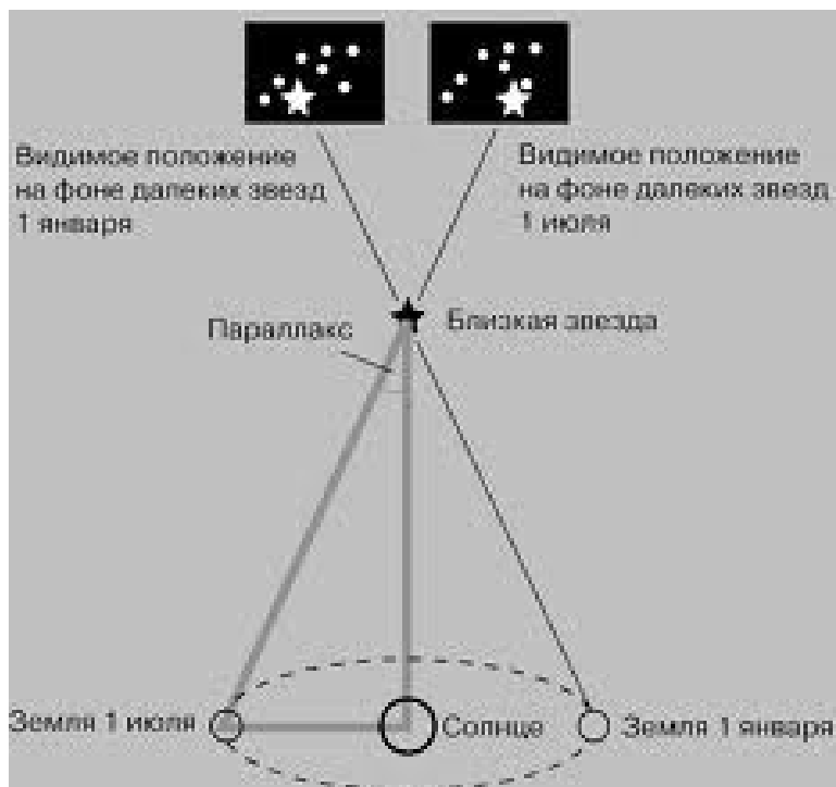
Рис. 34. Схематическое объяснение параллакса
