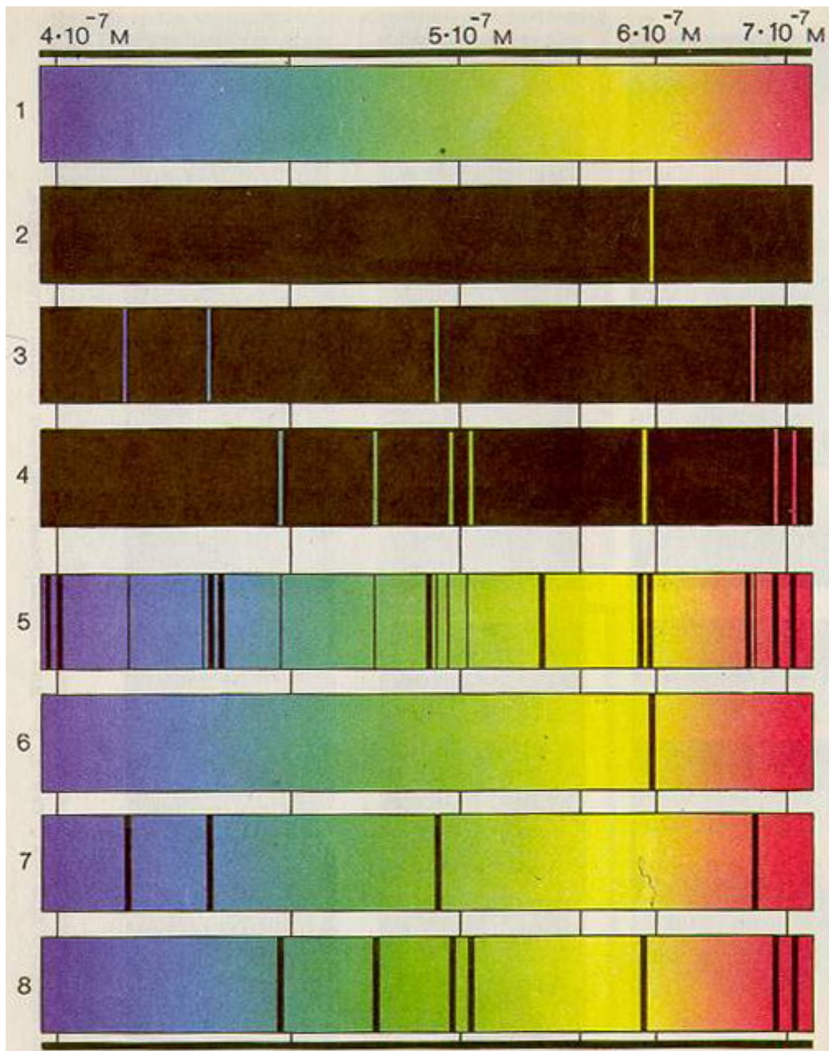
Рис. 15. Спектры испускания: 1 – сплошной; 2 – натрия; 3 – водорода; 4 – гелия. Спектры поглощения: 5 – солнечный; 6 – натрия; 7 – водорода; 8 – гелия
