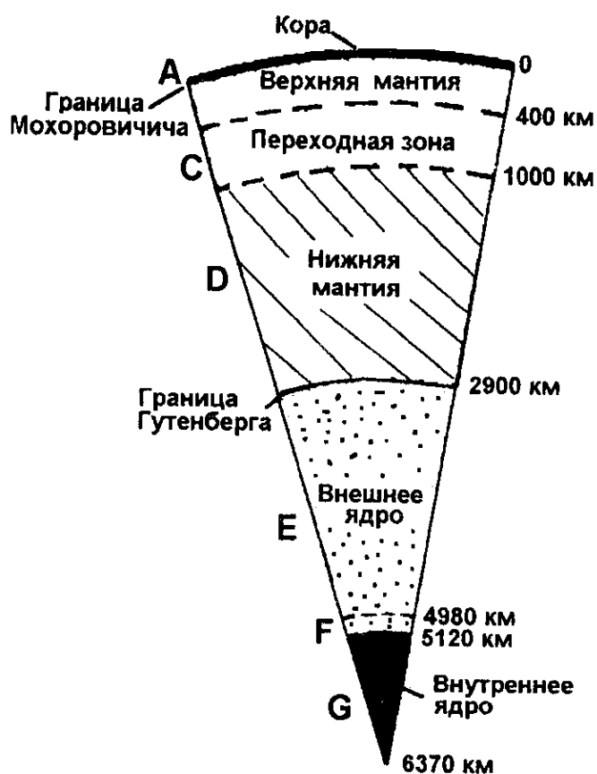
Рис. 45. Схема внутреннего строения Земли
