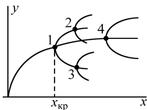
Рис. 50. Точки бифуркаций
