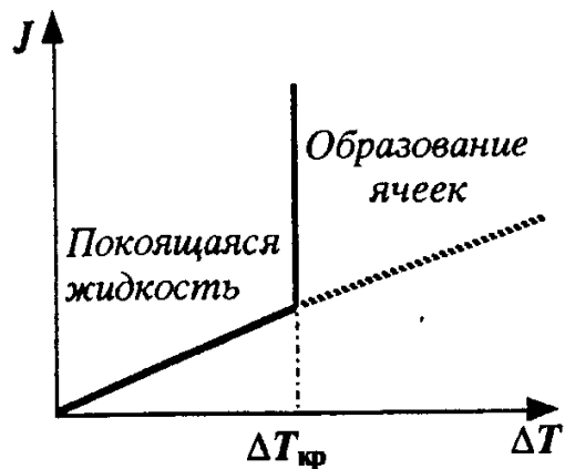
Рис. 42. Зависимость полного теплового потока J в единицу времени от разности температур
