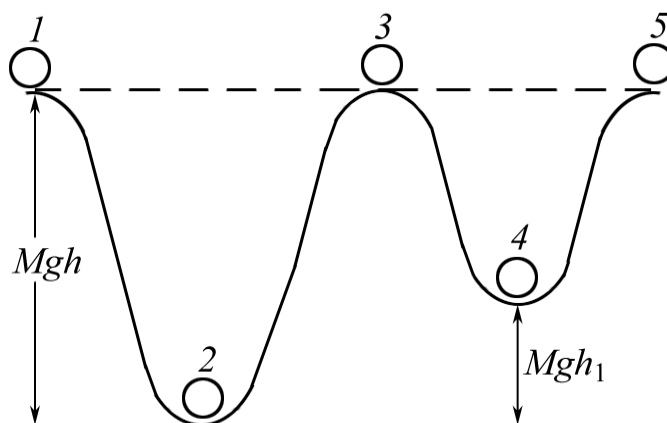
Рис. 35. Пример устойчивых и неустойчивых положений тела: 1, 3, 5 – неустойчивые; 2, 4 – устойчивые
