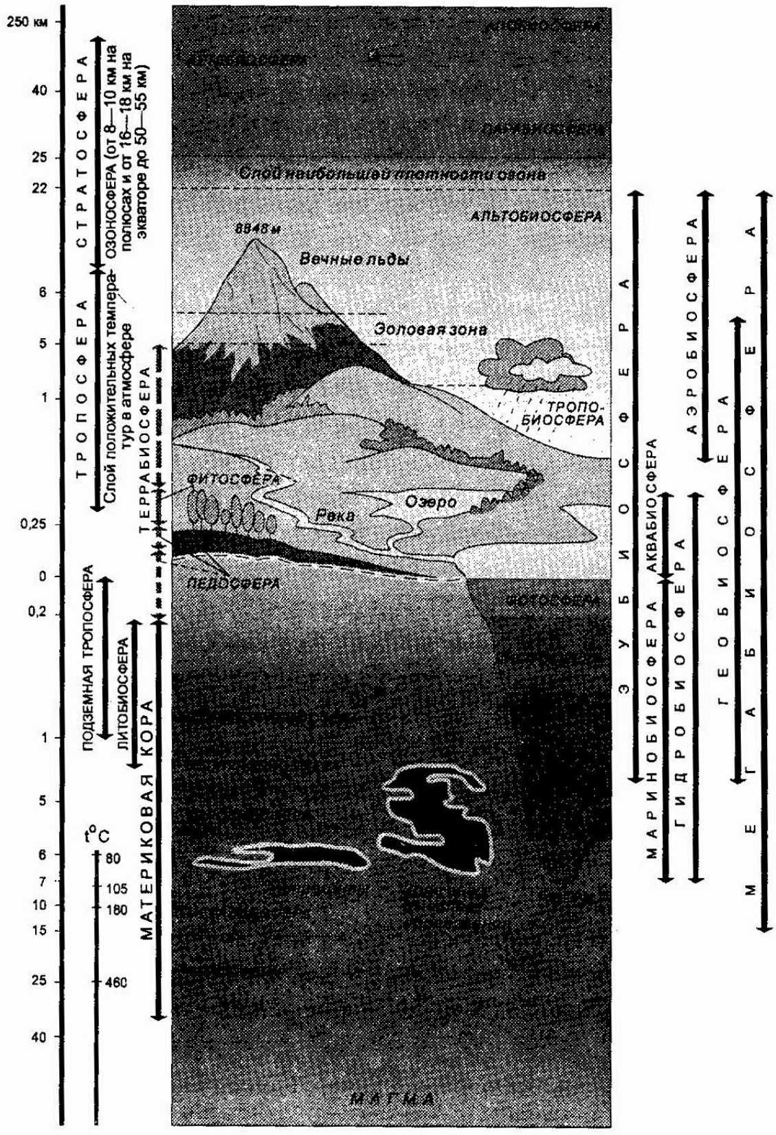
Рис. 44. Оболочки Земли
