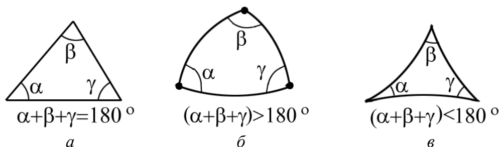
Рис. 25. Признаки геометрии
