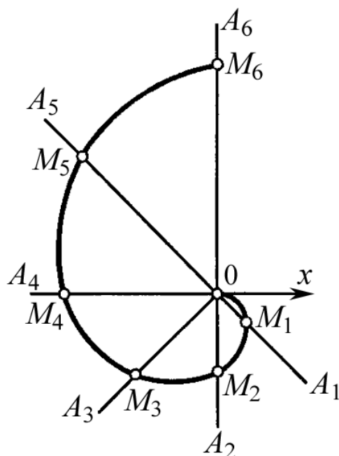
Рис. 7. Спираль Архимеда
