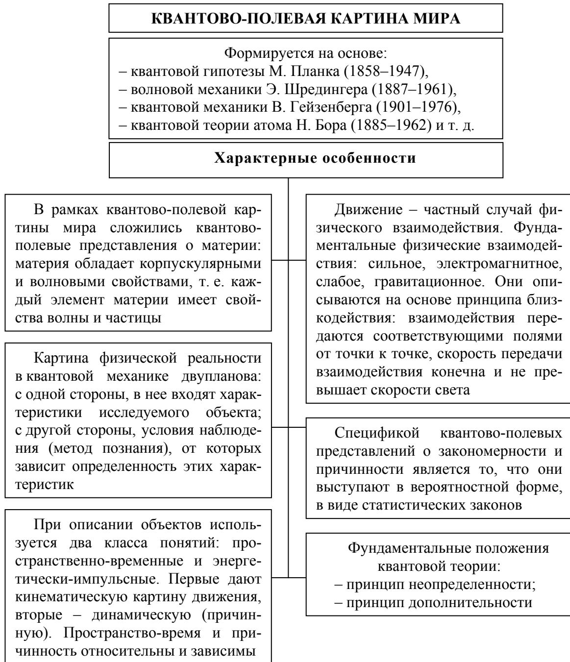
Рис. 19. Квантово-полевая картина мира
