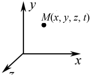
Рис. 20. Представление точки в четырехмерном пространстве
