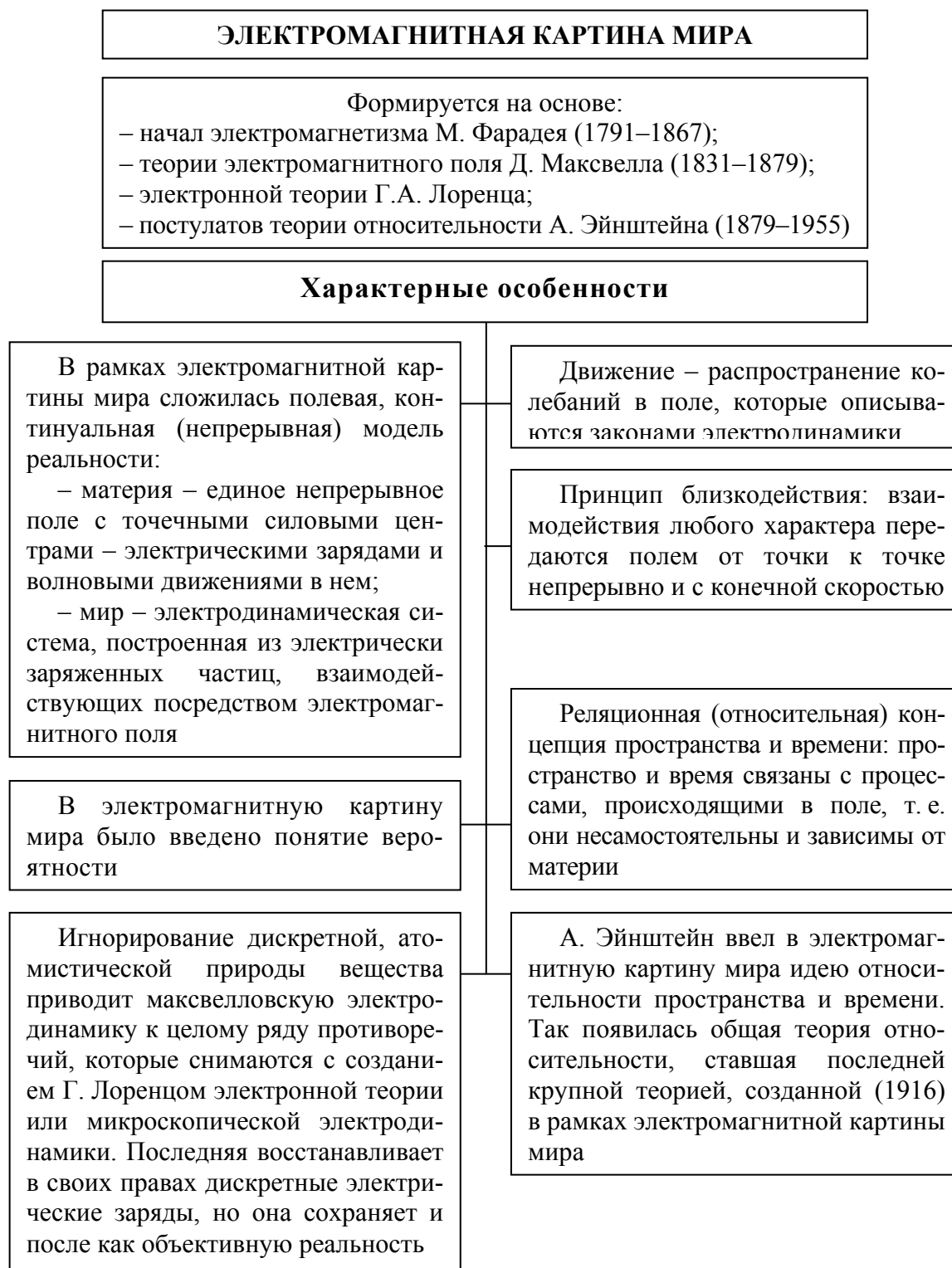
Рис. 17. Электромагнитная картина мира
