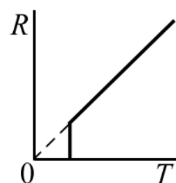
Рис. 24. График зависимости R(T) при сверхпроводимости
