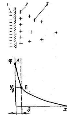
Рис.3. Модель строения ДЭС Штерна.
