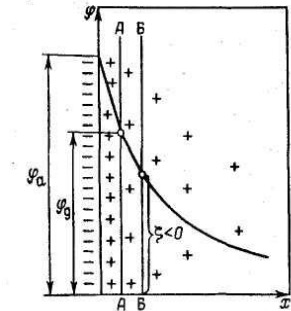
Рис.4. Современная модель строения ДЭС.
