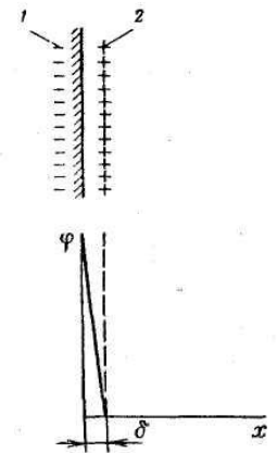
Рис.1. Модель строения ДЭС Гельмгольца.
