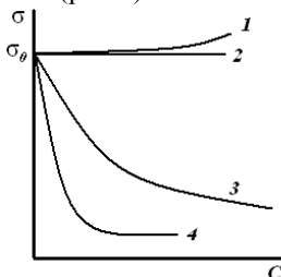
Рис. 2. Изотермы поверхностного натяжения: 1, 2 – ПИВ; 3 – ПАВ, 4 – мицеллообразующие ПАВ.
