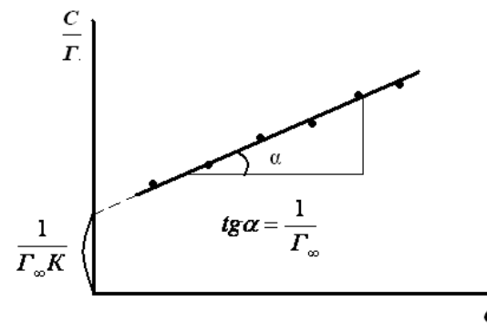
Рис.4. Изотерма адсорбции в координатах линейной формы уравнения Лэнгмюра.
