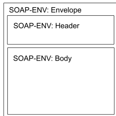
Рис. 4.4. SOAP-конверт
