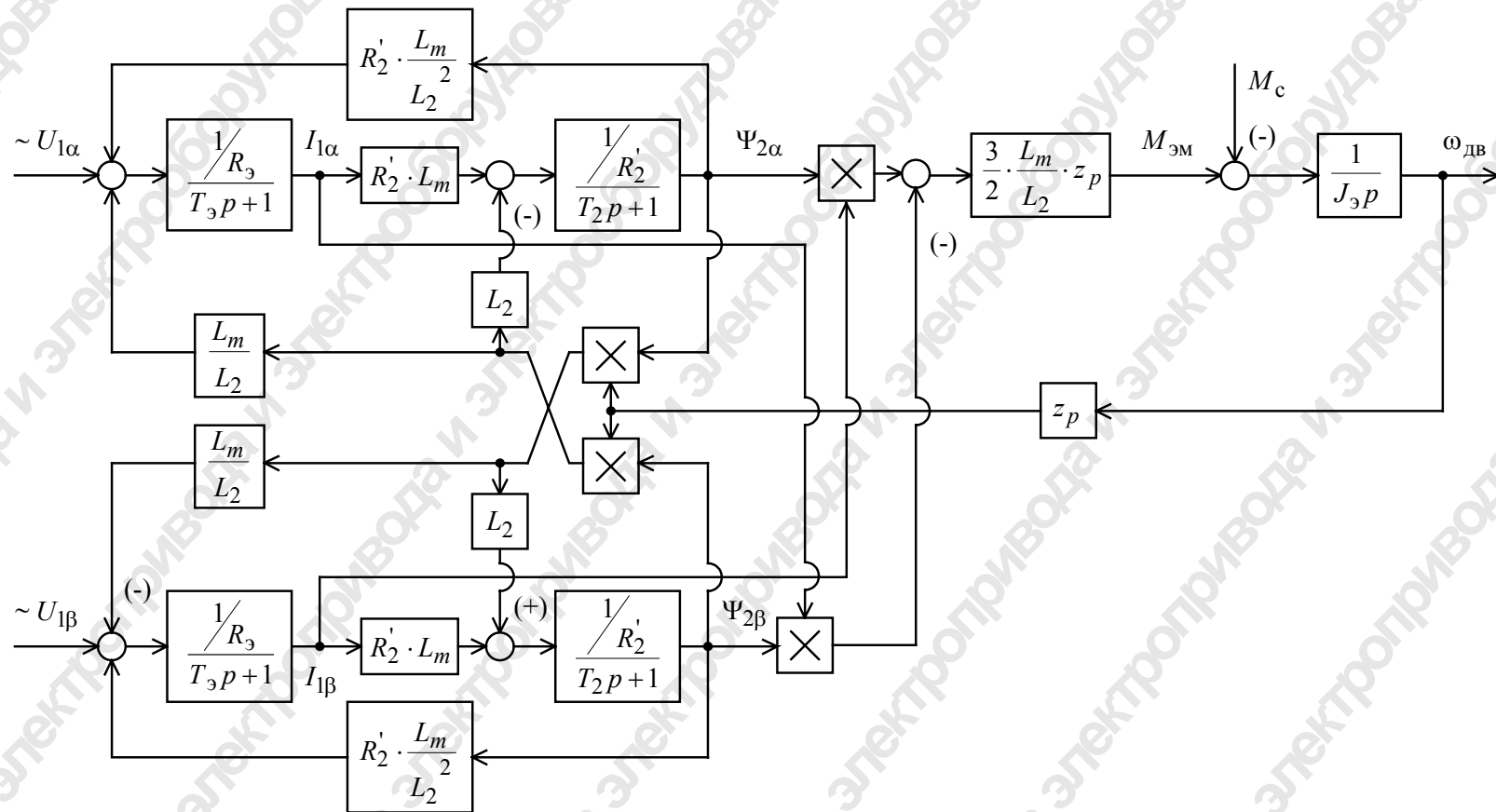
Рис. 2.1. Структурная схема асинхронного электродвигателя в неподвижной системе координат статора \alpha, \beta
