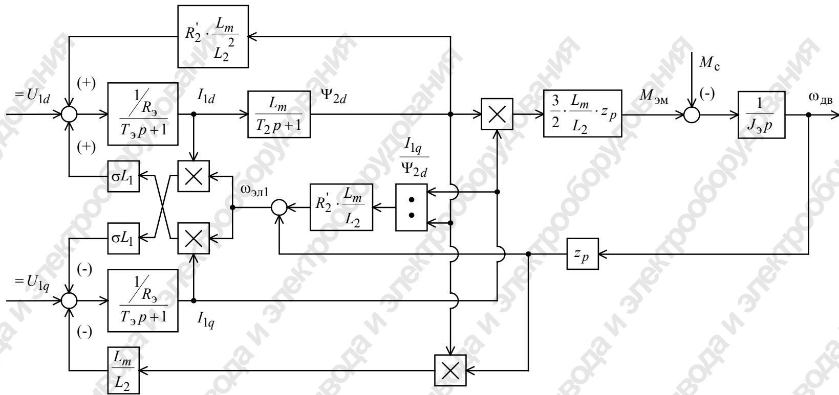
Рис. 2.3. Структурная схема асинхронного электродвигателя с короткозамкнутым ротором во вращающейся системе координат d, q , ориентированной по результирующему вектору потокосцепления ротора
