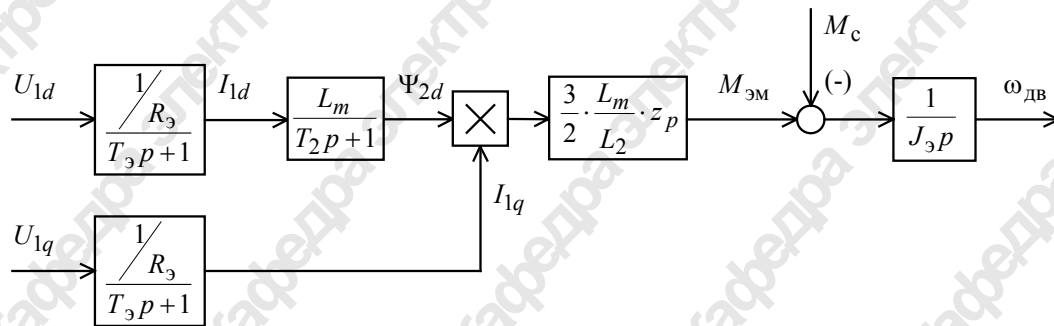
Рис. 2.4. Структурная схема асинхронного электродвигателя во вращающейся системе координат d, q , ориентированной по результирующему вектору потокосцепления ротора, при компенсации внутренних обратных связей
