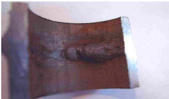
Рис. 1.2. Поперечный разрез трубы с дефектным швом
