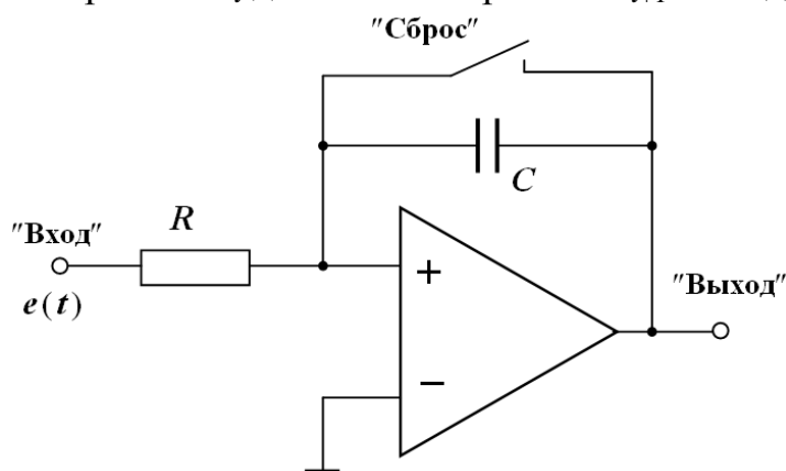
Рис. 3. Принципиальная схема электронного интегратора: 1/RC = 31,3 \text{ с}^{-1}
