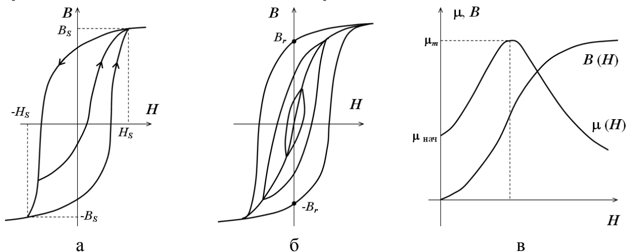
Рис. 1. Статические кривые намагничивания ферромагнетика: а – симметричные и несимметричные гистерезисные циклы; б – семейство симметричных частных гистерезисных циклов; в – кривая первоначального намагничивания.
