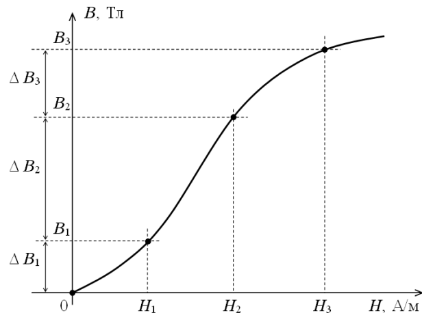
Рис. 6. Построение кривой первоначального намагничивания.
