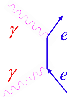
эффект Комптона
