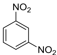
1,3-динитробензол
