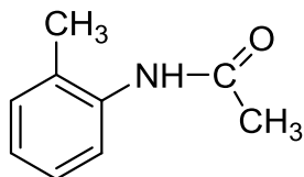
N-(о-толил)ацетамид
