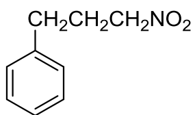
1-нитро-3-фенилпропан
