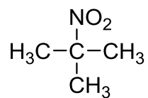
2-нитро-2-метилпропан
