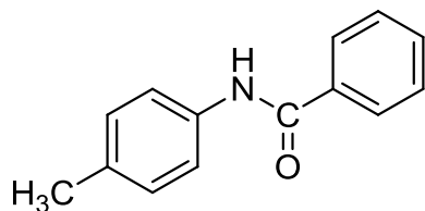
N-( p -толил)бензамид
