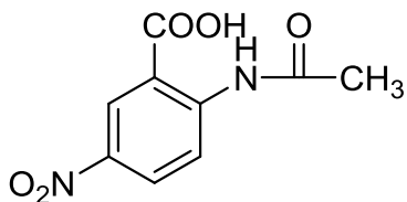
2-ацетамид-5-нитробензойная кислота
