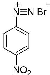
p -нитробензолдиазонийбромид (бромистый p -нитробензолдиазоний)
