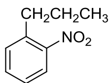
1-нитро-2-пропилбензол
