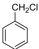
бензилхлорид
