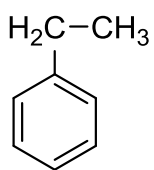
этилбензол
