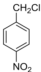
4-нитро-бензилхлорид
