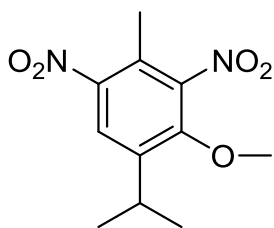
1-изопропил-2-метокси-4-метил- -3,5-динитробензол
