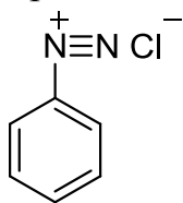
Бензолдиазонийхлорид (Хлористый бензолдиазоний)
