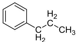
пропилбензол
