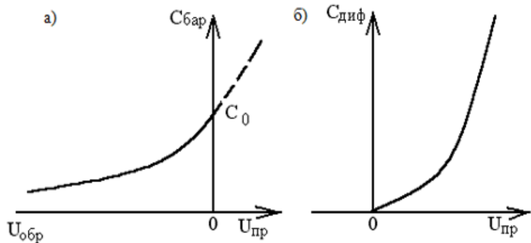
Зависимость барьерной (а) и диффузионной (б) емкости от приложенного напряжения
