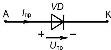
Включение диода в прямом направлении
