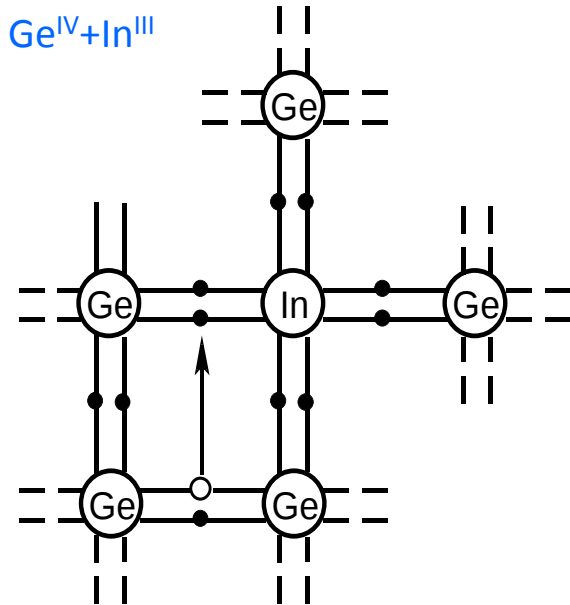
Процесс образования дырки
