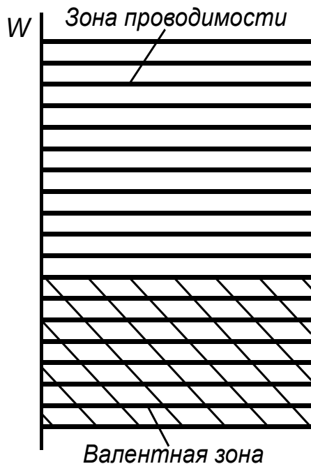
проводник
