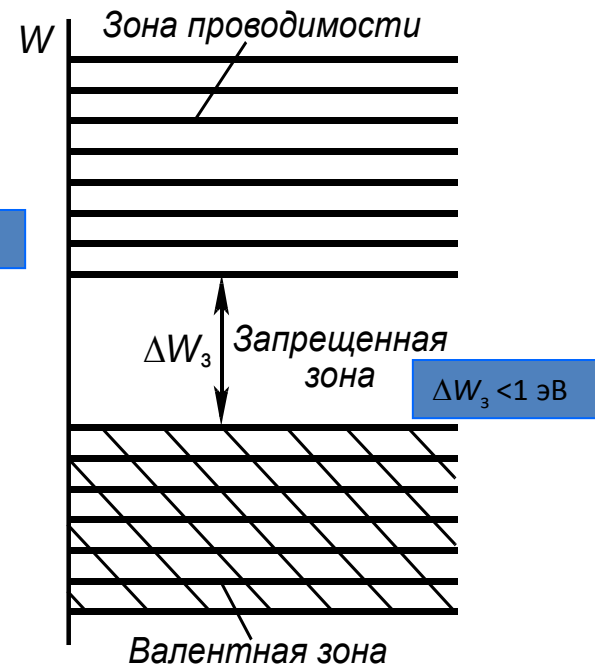
полупроводник
