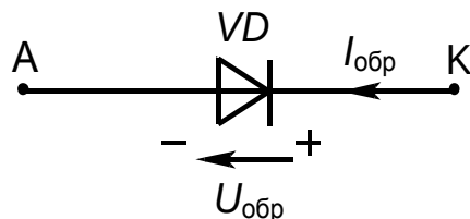
Включение диода в обратном направлении
