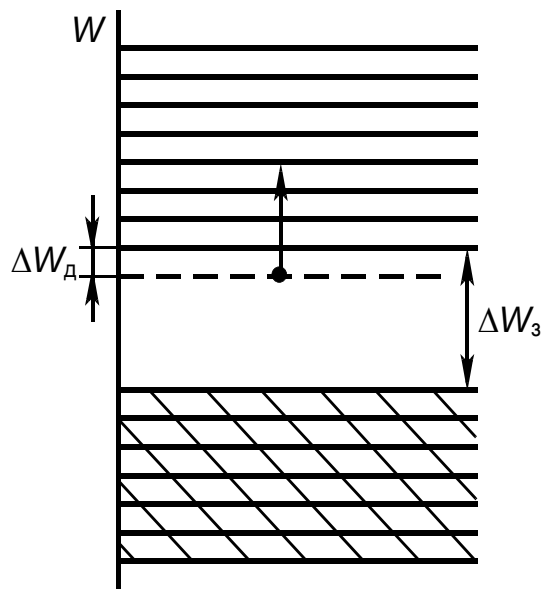
Процесс образования свободного электрона
