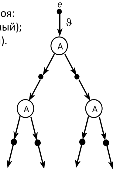
Механизм лавинного пробоя
