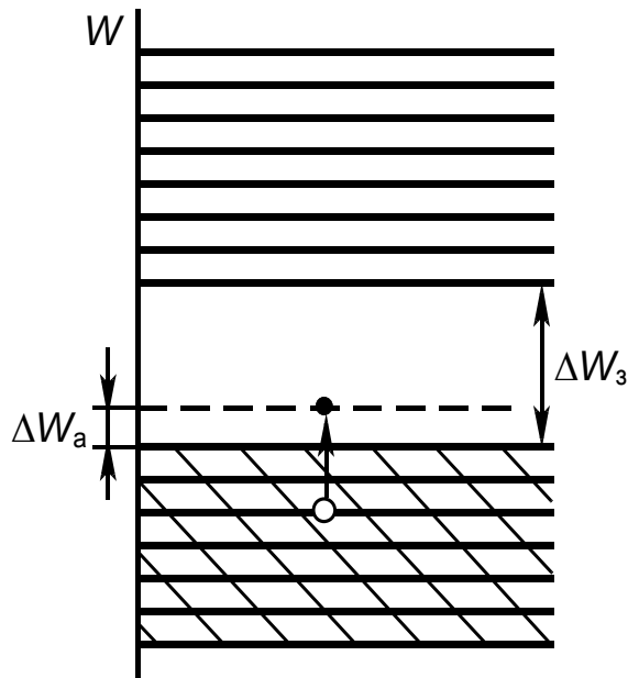
Процесс образования дырки
