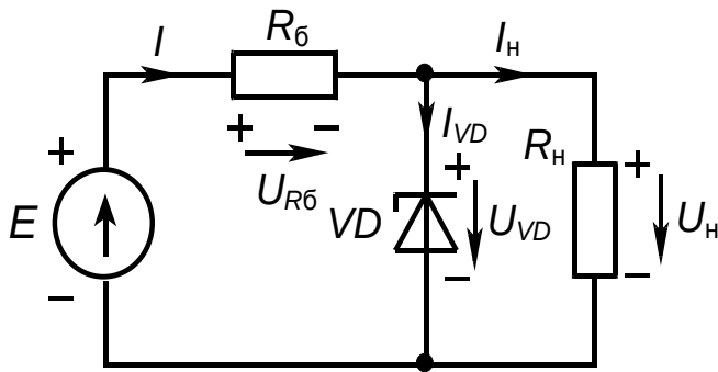
Схема параметрического стабилизатора. R_6 – балластный резистор
