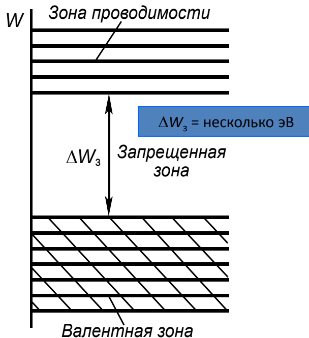
диэлектрик
