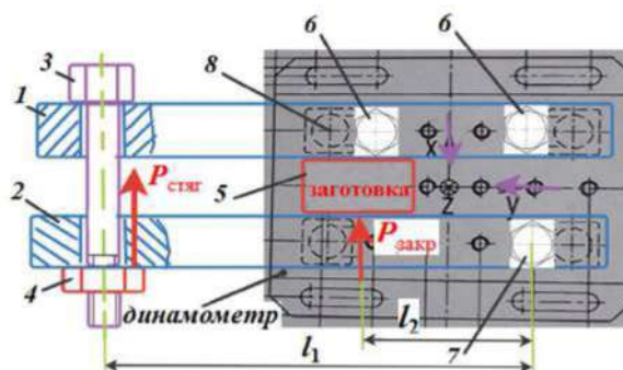
Рис. 1. Схема закрепления образца на динамометре Kistler. 1 – планка А; 2 – планка Б; 3 – болт М12; 4 – гайка М12; 5 – заготовка; 6 – болт М8 (2 шт.); 7 – болт М8; 8 – датчики динамометра.
