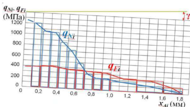
Рис. 3. Гистограммы удельных касательных q_{Fi} и нормальных q_{Ni} контактных нагрузок (МПа) на i -том участке пластины B . Абсцисса – расстояние от режущей кромки x_{Ai} (мм). Сталь 40Х – Т15К6, \gamma = +7^\circ ; v = 120 м/мин; a = s = 0,368 мм; b = 4 мм; c = 1,844 мм; c_1 = 0,922 мм; P_{y \text{ экп}} = 1623 Н; P_{z \text{ экп}} = 3061 Н; F_{\text{экп}} = 2014 Н; N_{\text{экп}} = 2837 Н.
