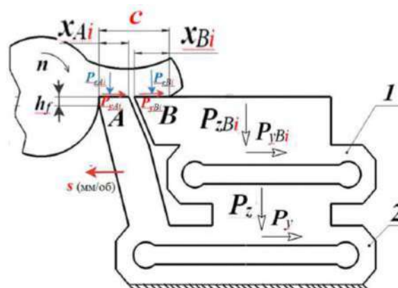
Рис. 1. Положение пластин А и В разрезного резца при контакте стружки с основной измерительной пластиной В на участке длиной x_{Bi} и шириной b .
