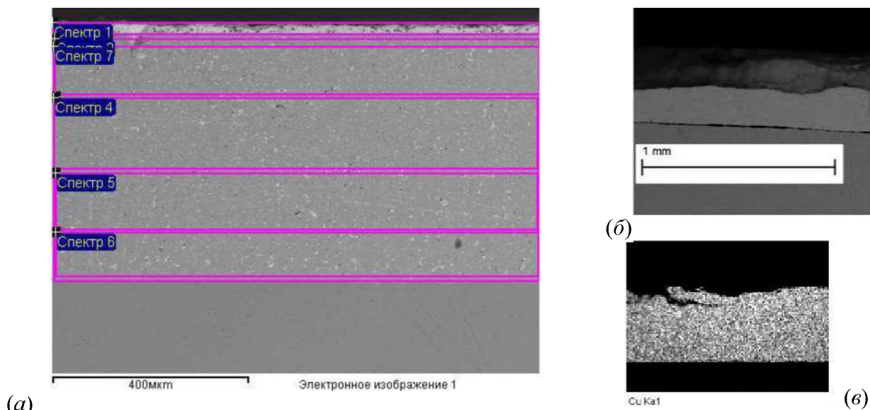
Рис. 2. Микрофотография СЭМ с торца вкладыша, отражающая слоистый характер трибослоя (а), микрофотография фрагмента верхнего поверхностного слоя (б) и верхнего слоя с катированием по Cu (в)
