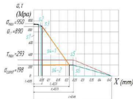
Рис. 6. Проверка правильности построения эпюр нормальных \sigma и касательных \tau контактных напряжений на передней поверхности резца. Сталь 40X-T15K6; t=2 мм; v=120 м/мин; \gamma=7^\circ , \varphi=45^\circ , s=0,07 мм/об.
