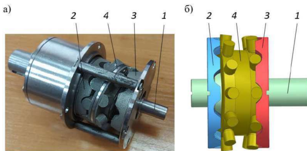
1 – ведущий вал; 2 – ведомый кулачок; 3 – остановленный кулачок; 4 – сателлит
