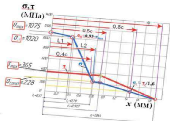
Рис. 4. Упрощенные формы эпюр нормальных \sigma и касательных \tau контактных напряжений (МПа) на передней поверхности резца. Сталь 40X – T15K6, \gamma = +7^\circ ; v = 120 м/мин; a = s = 0,368 мм.
