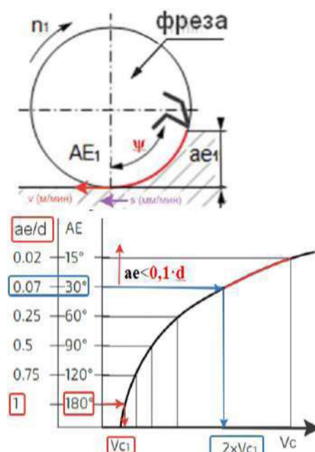
Рис. 1. Влияние длины дуги контакта AE и соотношения ae/d на скорость резания V_c . Ti-6Al-4V-BK8 [1].
