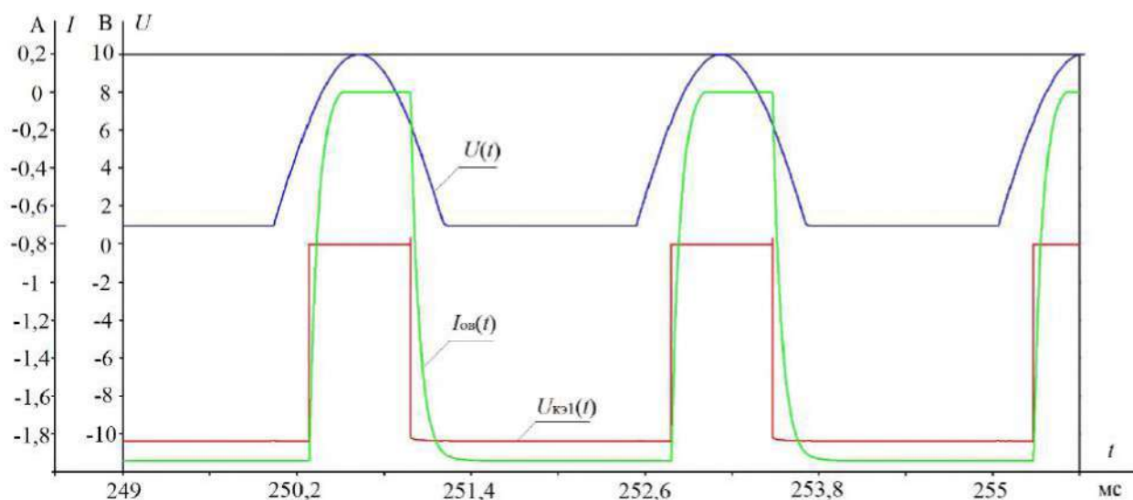
Рис. 2. Диаграммы тока возбуждения I_{ов}(t) , напряжения коллектор-эмиттер U_{кз1}(t) транзистора VT1 и выпрямленного напряжения U(t) с канала измерения
