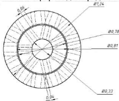
Рисунок 1 – Двухпоточная вихревая горелка с лопаточными завихрителями
