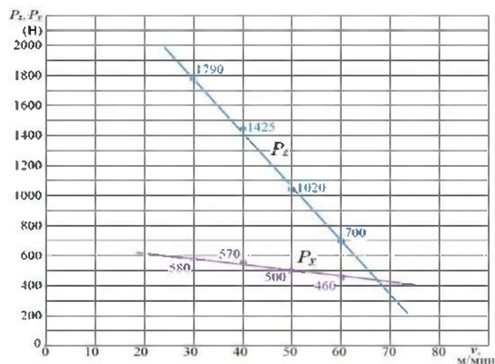
Рисунок 2. Влияние скорости резания v (м/мин) на составляющие P_x и P_z (Н) силы резания при обработке неизношенным резцом ВТЗ-1-ВК8, \gamma = 0^\circ , b = 2,3 мм, \alpha = 10^\circ , s_y = 0,21 мм/об
