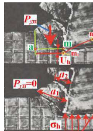
Рис. 2. Упругое восстановление поверхности резания m_1n_1
