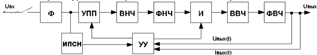
Рис. 1. Структурная схема источника питания системы охлаждения компьютерного оборудования автономного объекта.
