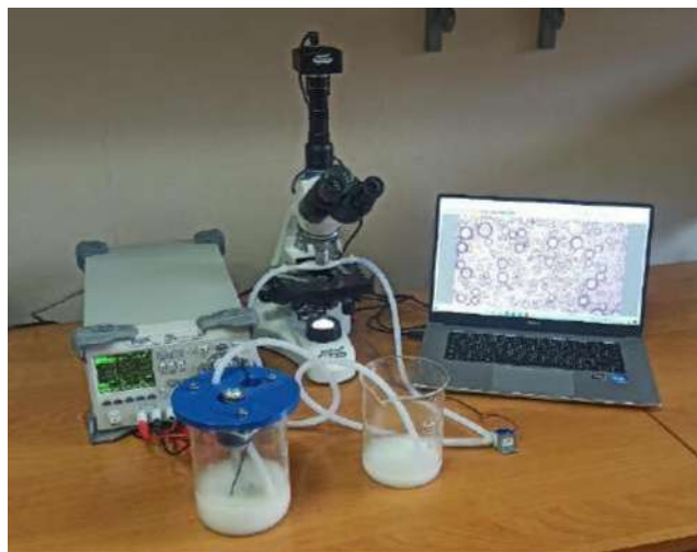
Рис.1 – Программно-аппаратный комплекс для определения дисперсного состава водомасляных эмульсий
