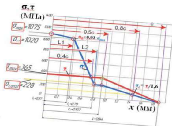
Рис. 4. Эпюры нормальных \sigma и касательных \tau контактных напряжений (МПа) на передней поверхности резца. Сталь 40Х – Т15К6, \gamma = +7^\circ ; v = 120 м/мин; a = s = 0,368 мм; b = 4 мм; c = 1,844 мм; c_1 = 0,922 мм; P_{y \text{ эксп}} = 1623 Н; P_{z \text{ эксп}} = 3061 Н; F_{\text{эксп}} = 2014 Н; N_{\text{эксп}} = 2837 Н.
