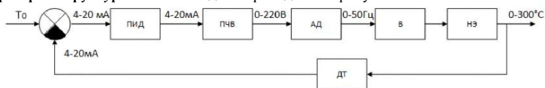
Рис. 1. Операторно-структурная схема САР температуры
