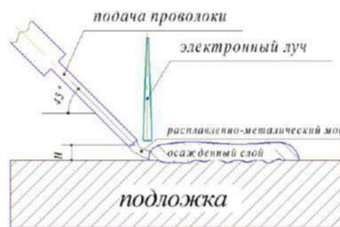
Рис.2. Принцип электронно-лучевой наплавки проволокой аддитивной технологии
