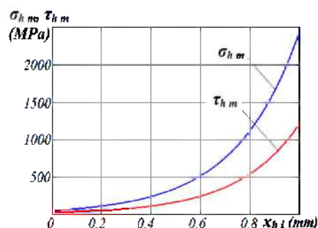
Рис. 3. Распределение средних контактных напряжений на фаске задней поверхности [МПа] при установившемся резании. Сталь 40Х-T15K6, t = 2 мм, v = 120 м/мин. Ордината – средние нормальное \sigma_{hm} [МПа] и касательное \tau_{hm} [МПа] контактные напряжения на фаске задней поверхности; абсцисса – расстояние от режущей кромки вдоль длины фаски износа по задней поверхности перпендикулярно главной режущей кромки x_{hi} [мм]
