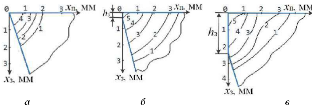
Рис. 1. Распределение температуры в режущем клине при обработке титанового сплава ВТ3-1 – ВК8, \gamma = 0^\circ \alpha = 18^\circ , v = 60 м/мин, s = 0,21 мм/об. а – h_3 = 0,05 мм; б – h_3 = 0,5 мм; в – h_3 = 2,5 мм. 1 - 500°С; 2 - 600°С; 3 - 700°С; 4 - 800°С; 5 - 900°С.
