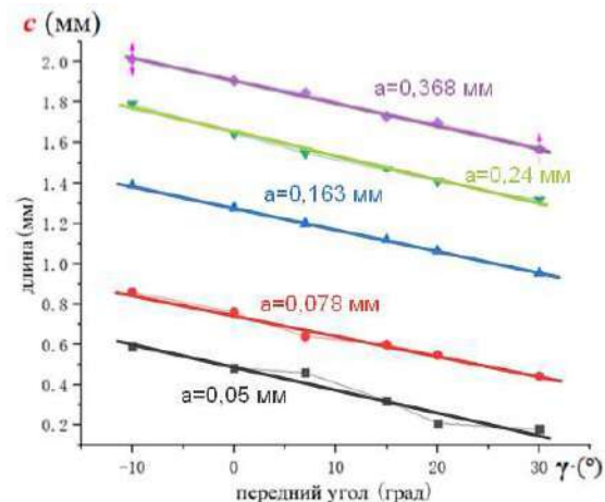
Рис. 2. Графики изменения длины контакта стружки c (мм) с передней поверхностью резца в зависимости от переднего угла \gamma (°) и толщины среза a (мм) при \phi = 45^\circ . Сталь 40X – T15K6, v = 120 м/мин
