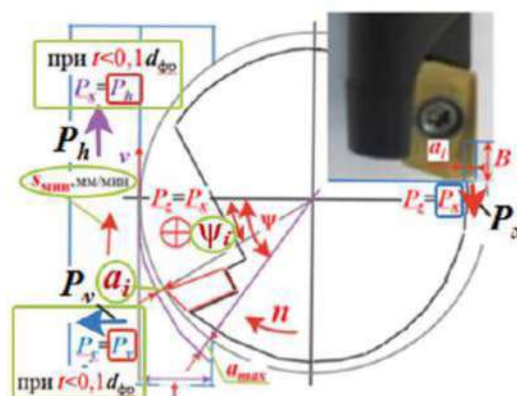
Рис. 2. Схема направления составляющих P_h , P_v и P_x силы резания при попутном фрезеровании концевой фрезой с СМП
