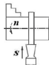
Рис. 1. Точение периферии диска с радиальной подачей резца s
