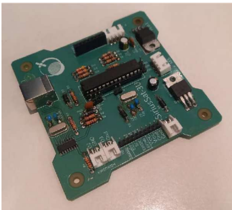
Рисунок 4 - Плата СЭП.
