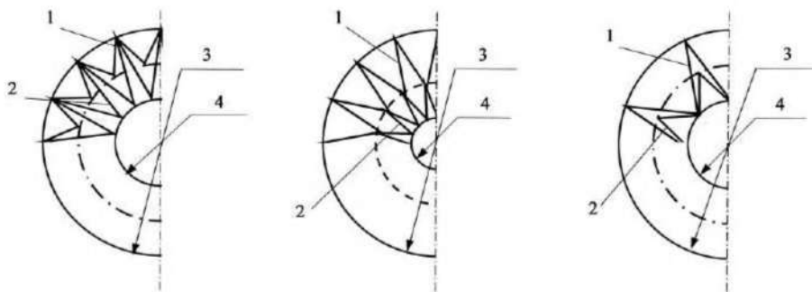
Рис. 1 Схема фильтрующего двухступенчатого элемента с звездообразной шторой:
