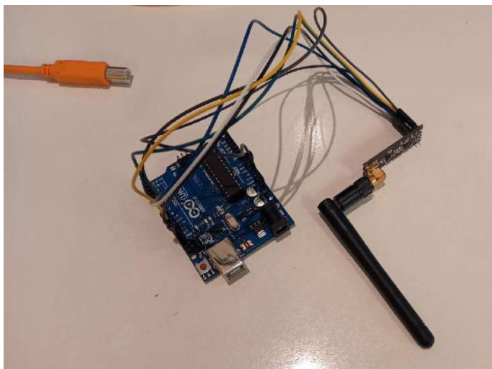
Рисунок 4 - Приёмник.
