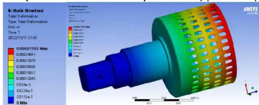
Рис. 2. Деформация сепаратора от расчетной нагрузки на валу 800 \text{ Н} \cdot \text{м}
