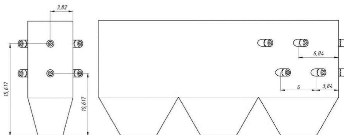
Рисунок 2 – Расположение двухпоточных вихревых горелок
