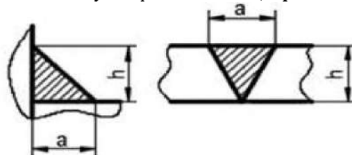
Рис. 1. Сварочный шов.
