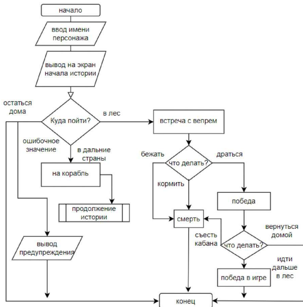
Рис. 1. Блок-схема игры
