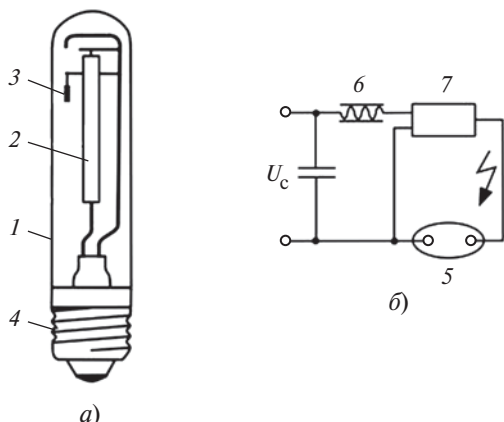
Рис. 5.6. Общий вид (а) и схема включения (б) НЛВД:
