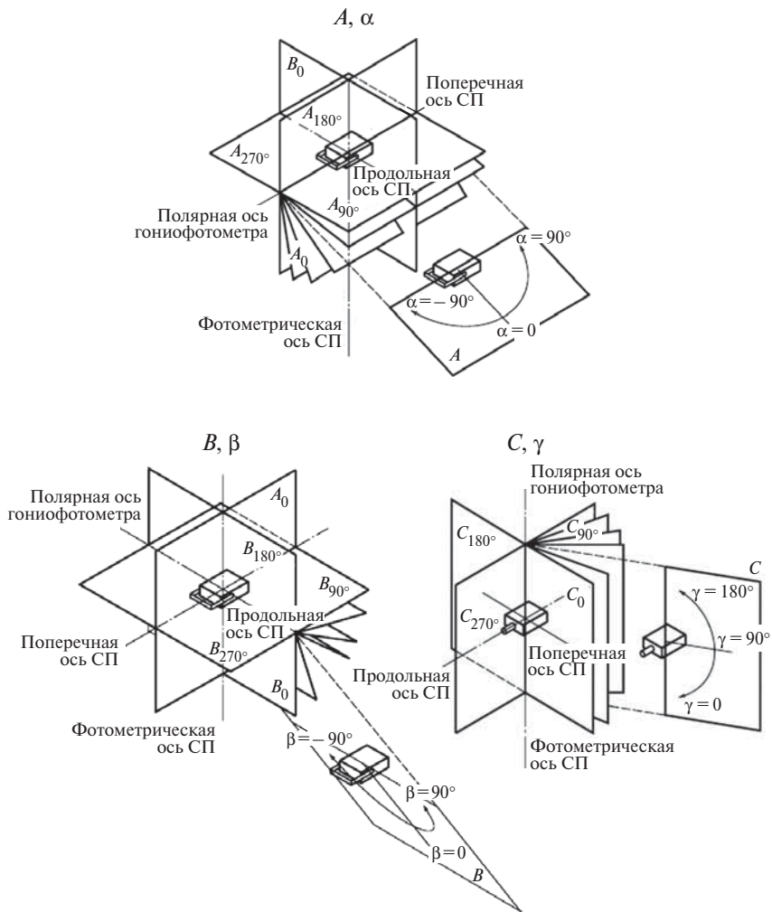
Рис. 3.1. Системы фотометрирования
