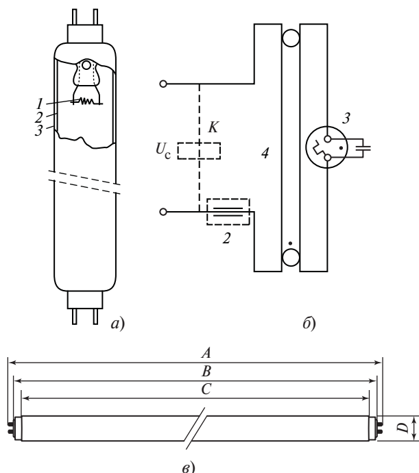
Рис. 5.3. Общий вид (а), стартерная схема подключения (б) и габаритные размеры (в) ЛЛ:
