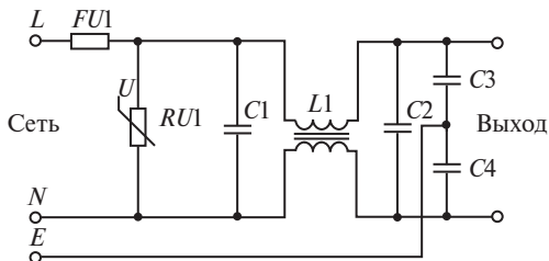
Рис. 8.5. Схема входного фильтра ИЭП
