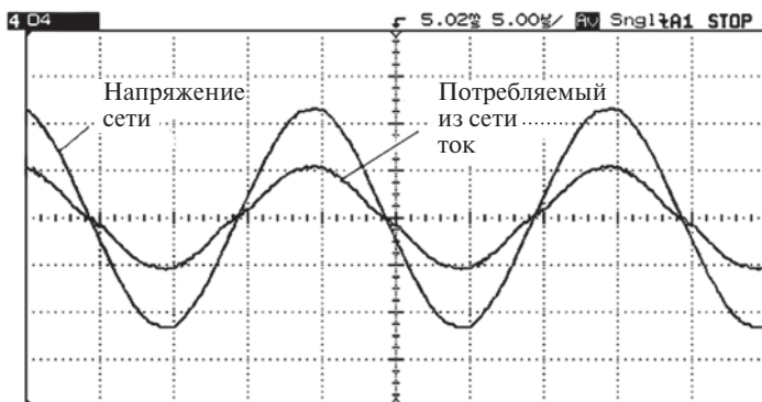
Рис. 8.9. Оциллограммы сетевого напряжения и потребляемого тока
